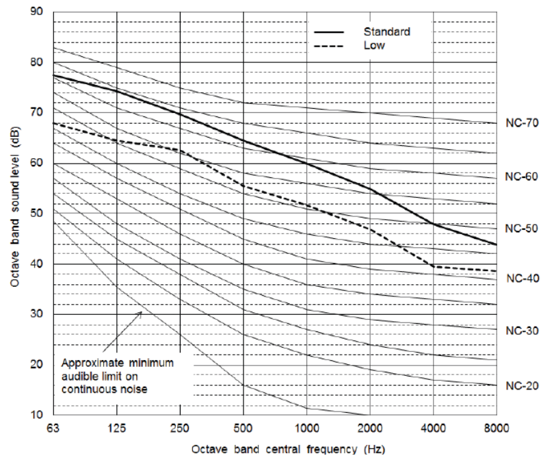
Fig. 47 —38VMA336RDS5-1
