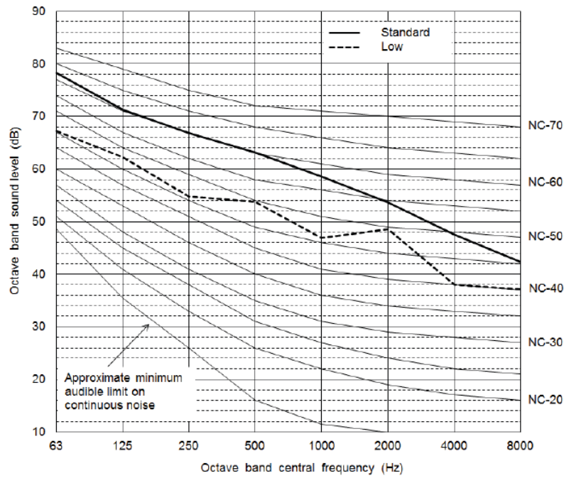
Fig. 41 —38VMA264RDS5-1
