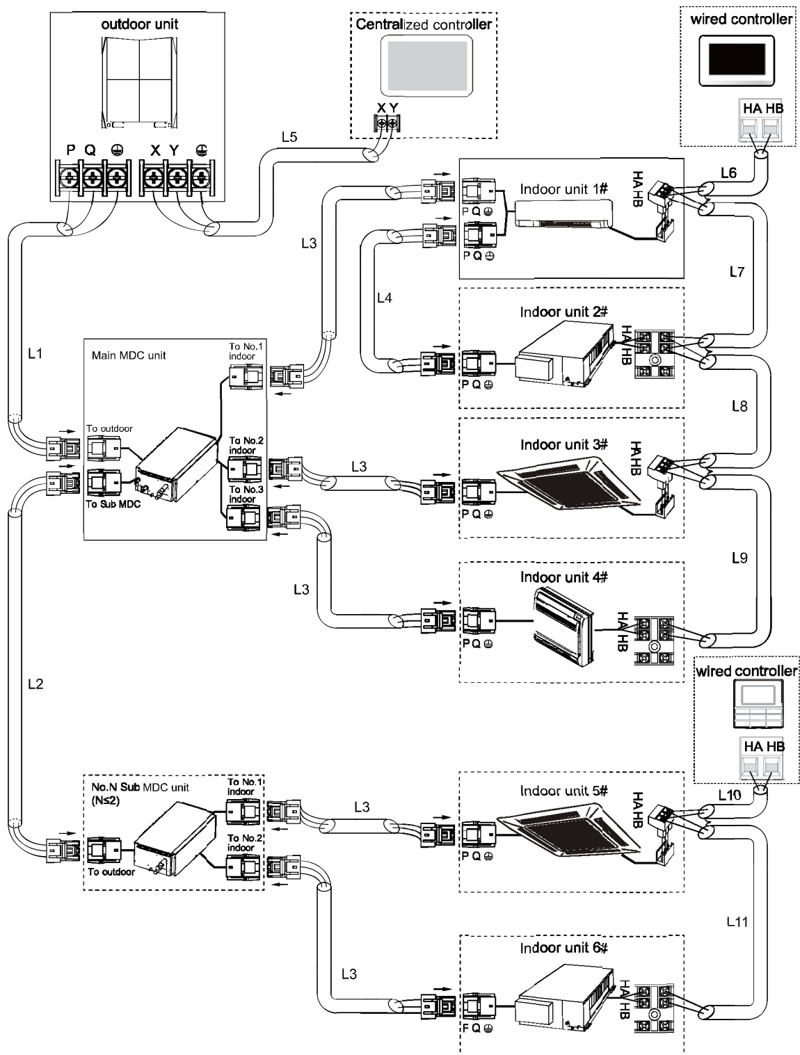
Fig. 19 —Controls Wiring
