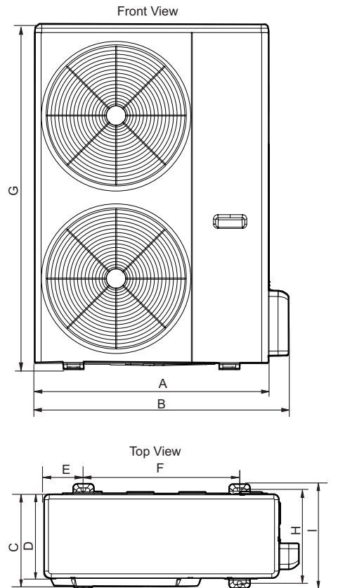
Fig. 8 —4.0 / 5.0 ton unit
