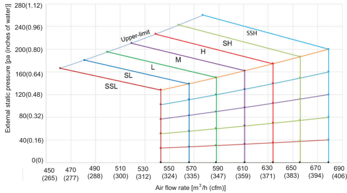
Fig. 15 —45VMV12---3
