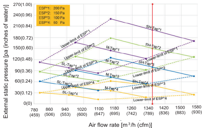
Fig. 23 —45VMV24---3
