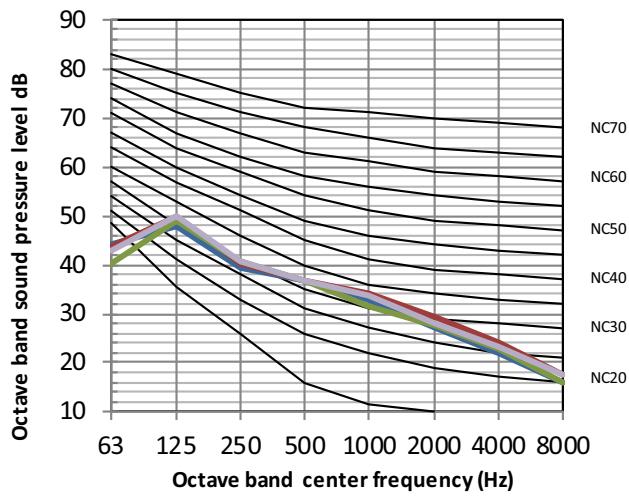
Fig. 9 —45VMV18---3
