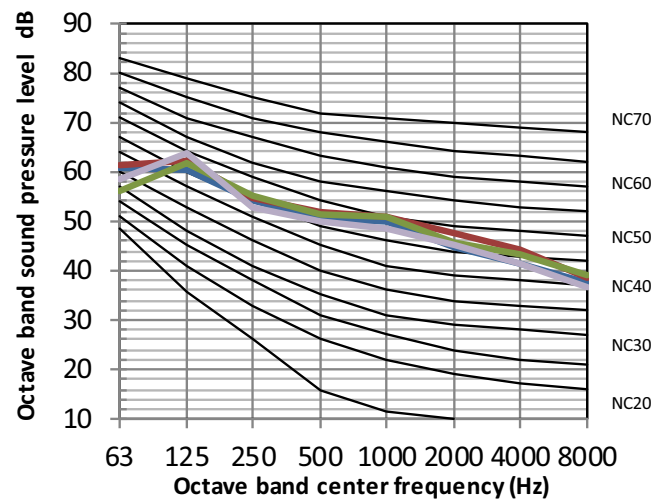
Fig. 13 —45VMV48---3
