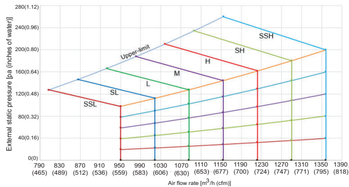
Fig. 17 —45VMV24---3
