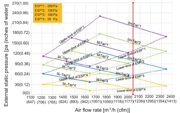
Fig. 25 —45VMV36---3
