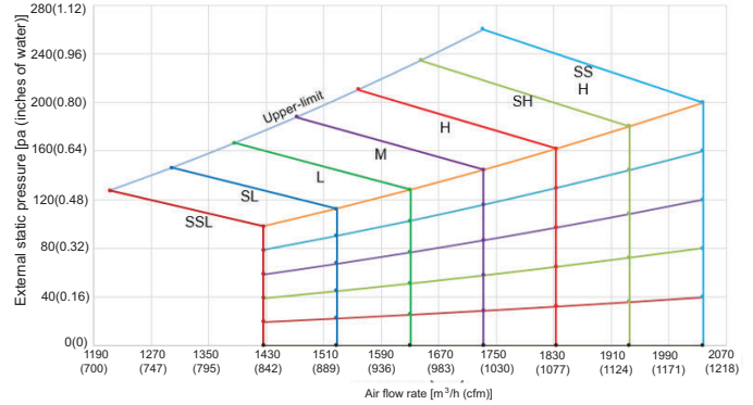
Fig. 18 —45VMV36---3
