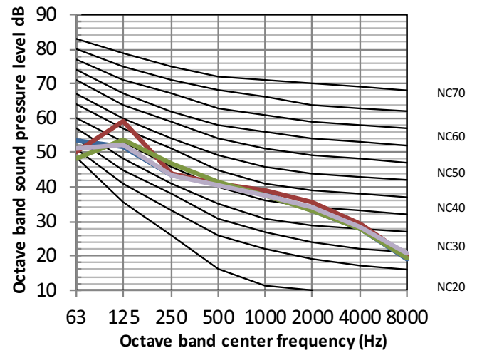
Fig. 11 —45VMV30---3
