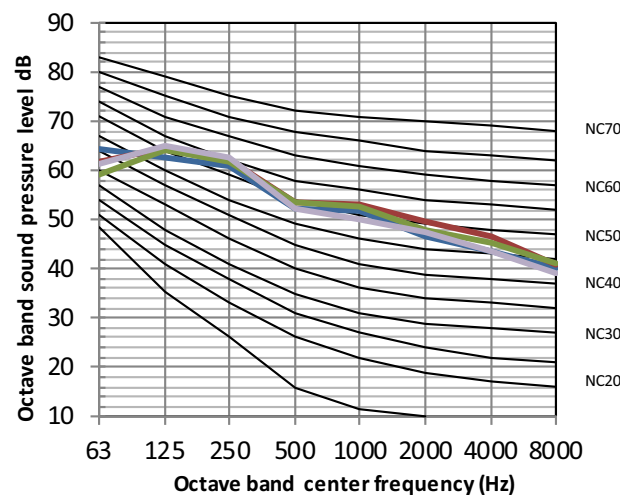
Fig. 14 —45VMV54---3
