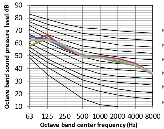
Fig. 12 —45VMV36---3
