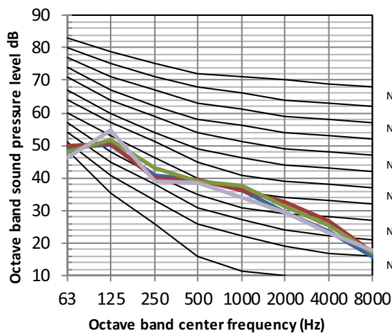
Fig. 10 —45VMV24---3
