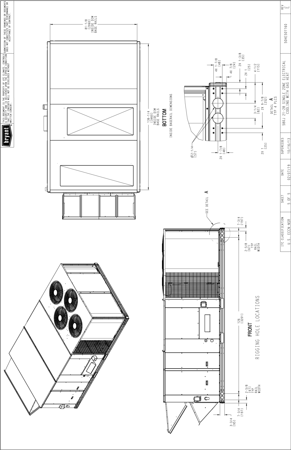
580J*21-25 BOTTOM VIEW
