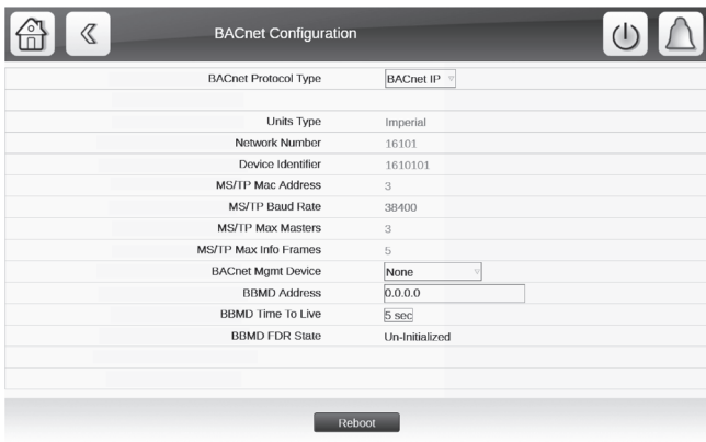
Fig. 67 — BACnet IP
