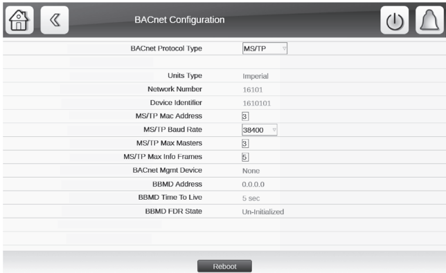
Fig. 66 — BACnet MS/TP
