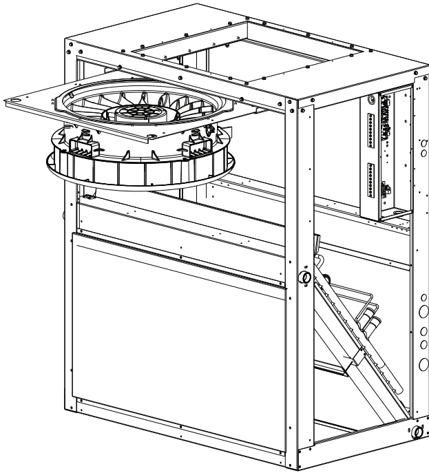
Fig. 39 — Slide Out Fan Deck Assembly
