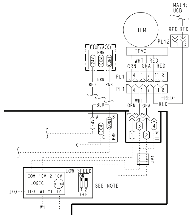
Fig. 30 — Supply Fan Control Wiring Diagram
