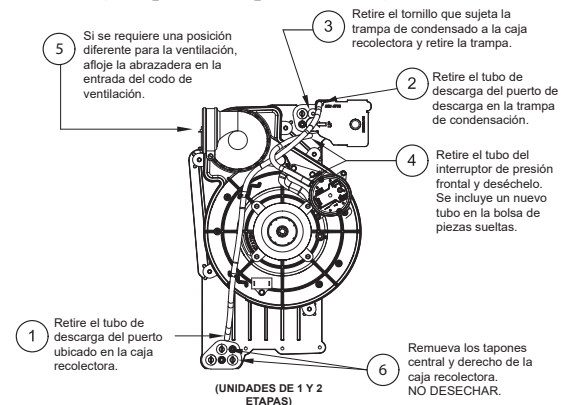
Fig. 10 – Configuración de la trampa horizontal a la derecha (La apariencia puede variar)
