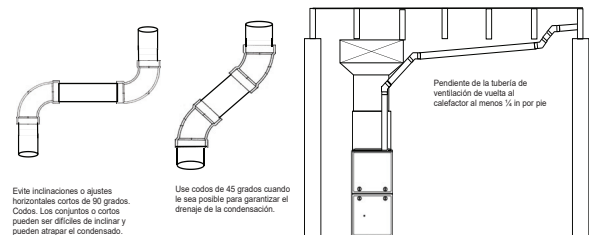
Fig. 52 – Conexiones de ventilación cerca del calefactor
