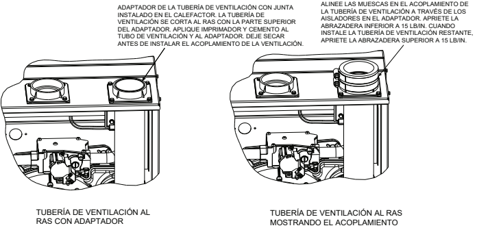
Fig. 59 – Tubería opcional de ventilación al ras con adaptador
