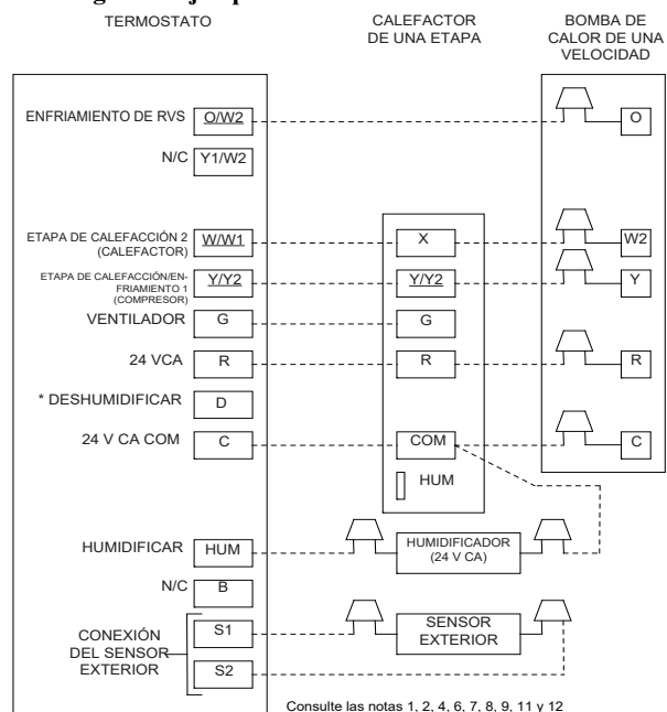
Fig. 38 – Ejemplo de control monofásico del calefactor
