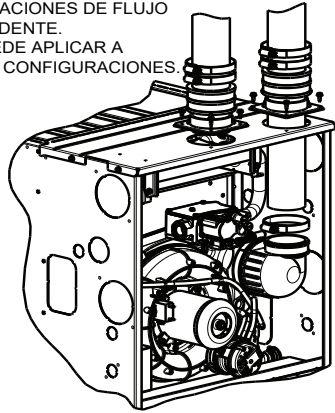
Fig. 44 – Ejemplo de conexión de la tubería de aire de admisión para sistemas de ventilación de polipropileno
