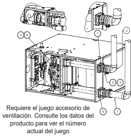
CONFIGURACIÓN DE VENTILACIÓN DERECHA HORIZONTAL A LA IZQUIERDA
