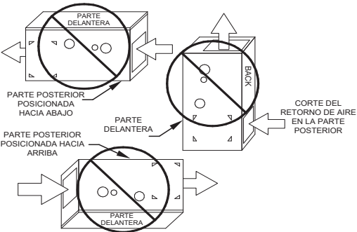
Fig. 4 – Instalaciones prohibidas
