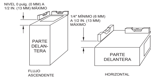
Fig. 19 – Requisitos de inclinación del calefactor
