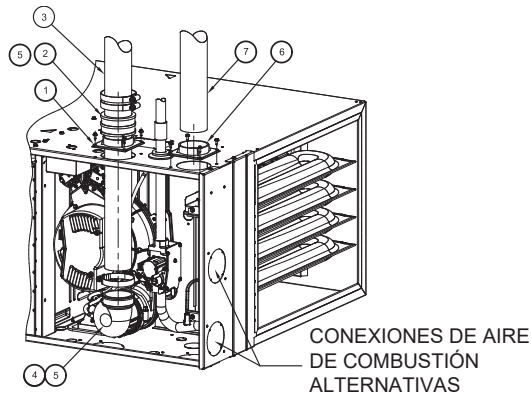
CONFIGURACIÓN DE VENTILACIÓN VERTICAL HORIZONTAL A LA DERECHA
