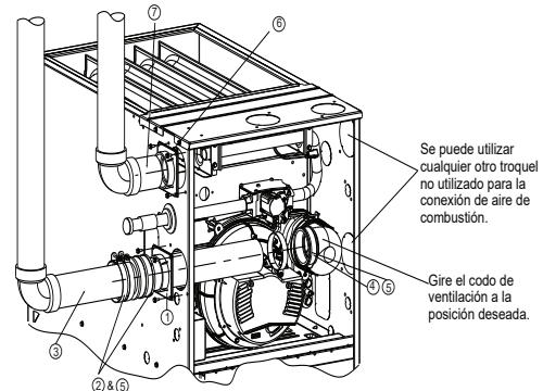
Fig. 53 – Codo de ventilación del inductor
