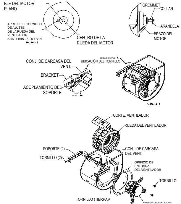
Fig. 65 – Conjunto del ventilador en 30040E14 y 36060E14
