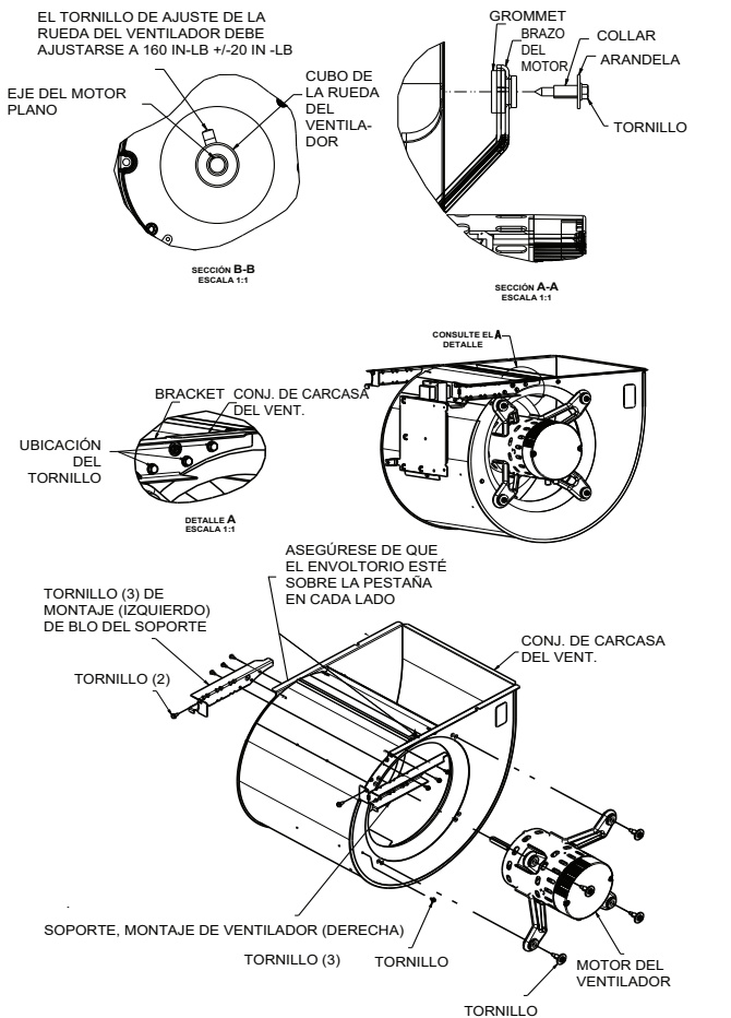
Fig. 66 – Conjunto de ventilador en 66100E21
