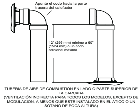
Fig. 45 – Accesorio de tubería de aire de combustión
