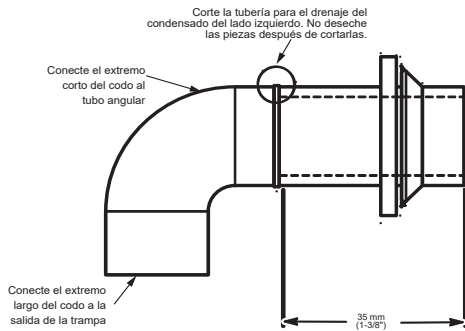
Fig. 17 – Modificación del codo de goma de drenaje
