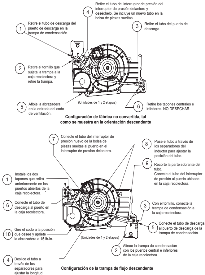
Fig. 9 – Configuración de la trampa de flujo descendente (La apariencia puede variar)
