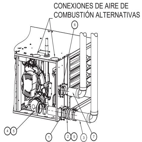
CONFIGURACIÓN DE VENTILACIÓN DERECHA HORIZONTAL A LA DERECHA
