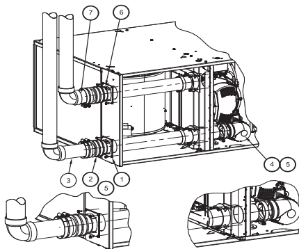
CONFIGURACIÓN DE VENTILACIÓN VERTICAL HORIZONTAL A LA DERECHA
