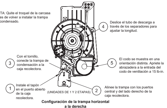
Fig. 10 – Configuración de la trampa horizontal a la derecha (La apariencia puede variar)
