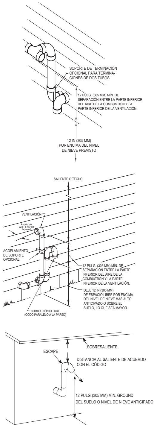
Fig. 49 – Terminación de ventilación en Alberta y Saskatchewan Tamaño de las tuberías de ventilación y aire de combustión
