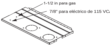
Fig. 31 – Entrada de gas y electricidad alternativa
