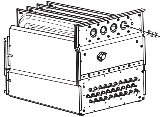
Fig. 70 – Limpieza de la celda del intercambiador de calor A11273SP
