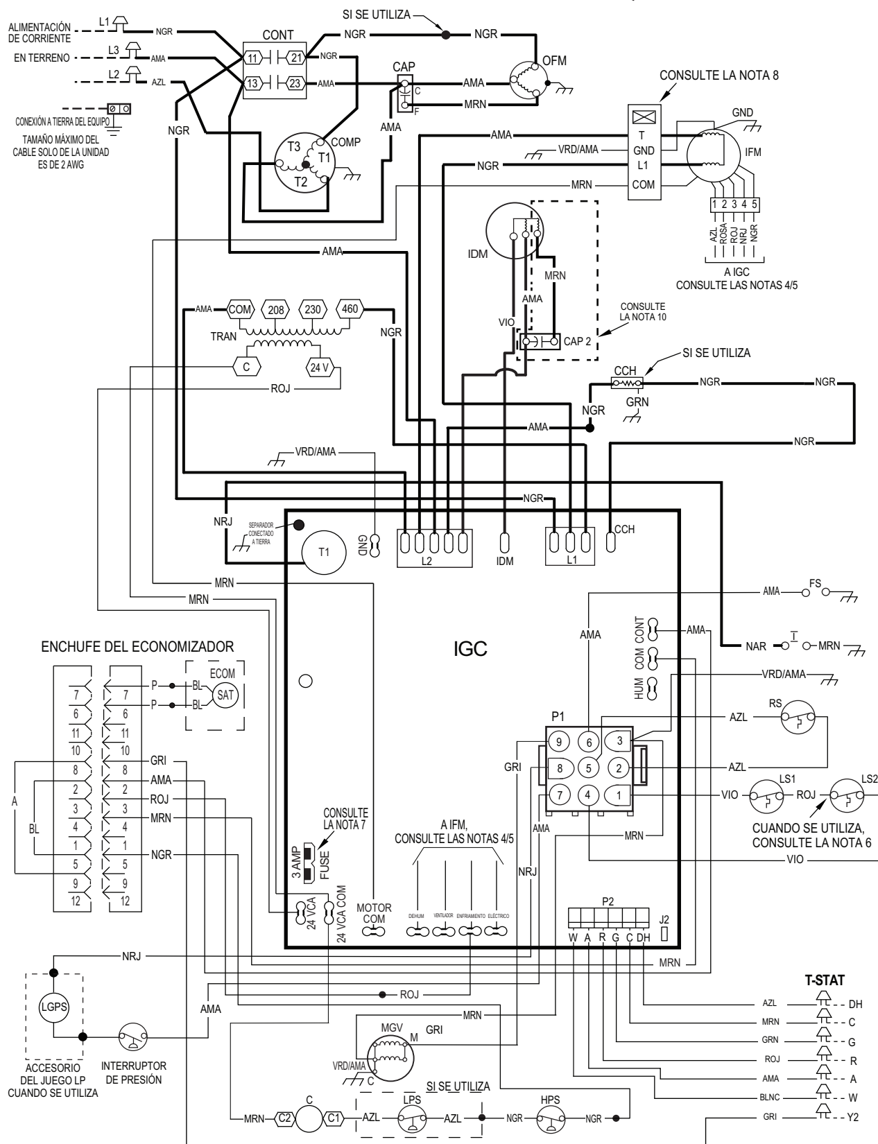
Fig. 18 – Diagrama eléctrico de conexión 460-3-60
