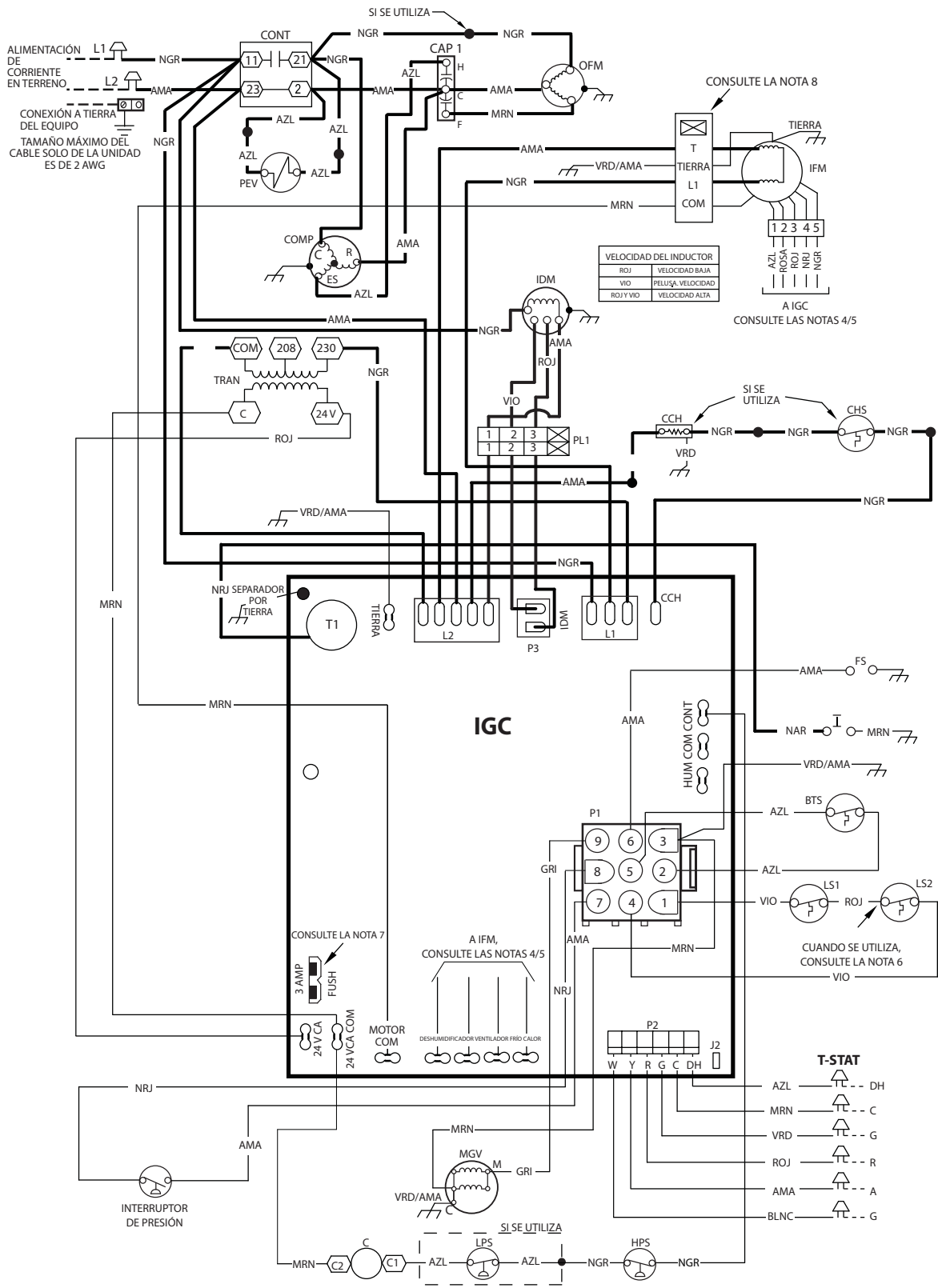
Fig. 15 – Diagrama eléctrico de conexión con NOx ultrabaja de 208/230-1-60
