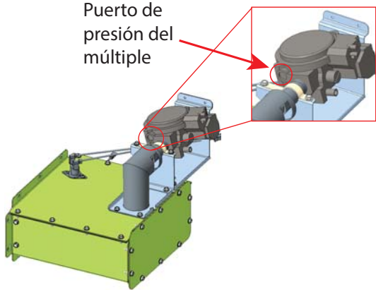
Fig. 12 – Conjunto de colector de gas y caja del quemador
