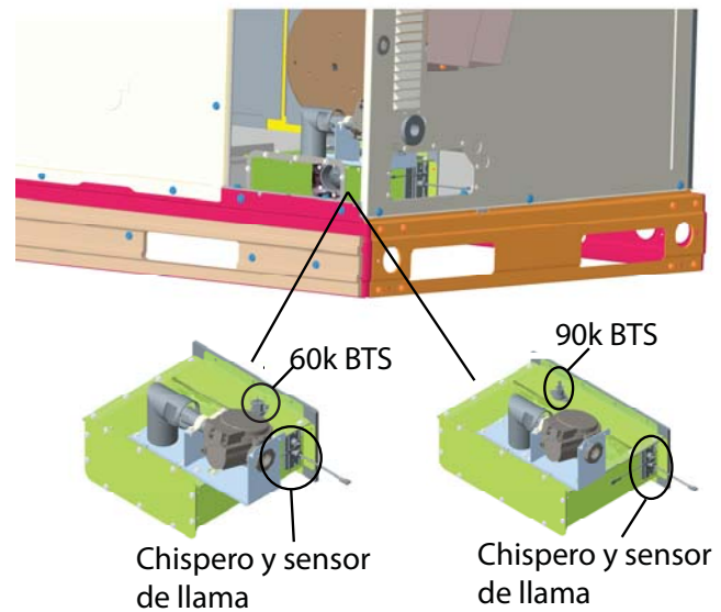
Fig. 20 – Interruptor térmico del quemador (BTS) (NOx ultrabajo)
