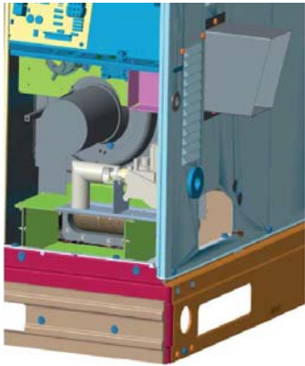
Fig. 11 – Conjunto del quemador
