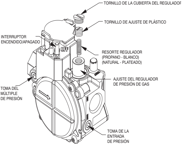
Fig. 13 – Válvula de gas estándar de una etapa
