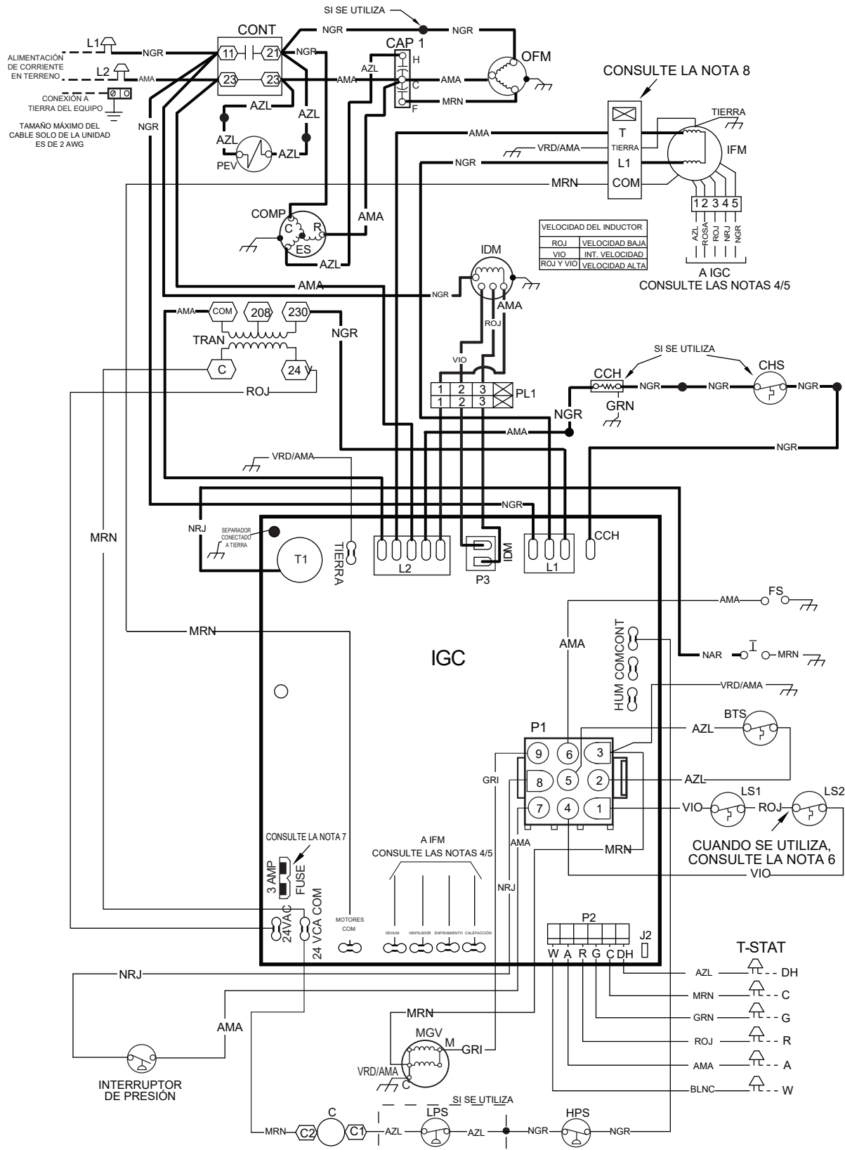
Fig. 15 – Diagrama eléctrico de conexión con NOx ultrabajo de 208/230-1-60
