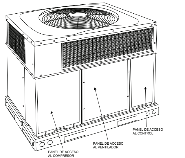
Fig. 22 – Paneles de acceso de la unidad
