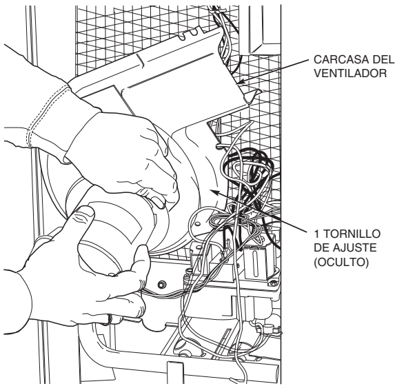
Fig. 23 – Extracción del motor y la rueda del ventilador
