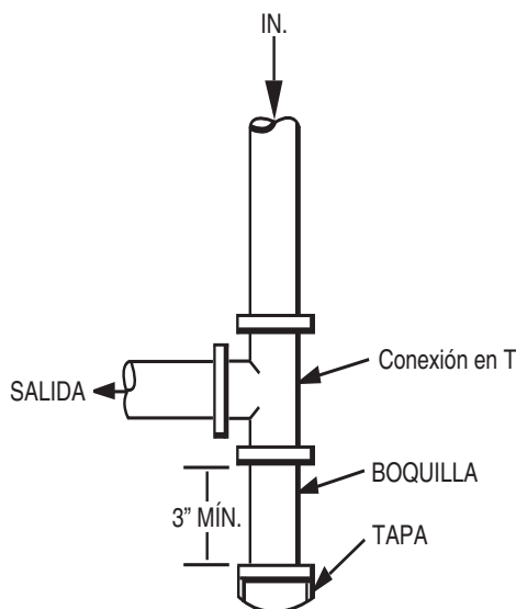
Fig. 8 – Trampa de sedimentos
