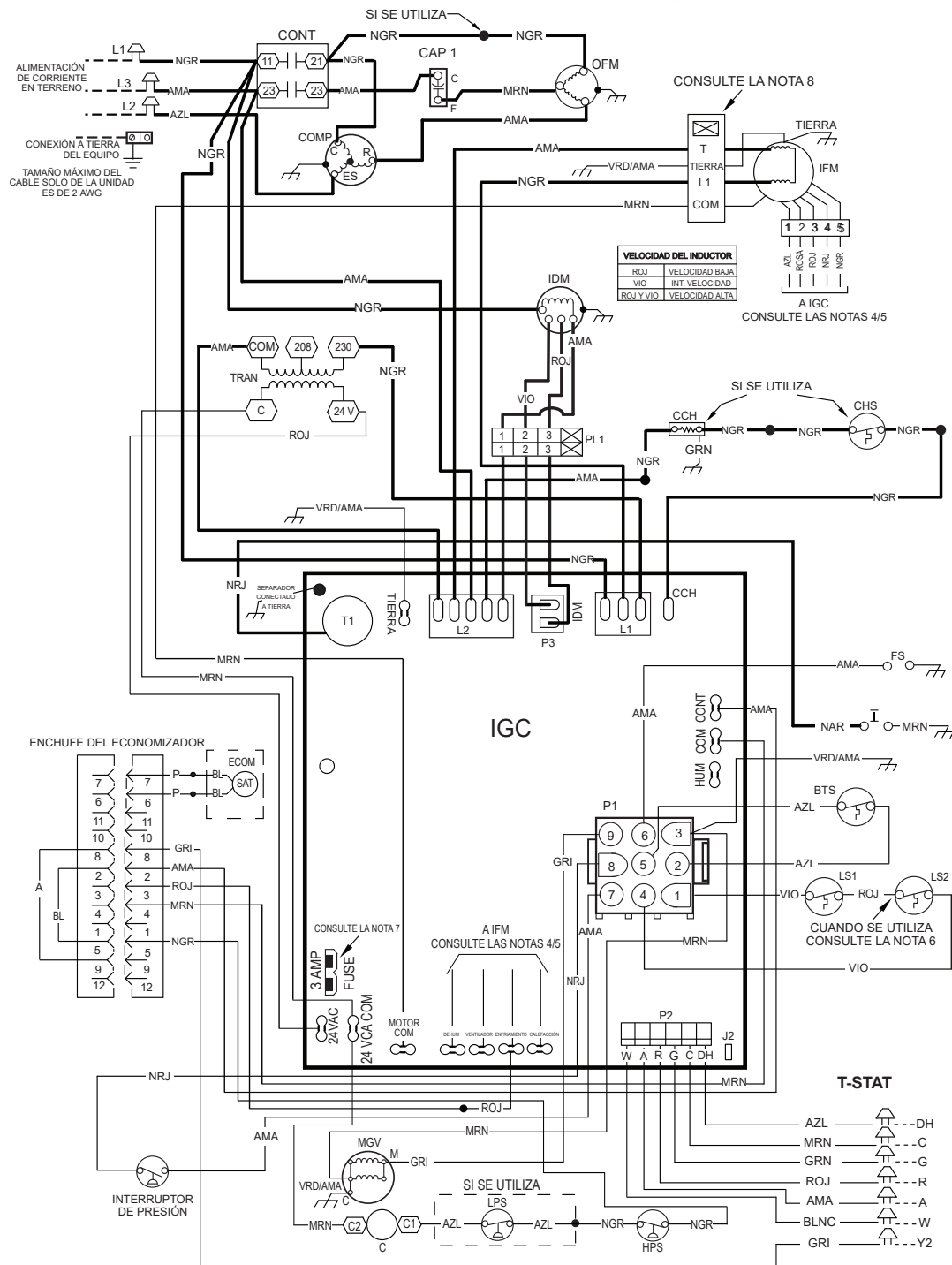
Fig. 17 – Diagrama eléctrico de conexión con NOx ultrabajo de 208/230-3-60
