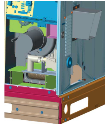
Fig. 11 – Conjunto del quemador
