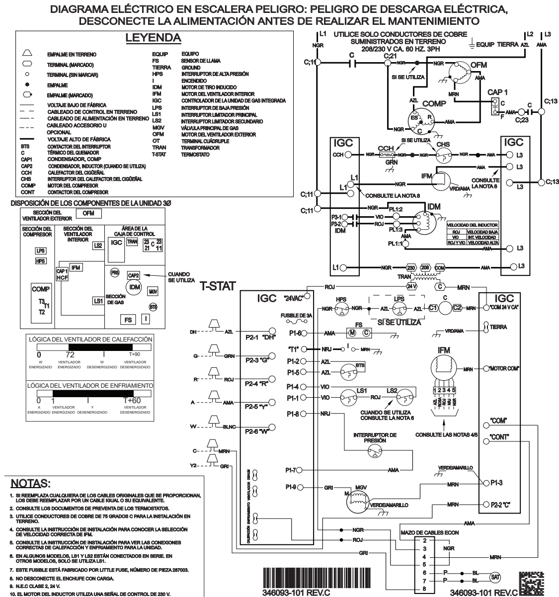
Fig. 18 – Diagrama eléctrico en escalera con NOx ultrabajo de 208/230-3-60, tamaño 30
