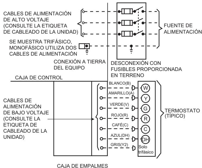
Fig. 10 – Conexiones de alto voltaje y de control de voltaje
