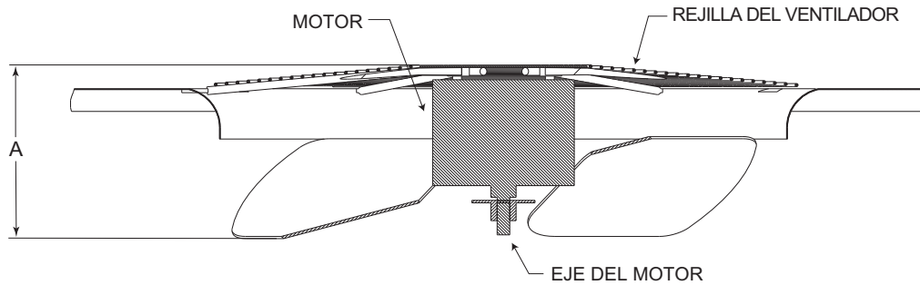
Fig. 23 – Extracción del motor y la rueda del ventilador
