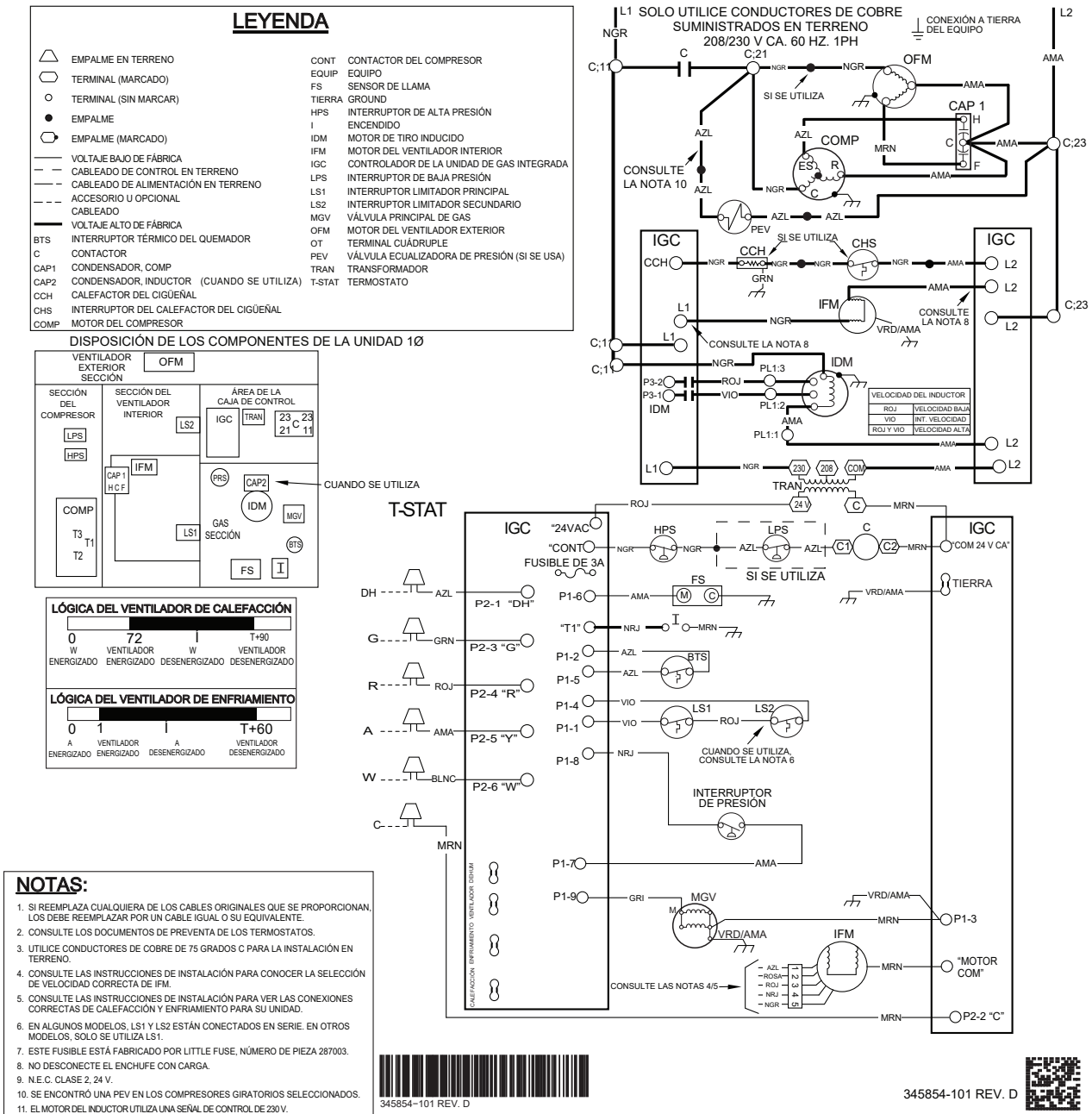
Fig. 16 – Diagrama eléctrico en escalera con NOx ultrabajo de 208/230-1-60, tamaño 30
