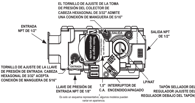
Fig. 13 – Válvula de gas estándar de una etapa
