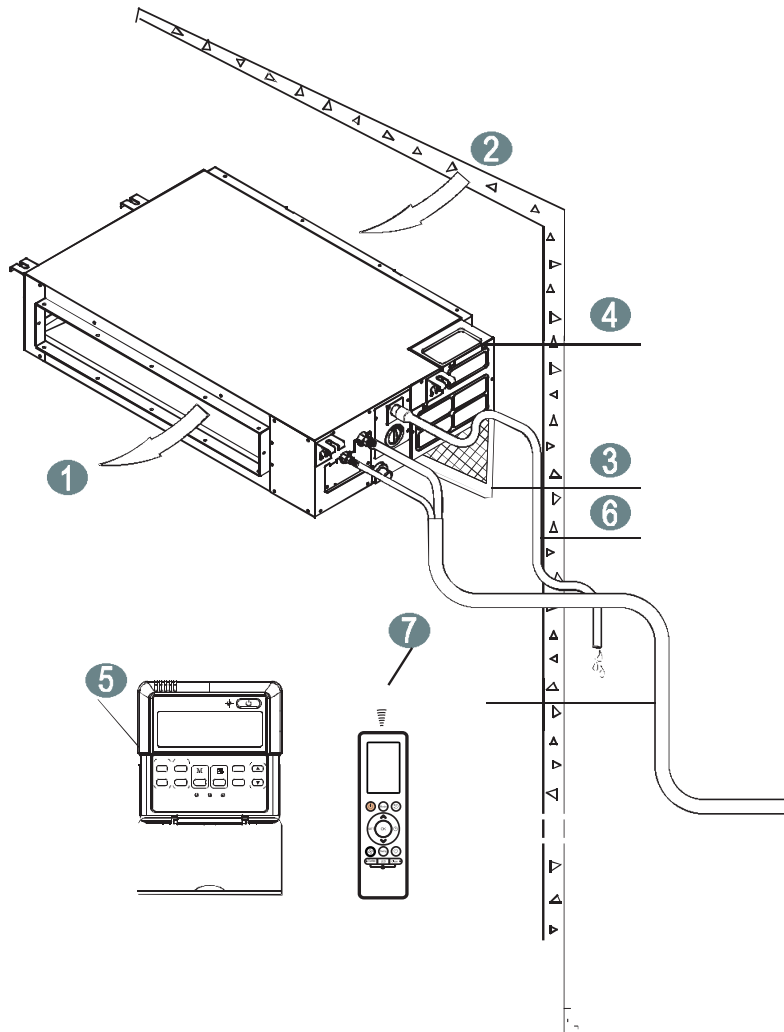
Fig. 1 — Indoor Unit
