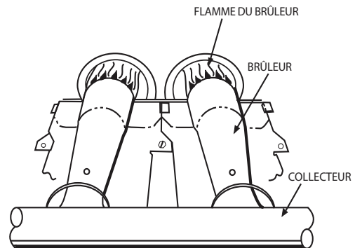
Figure 10 – Brûleur monoport
