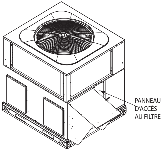
Figure 8 – Accès au filtre à petit châssis
