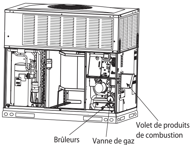
Figure 3 – Appareil de chauffage au gaz et de climatisation électrique avec panneau d'accès retiré A14490FR
