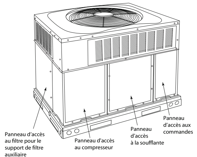
Figure 2 – Panneaux d'accès de l'appareil
