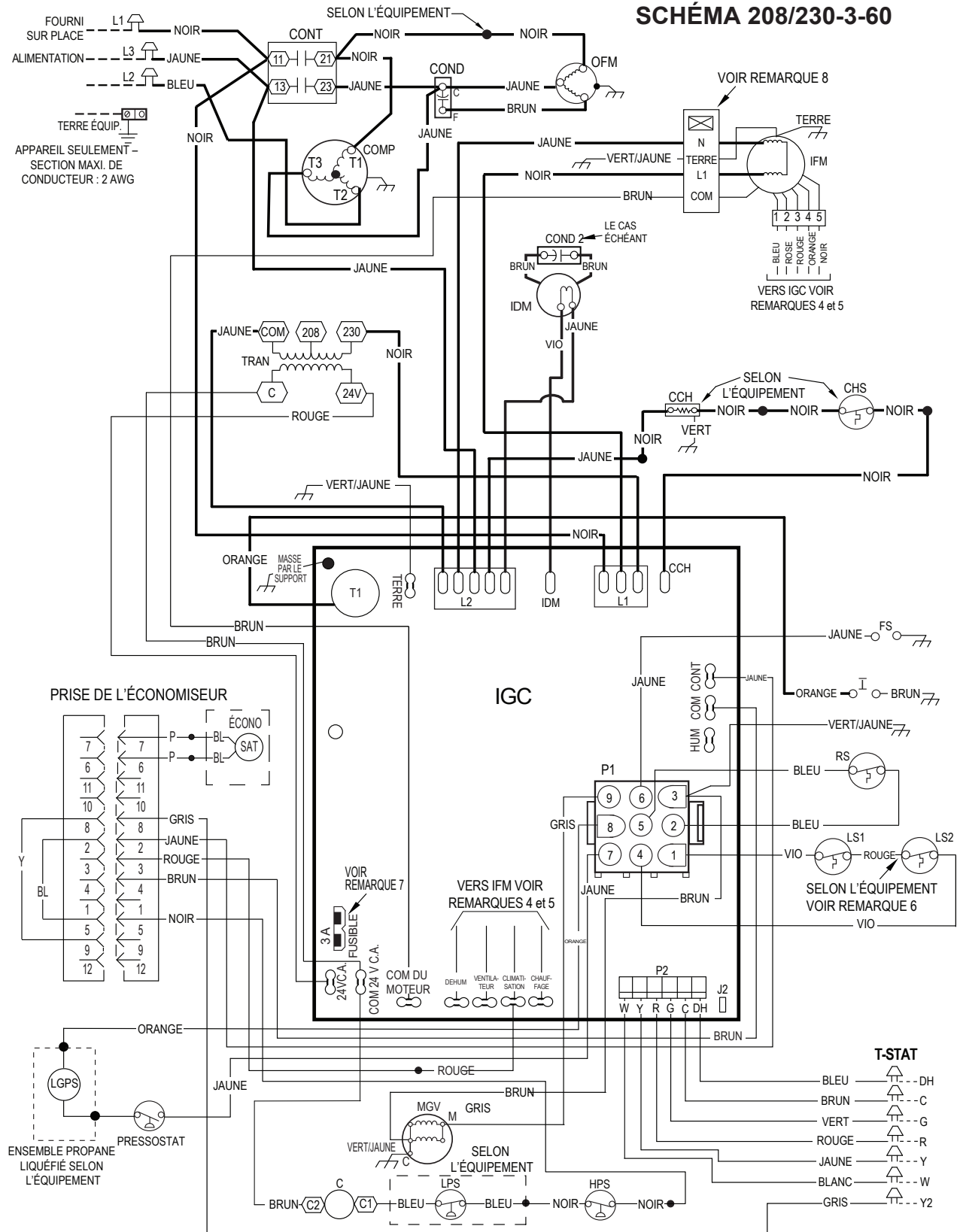
Fig.16 – Schéma de connexion de câblage – 208/230-3-60
