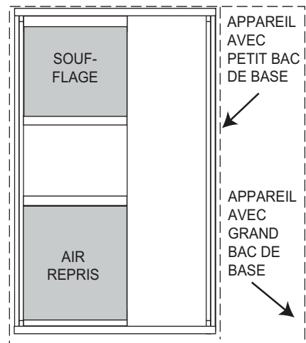
POSE DE L'APPAREIL SUR UN CADRE COMMUN
