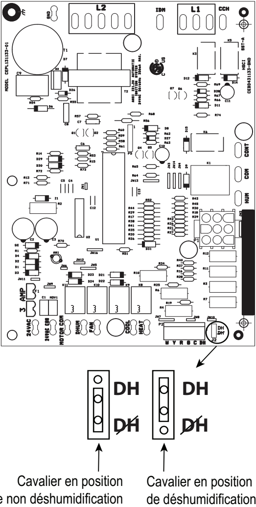
Fig. 20 – Carte de l'IGC
