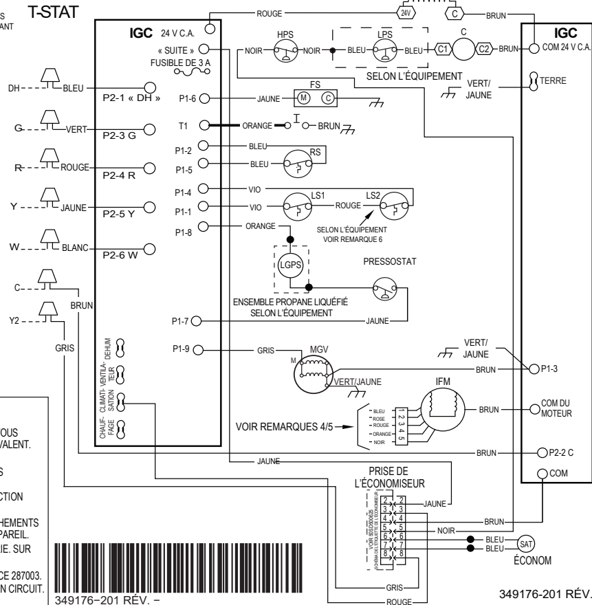
Fig.17 – Schéma de câblage en échelle – 208/230-3-60
