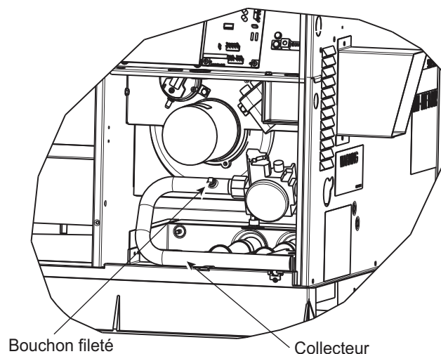
Fig. 11 – Ensemble du brûleur
