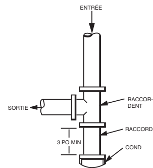
Fig. 8 – Piège à sédiments
