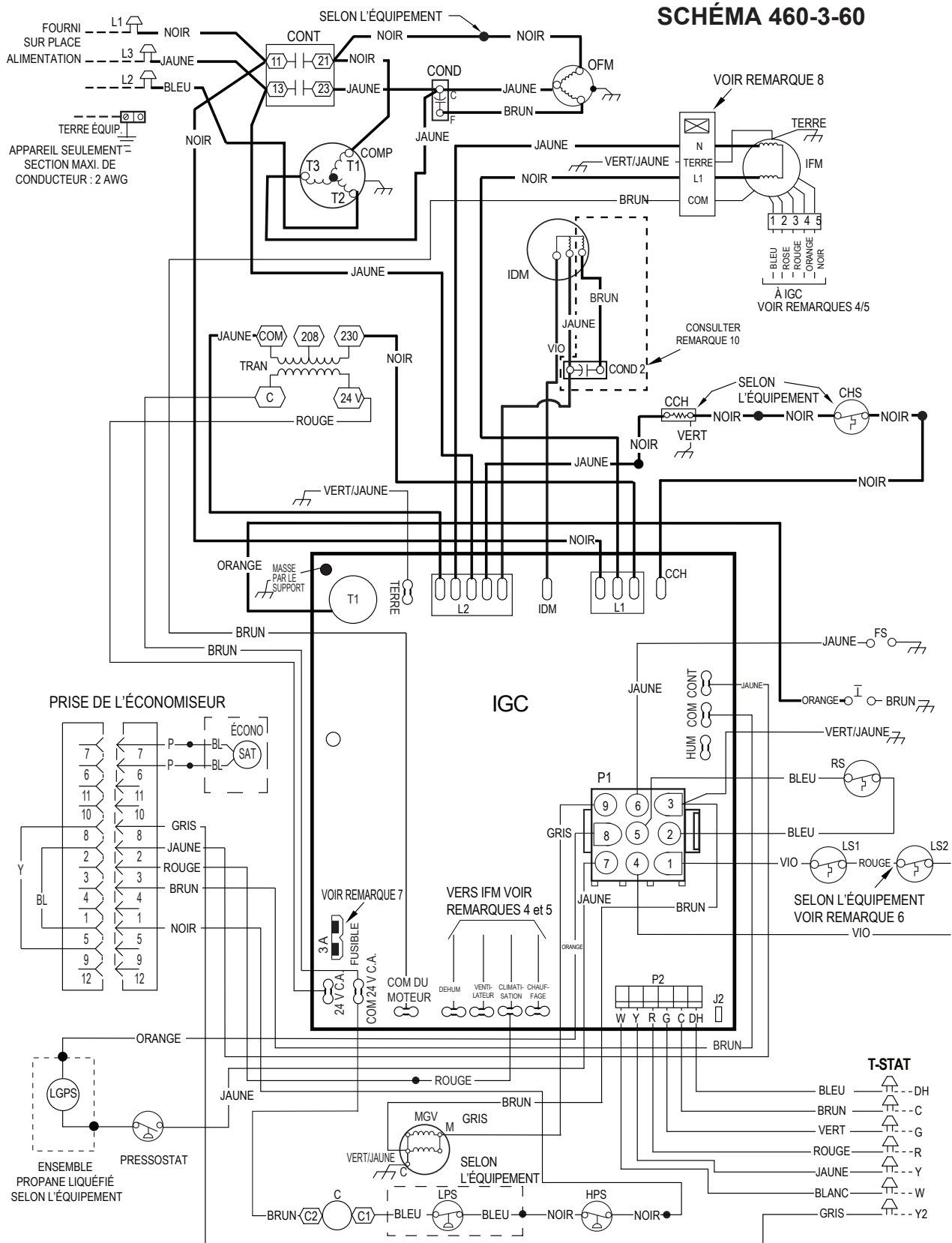
Fig.18 – Schéma de connexion de câblage – 460-3-60
