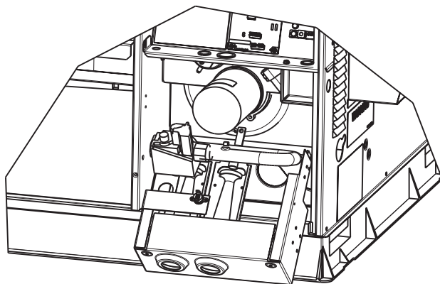
Fig. 24 – Porte-brûleur déposé
