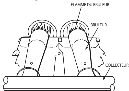
Fig. 12 – Brûleur monoport
