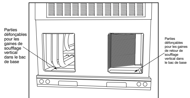
Fig. 9 – Ouvertures d'air de soufflage et de retour
