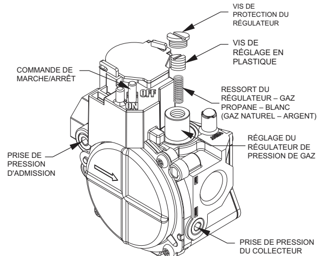
Fig. 13 – Vanne de gaz à une phase
