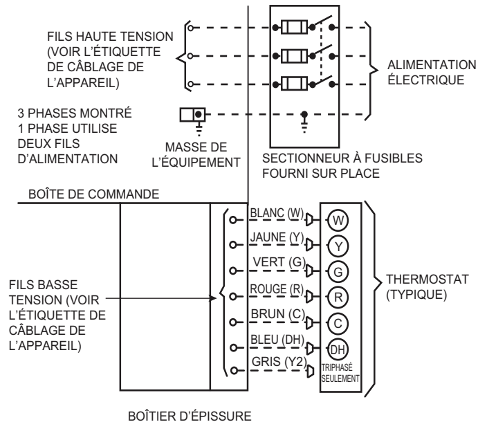
Fig. 10 – Branchements haute et basse tensions
