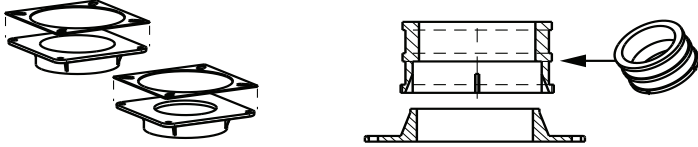
Fig. 47 – Adaptador y acoplamiento de ventilación con juntas
