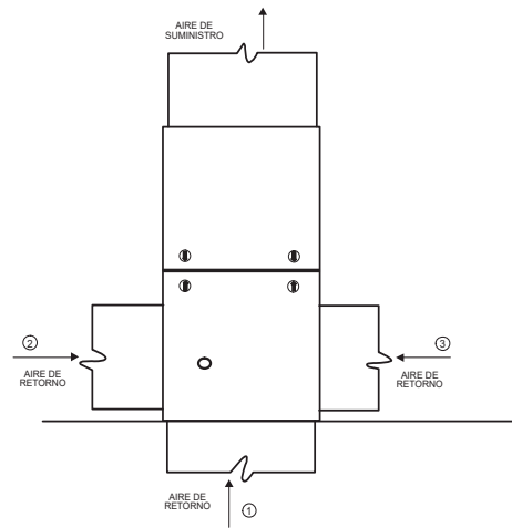
Fig. 28 – Configuraciones y restricciones de aire de retorno de flujo ascendente
