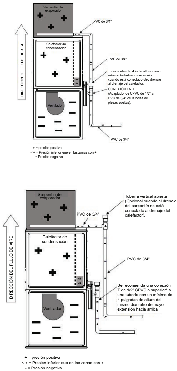
Fig. 10 – Ejemplo de conexión del drenaje in situ (no permitido)
