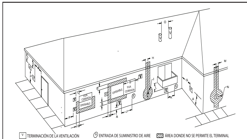
Fig. 55 – Distancias para las terminaciones de ventilación de aire de combustión ventilado y de ventilación indirecta
