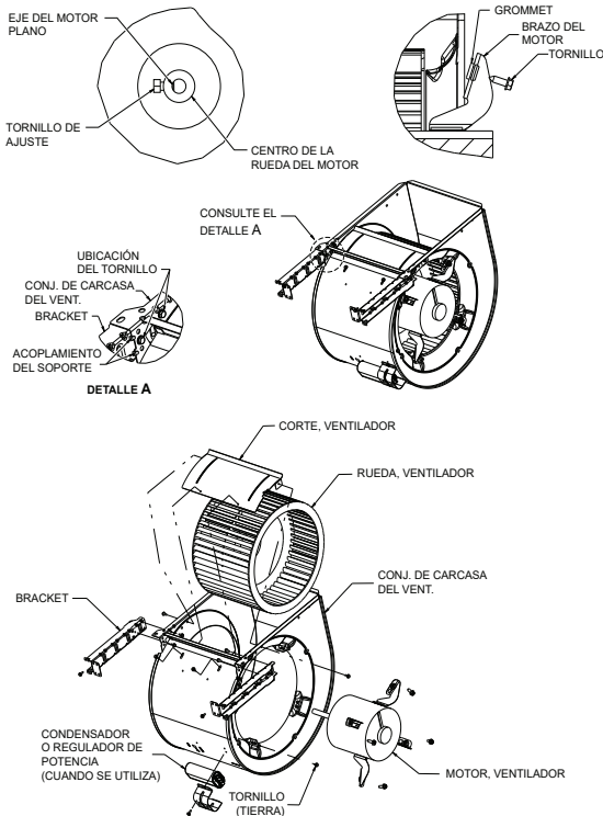
Fig. 65 – Conjunto de ventilador en 100E21-22
