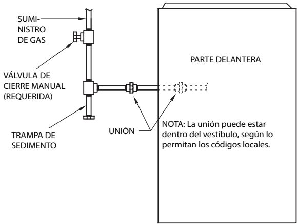
Fig. 37 – Disposición típica de las tuberías de gas
