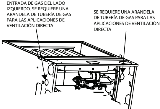
Fig. 35 – Entrada de gas
