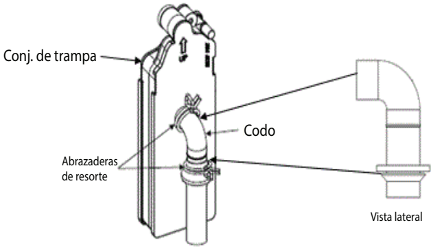
Fig. 24 – Conexión del drenaje de condensación Instalación de los serpentines del evaporador
