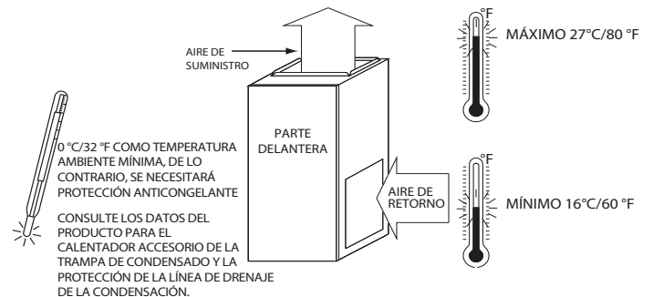
Fig. 3 – Protección anticongelante y temperatura del aire de retorno
