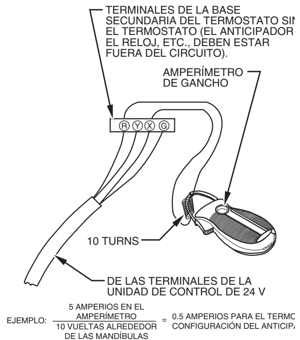
Fig. 62 – Verificación del consumo en amperios con un amperímetro
