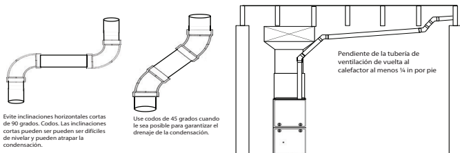
Fig. 46 – Conexiones de ventilación cerca del calefactor
