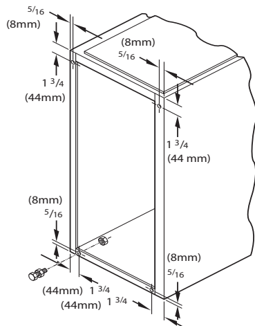
Fig. 30 – Patas niveladoras
