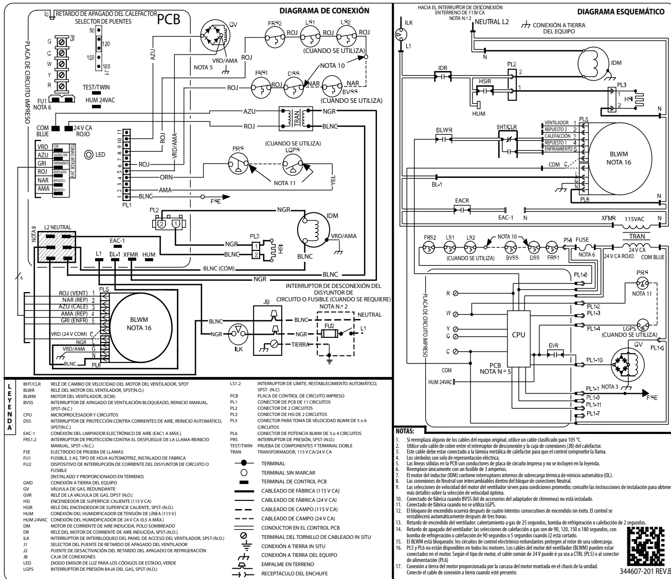
Fig. 50 – Diagrama eléctrico
