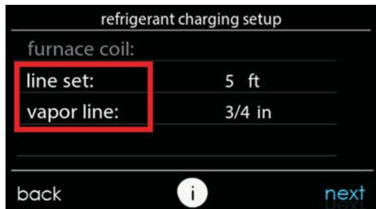
Fig. 17 – Sélection de la longueur de la conduite et du diamètre de la A200035 conduite de vapeur
