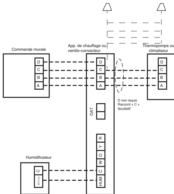
Fig. 5 – Câblage de chaudière ou de ventilateur-convecteur Infinity avec thermopompe communicante à vitesse variable Étape 7 – Raccordement des conduites
