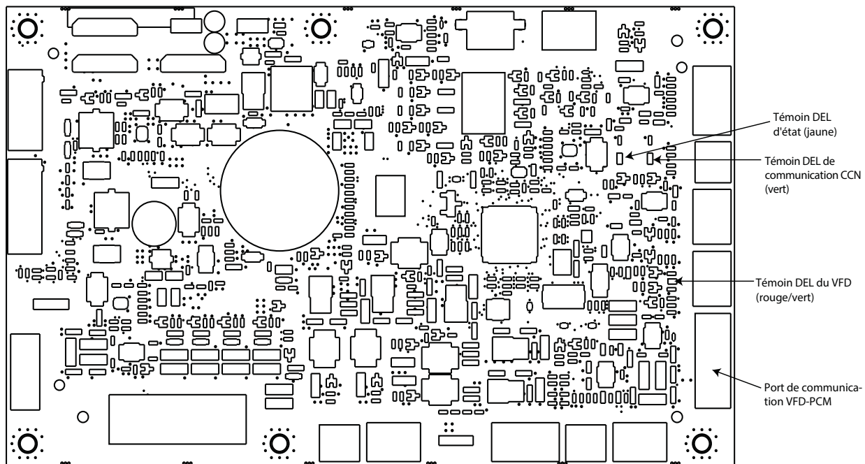
Fig. 27 – Panneau de commande du registre
