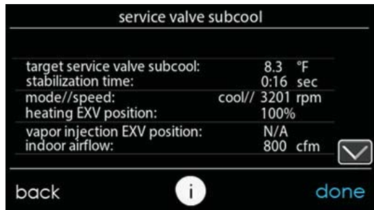
Fig. 14 – Vanne de service de liquide – Sous-refroidissement cible A200032
