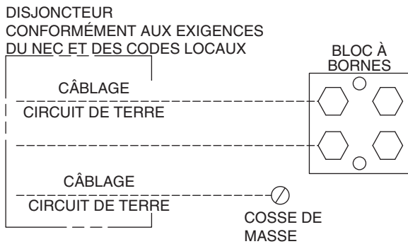
Fig. 9 – Branchements de l'alimentation secteur
