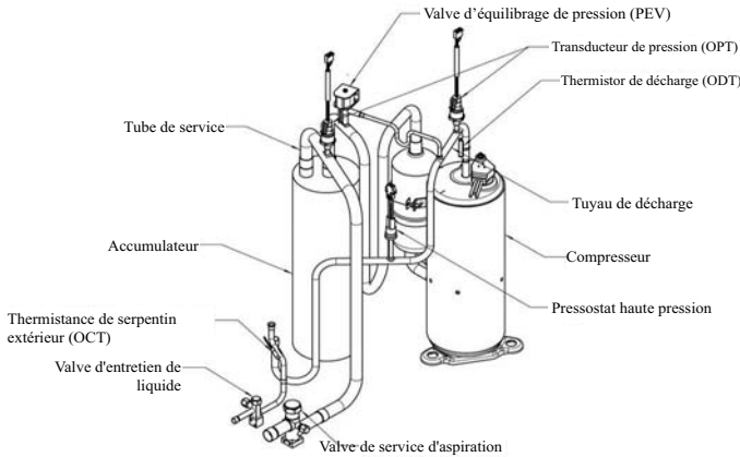
Fig. 30 – Emplacements de montage du thermistor de décharge (ODT)
