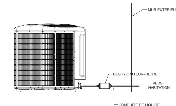
Fig. 6 – Déshydrateur-filtre de conduite de liquide pour capacités de 2, 3 et 4 tonnes
