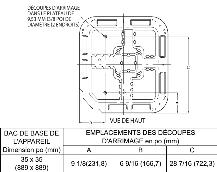
Fig. 3 – Emplacements des découpes d'arrimage
