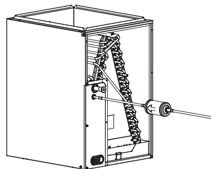
Fig. 6 – Déshydrateur-filtre de conduite de liquide pour capacités de 2, 3 et 4 tonnes
