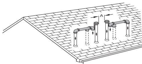
Fig. 48 – Sortie d'évacuation et de combustion
