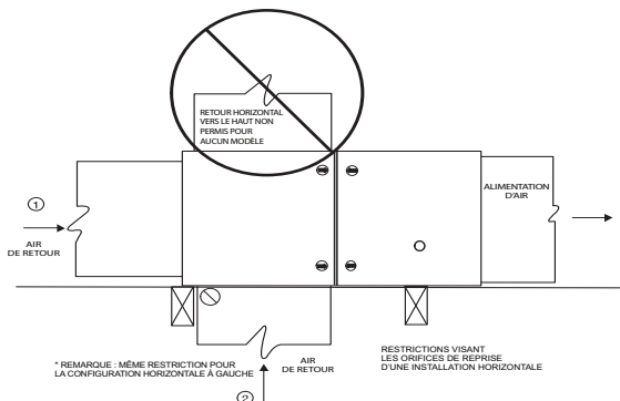
Fig. 23 – Configurations et restrictions des conduits de retour d'air horizontal and Restrictions
