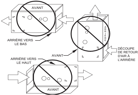
Fig. 4 – Installations prohibées
