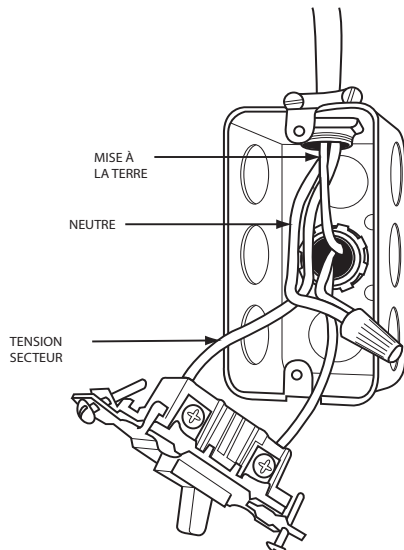
Fig. 36 – Coffret électrique externe
