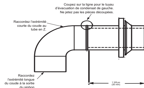
Fig.16 – Modification du coude d'évacuation en caoutchouc A190401FR
