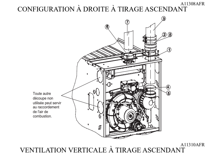
Fig. 53 – Configurations de siphon à tirage ascendant (l'apparence peut varier) Consultez les « Remarques concernant les options de ventilation ».
