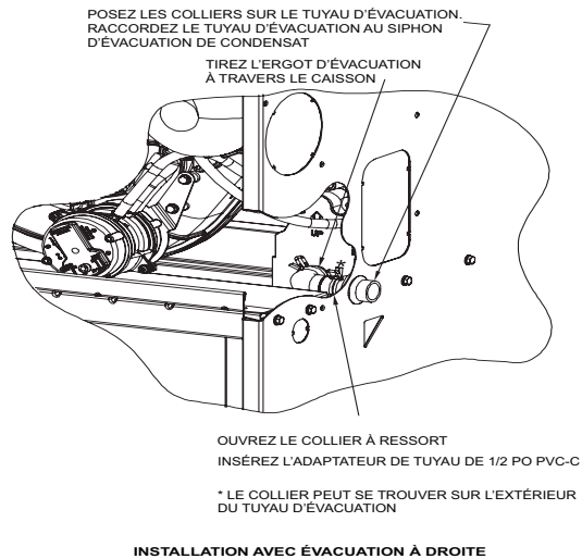
Fig.14 – Œillet d'évacuation de condensat formé en caoutchouc A11342AFR
