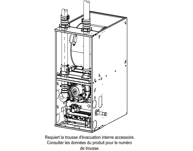
Fig. 54 – Configurations à tirage descendant (l'apparence peut varier) Consultez les « Remarques concernant les options de ventilation ».
