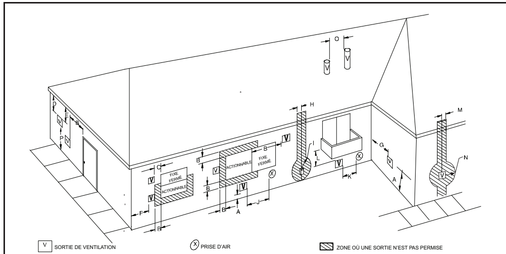
Fig. 44 – Dégagement des sorties des systèmes à air de combustion ventilé et à ventilation indirecte
