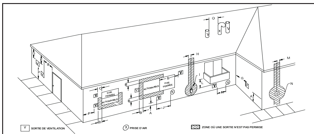
Fig. 43 – Dégagement de sortie à ventilation directe
