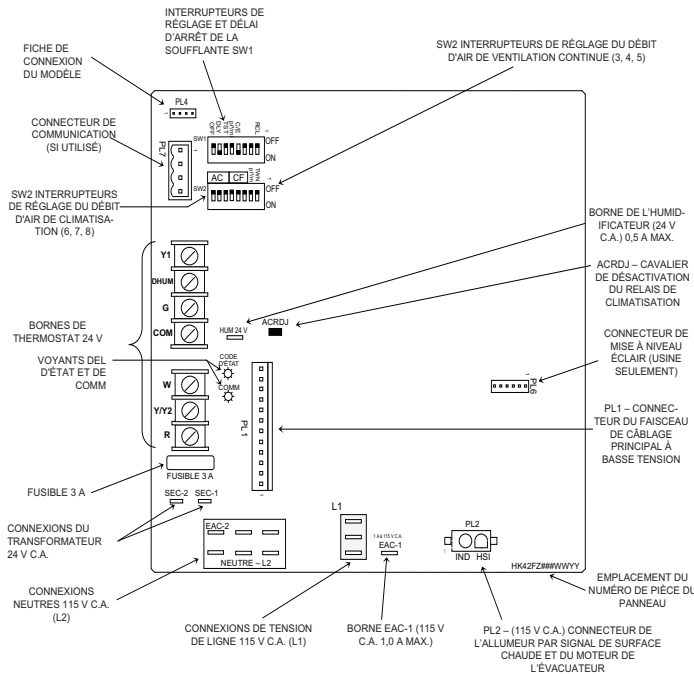
Fig. 39 – Exemple de panneau de commande de chaudière à une phase
