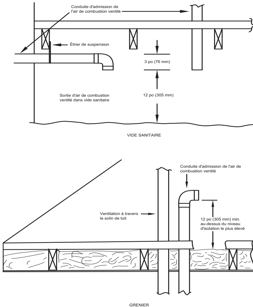
Fig. 51 – Sorties de ventilation pour système à air de combustion ventilé
