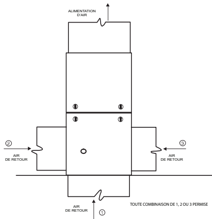
Fig. 21 – Configurations et restrictions des conduits de retour d'air ascendant
