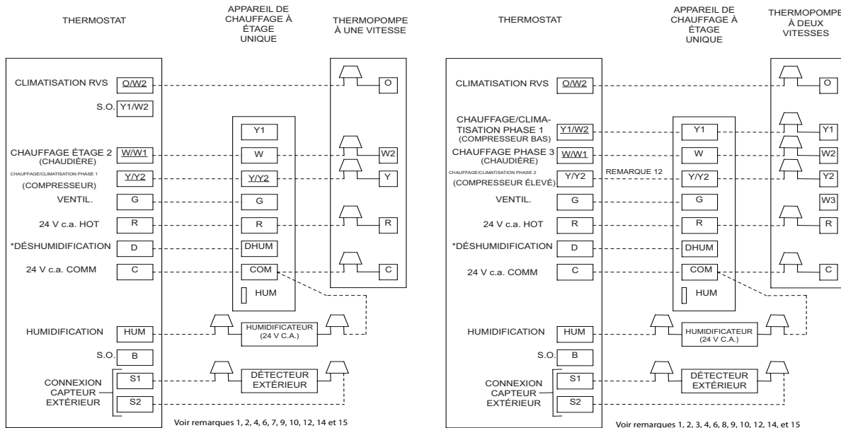
Chaudière à une phase avec thermopompe à une phase
