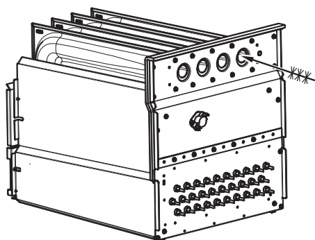
Fig. 71 – Nettoyage de la cellule de l'échangeur thermique
