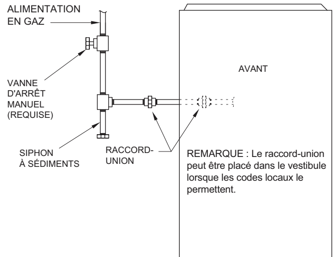
Fig. 32 – Disposition type de la tuyauterie de gaz
