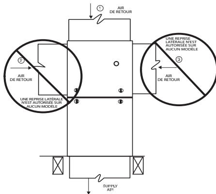
Fig. 22 – Configurations et restrictions des conduits de retour d'air descendant and Restrictions
