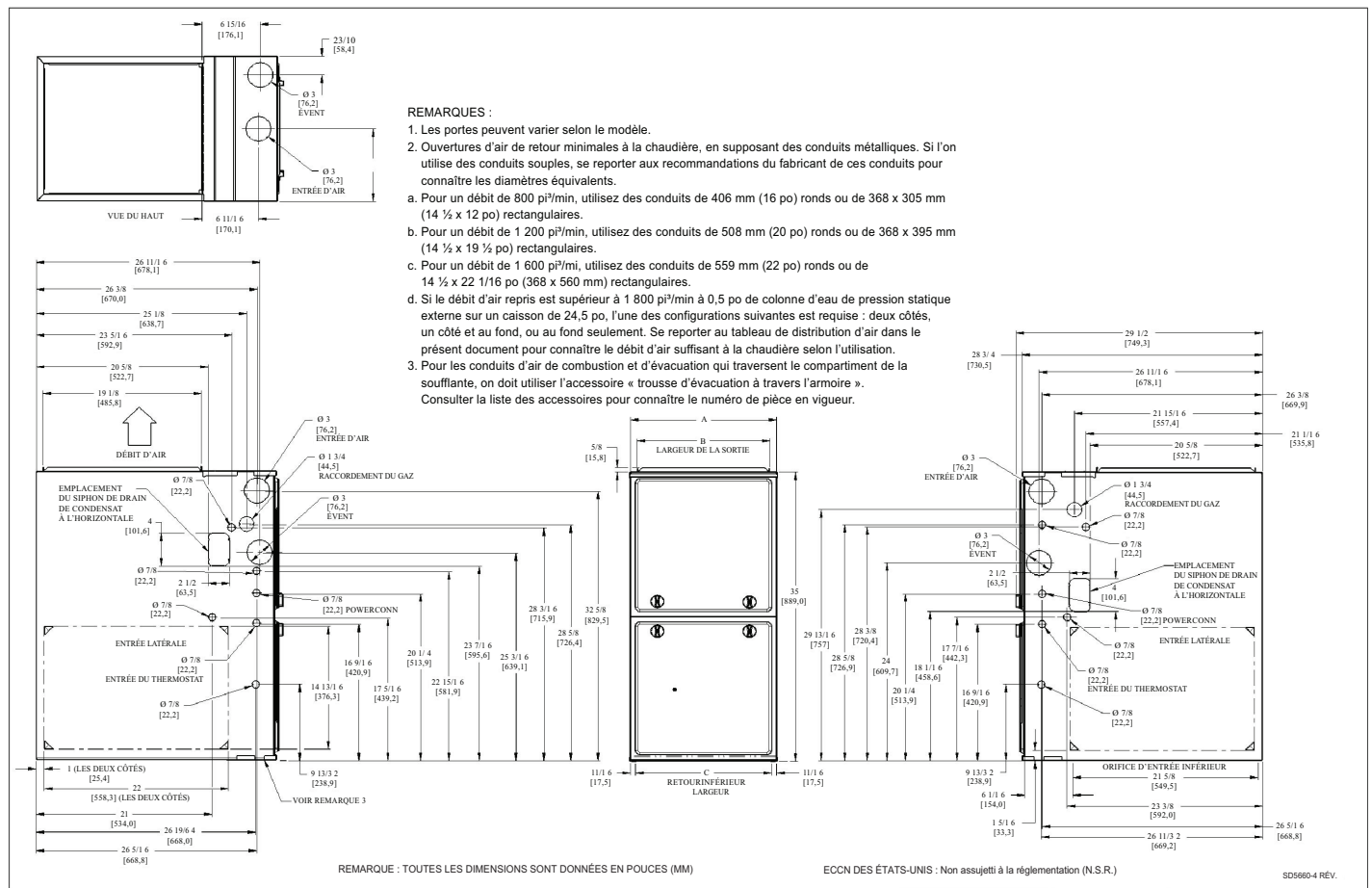
Fig. 1 – Schéma des cotes
