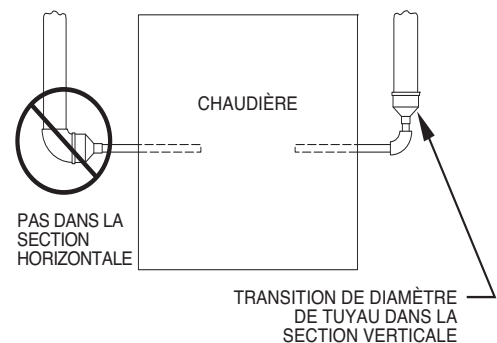
Fig. 50 – Emplacement des transitions de diamètre de tuyau de ventilation et d'air de combustion et configuration des coudes
