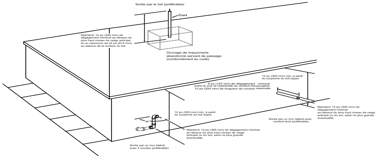
Fig. 41 – Air de combustion et sortie de ventilation pour système à ventilation directe (deux conduits)
