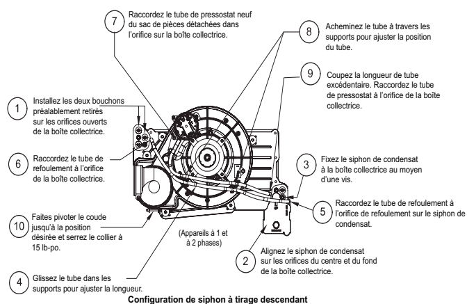
Fig. 9 – Configuration de siphon à tirage descendant (l'apparence peut varier) A11587FR
