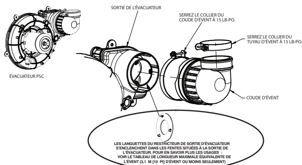
Fig. 57 – Raccordement des évents près de la chaudière
