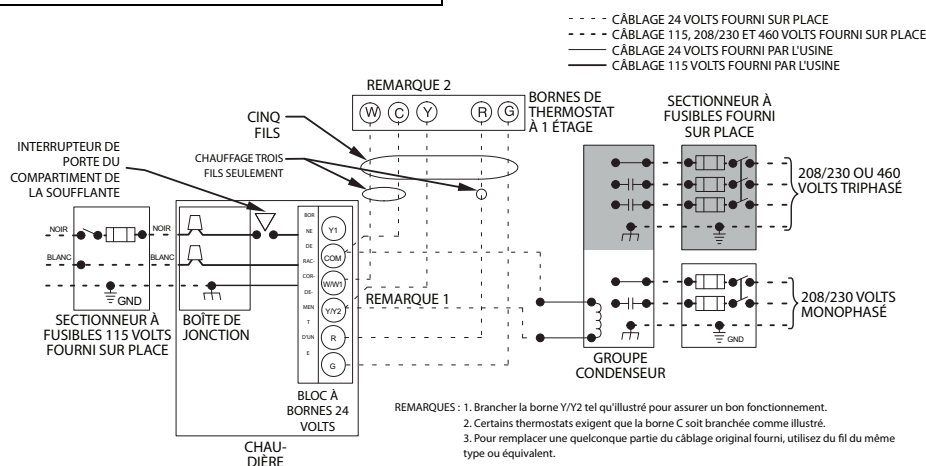
Fig. 33 – Schéma de câblage d'appareil à une phase type Tableau11 – Données électriques
