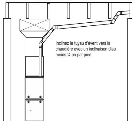
Fig. 57 – Raccordement des évents près de la chaudière
