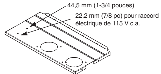
Fig. 31 – Entrée de gaz et d'électricité facultative
