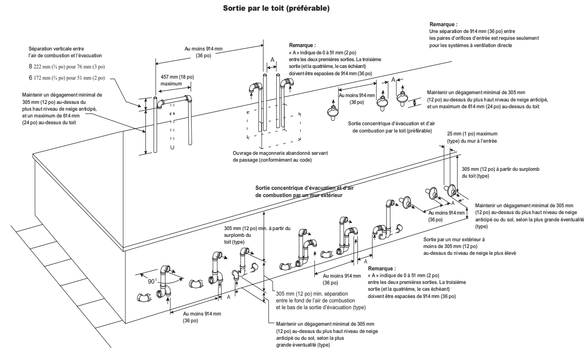
Fig. 41 – Air de combustion et sortie de ventilation pour système à ventilation directe (deux conduits)
