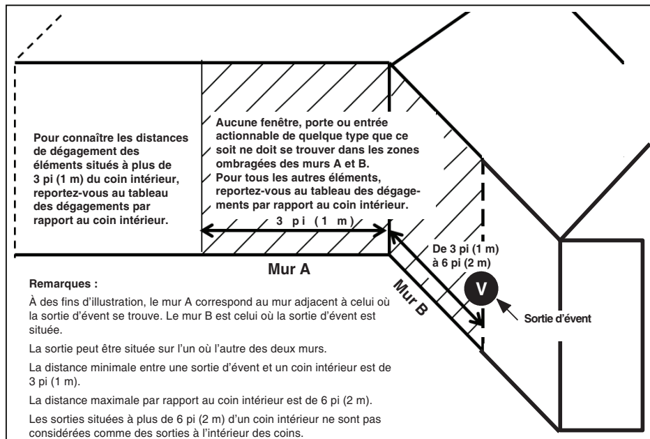
Fig. 45 – Sorties dans les coins intérieurs
