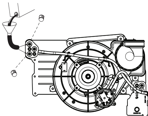
CONFIGURATION DE SIPHON À TRACÉ ASCENDANT APPAREILS A 1 ET A 2 PHASES
