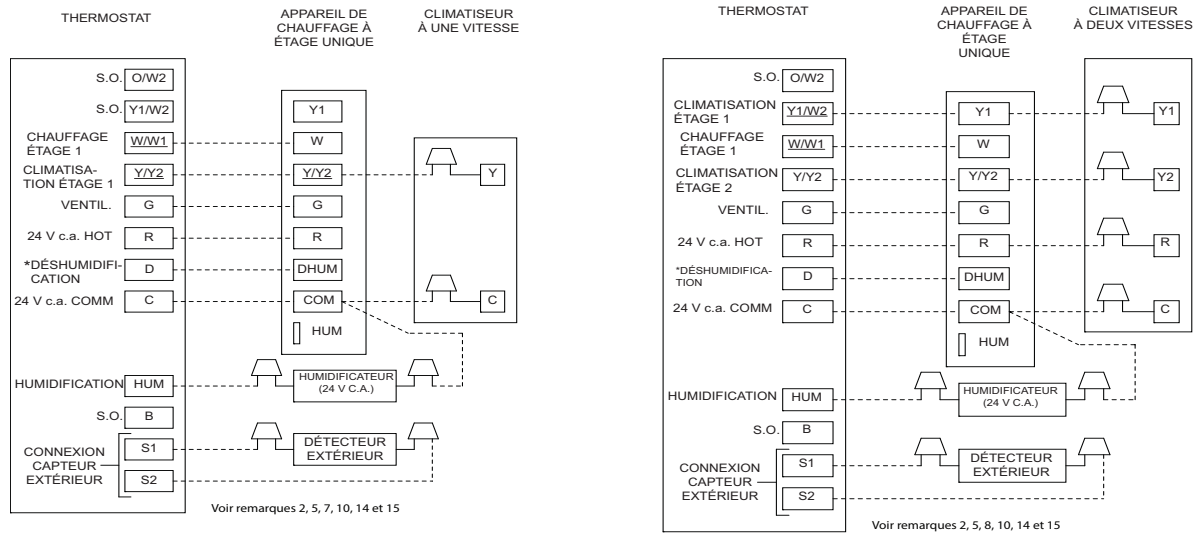
Chaudière à une phase avec climatiseur à une phase
