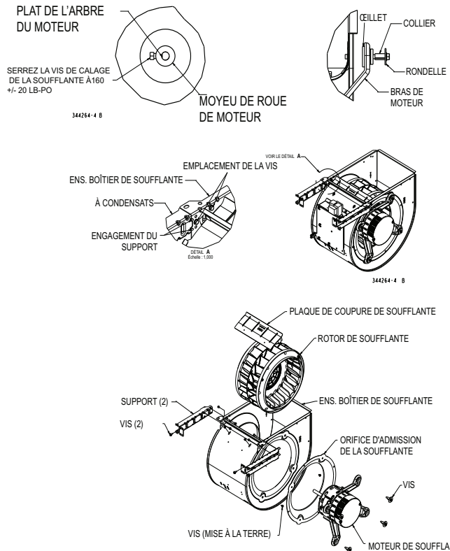
Fig. 67 – Ensemble de soufflante
