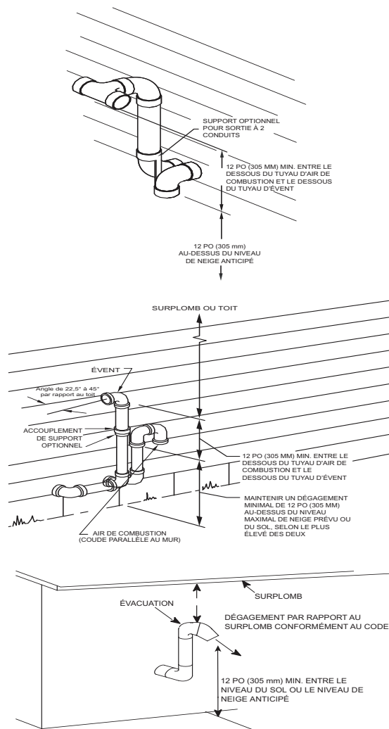
Fig. 49 – Sortie de ventilation pour l'Alberta et la Saskatchewan
