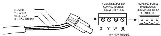
Fig. 37 – Connexion de communication de jumelage
