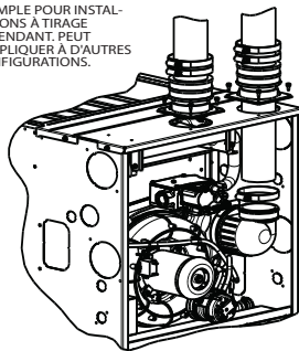
Fig. 46 – Exemple de raccordement de conduit d'admission d'air pour des systèmes de ventilation en polypropylène
