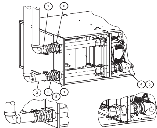
CONFIGURATION HORIZONTALE À DROITE ET VENTILATION VERTICALE
