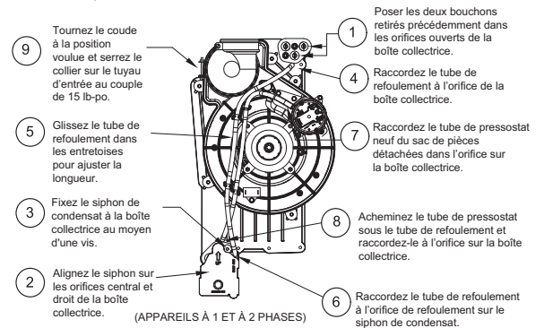
Siphon en configuration horizontale à gauche
