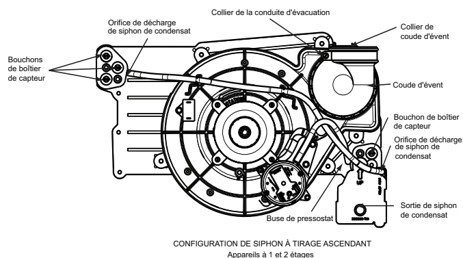
Fig. 8 – Configuration de siphon à tirage ascendant (l'apparence peut varier) A11307FR
