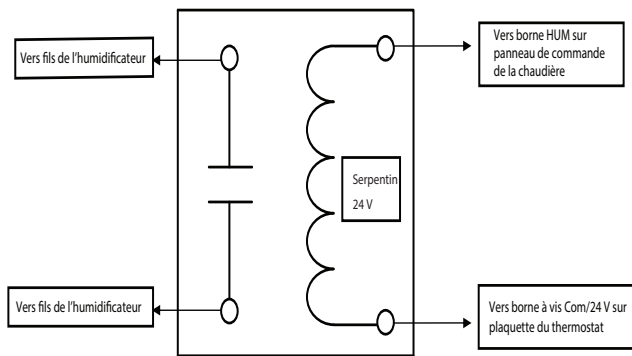
Fig. 38 – Relais d'isolation pour humidificateurs, fourni sur place, avec bloc d'alimentation interne
