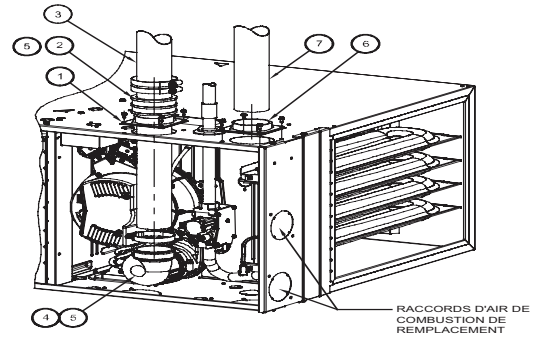
CONFIGURATION HORIZONTALE À DROITE ET VENTILATION VERTICALE
