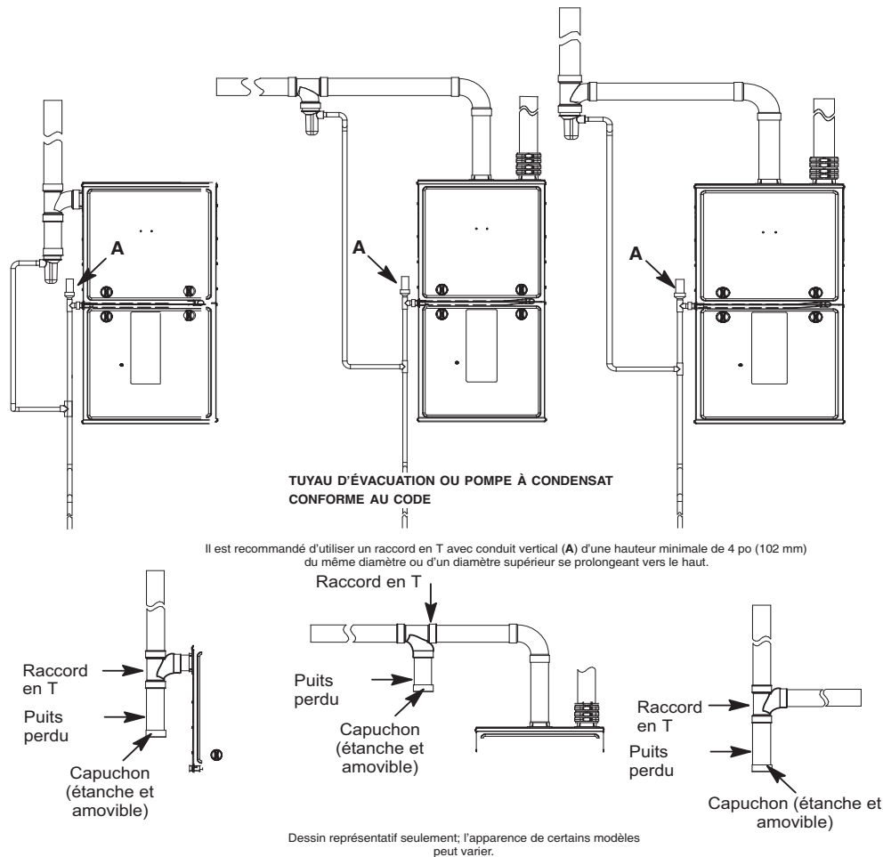
Fig. 52 – Siphon de condensat d'admission d'air de combustion recommandé
