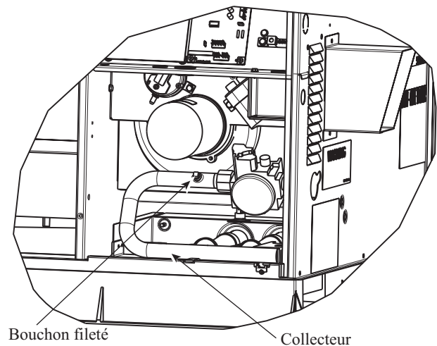
Figure 14 – Bloc brûleur
