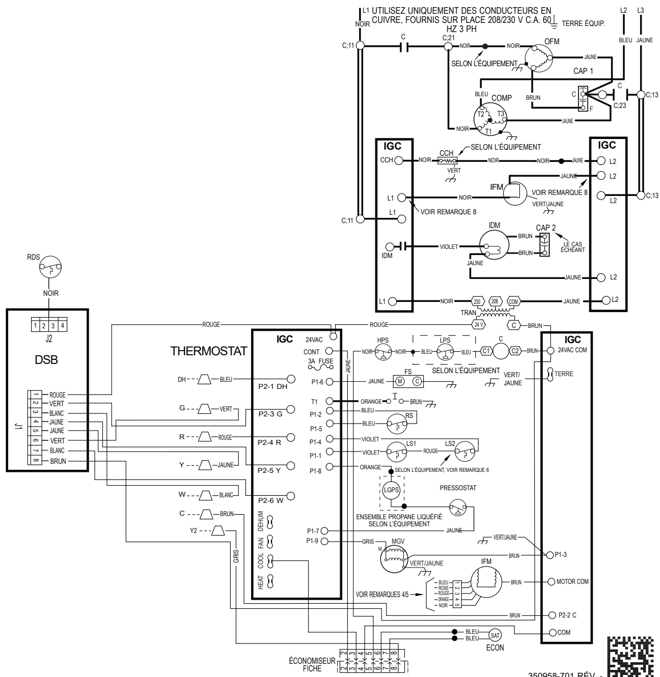
Figure 20 – Schéma de connexion en échelle 208/230-3-60
