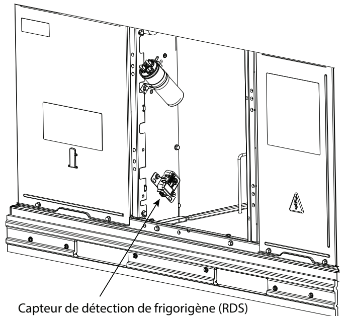
Figure 12 – Capteur de détection de frigorigène – Capacités d'appareil 24 et 30
