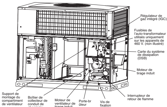
Figure 24 – Compartiment de ventilateur et boîtier de collecteur de conduit de cheminée
