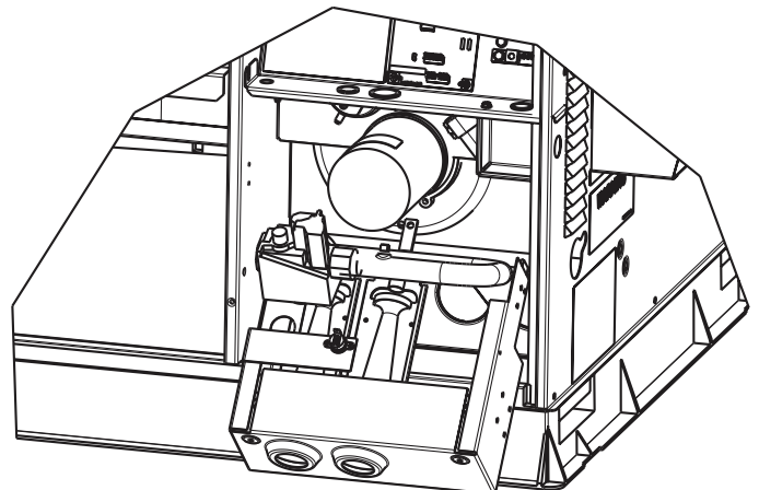
Figure 27 – Porte-brûleur retiré
