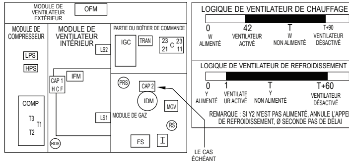
Figure 17 – Schéma de connexion de câblage 208/230-1-60
