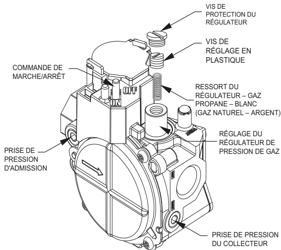
Figure 16 – Vanne de gaz à une phase
