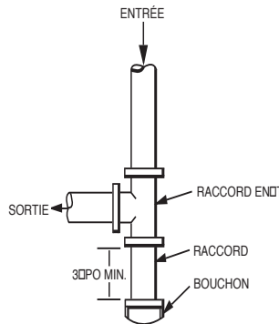
Figure 8 – Piège à sédiments
