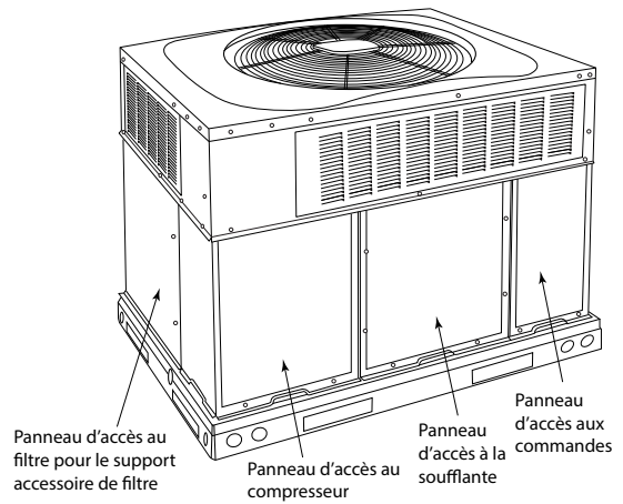
Figure 25 – Panneaux d'accès de l'appareil
