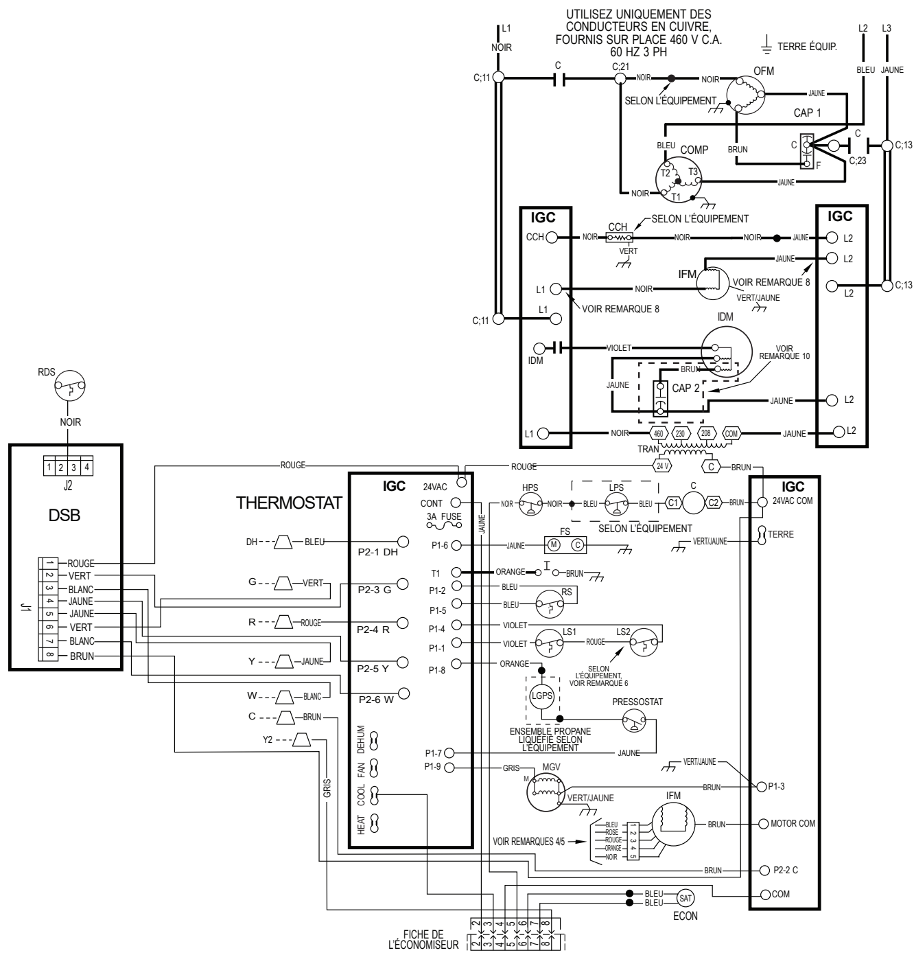
Figure 22 – Schéma de câblage en échelle 460-3-60
