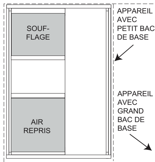
POSE DE L'APPAREIL SUR UN CADRE COMMUN
