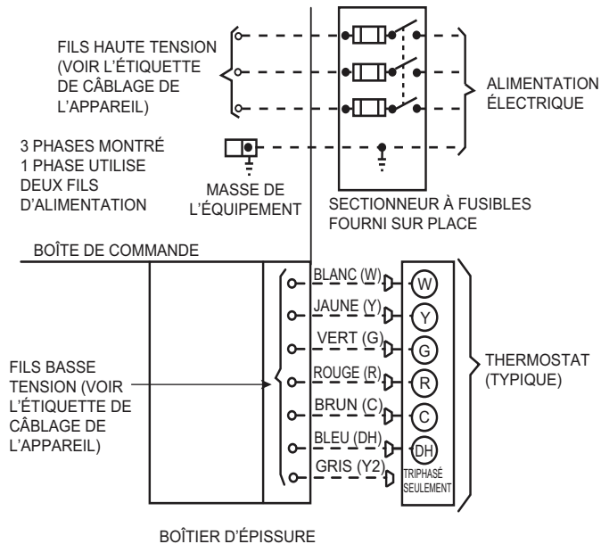
Figure 10 – Raccords haute et basse tensions
