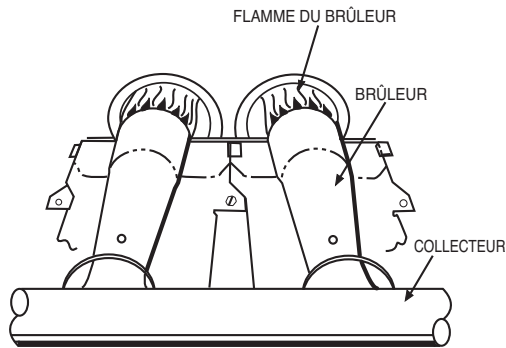
Figure 15 – Brûleur monoport
