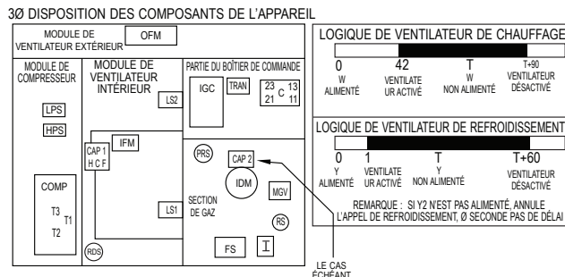
Figure 21 – Schéma de connexion de câblage 460-3-60
