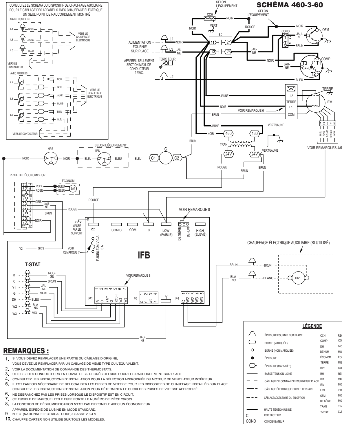
Fig. 16 – Schéma de connexion de câblage – 460-3-60
