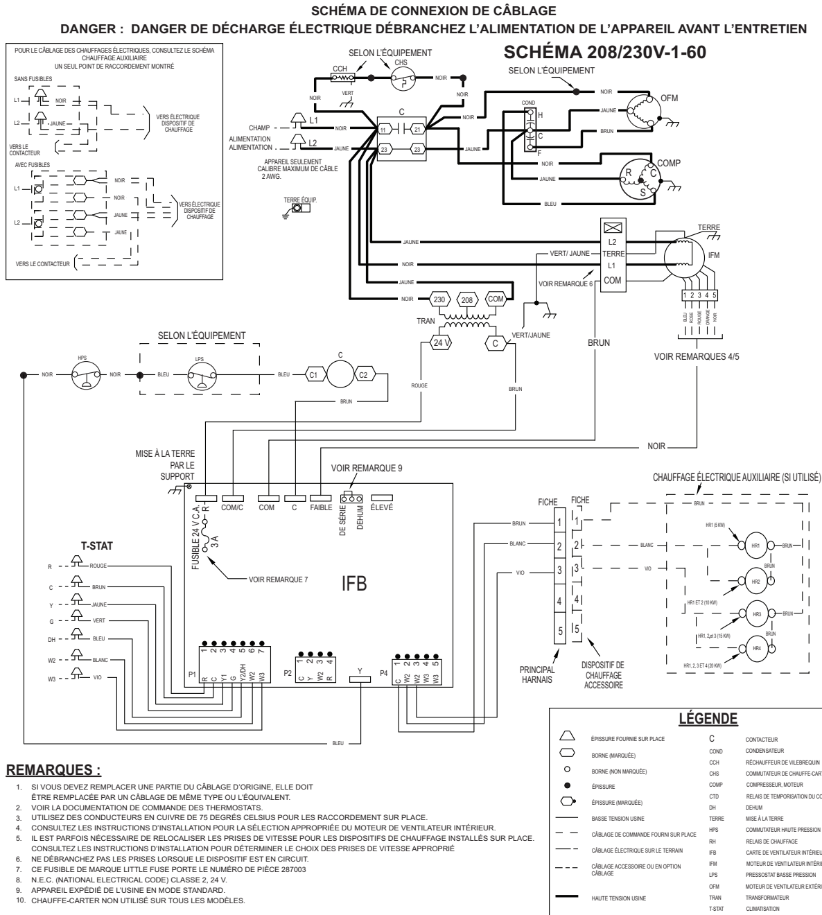
Fig. 12 – Schéma de connexion de câblage – 208/230V, 1 phase, 60Hz
