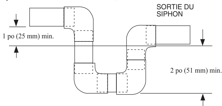
Fig. 8 – Siphon de condensat
