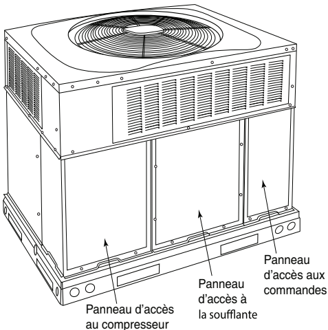
Fig. 20 – Panneaux d'accès de l'appareil
