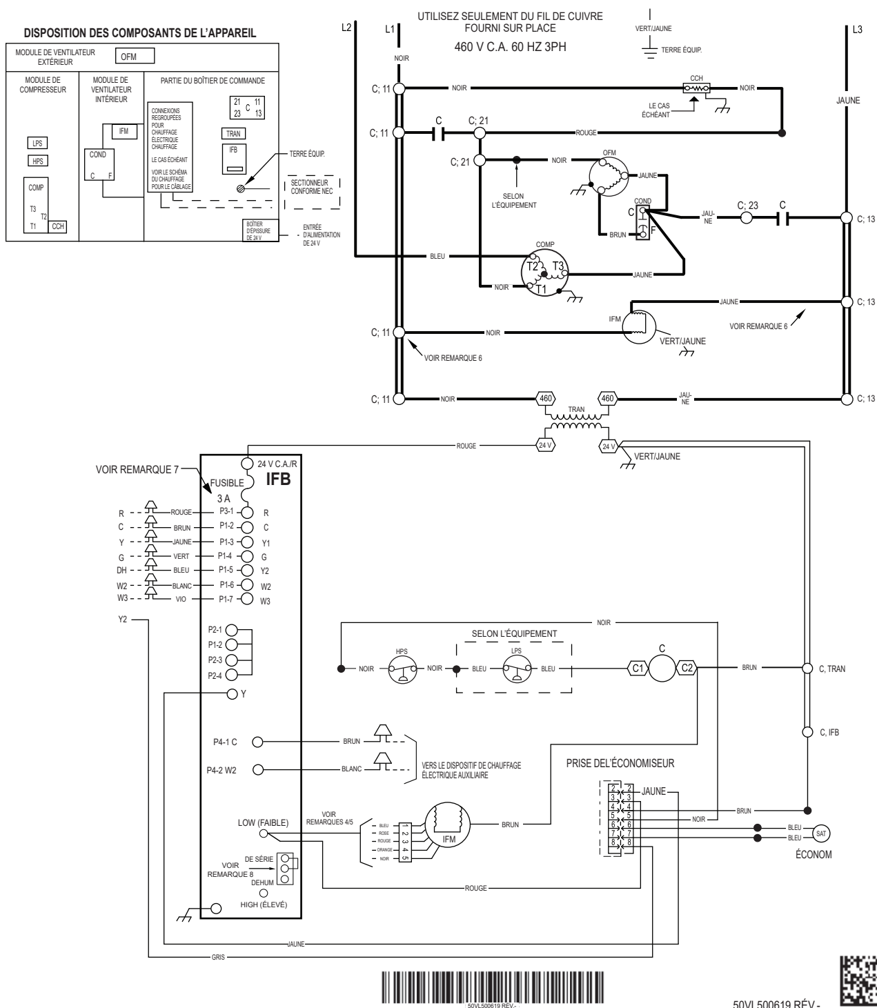
Fig. 17 – Schéma de câblage en échelle – 460-3-60
