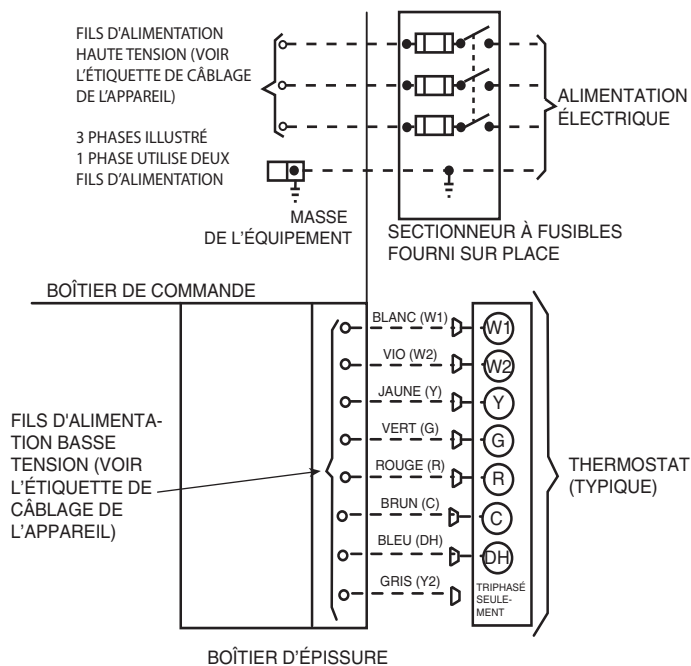
Fig. 10 – Branchements haute et basse tensions
