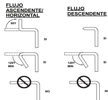
Fig. 17 – Bridas de conductos
