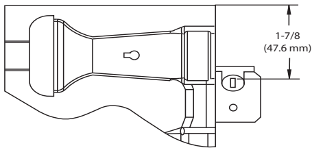
Fig. 56 – Posición del encendedor: vista superior
