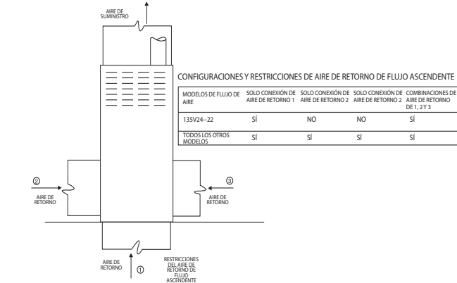
Fig. 19 – Configuraciones y restricciones de aire de retorno ascendente
