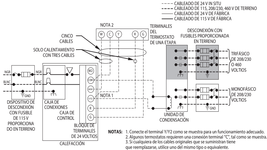
Fig. 24 – Diagrama de cableado de terreno Tabla 5 – Datos eléctricos
