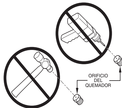
Fig. 51 – Abertura del orificio
