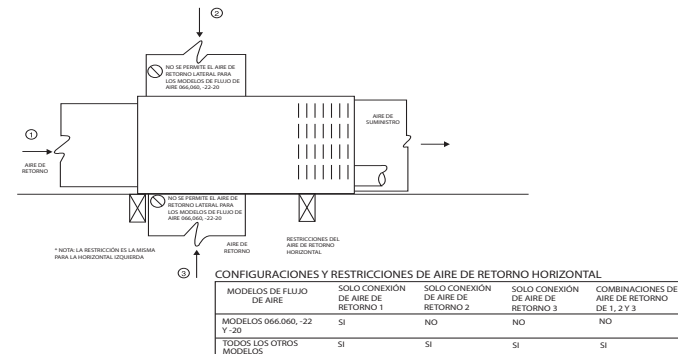
Fig. 20 – Configuraciones y restricciones de aire de retorno horizontal
