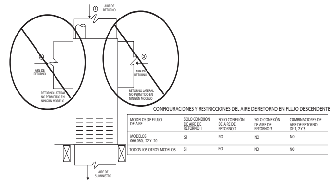
Fig. 18 – Configuraciones y restricciones del aire de retorno en flujo descendente
