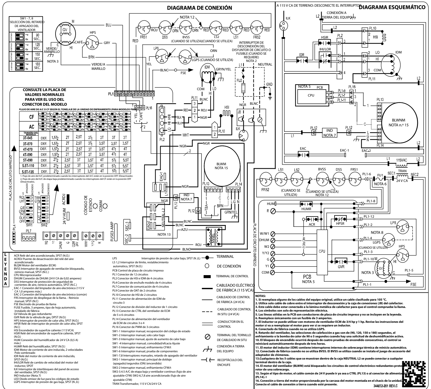
Fig. 59 – Diagrama eléctrico
