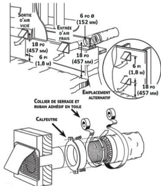
Fig. 12 – Hottes Extérieures
