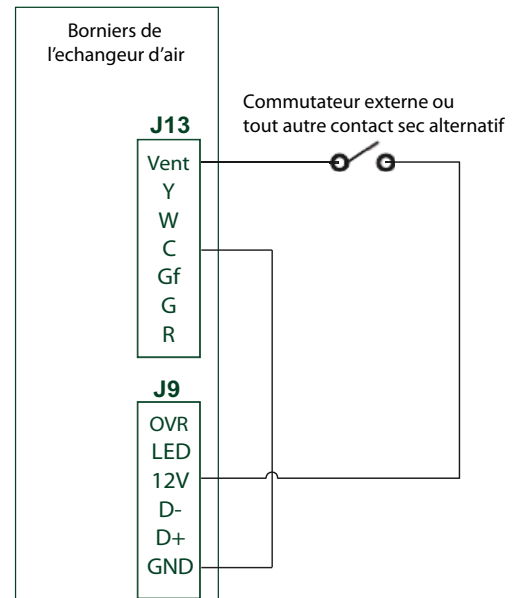
Fig. 18 – Câblage Alternatif Pour Une Installation Indépendante à Contact Sec (T-1)
