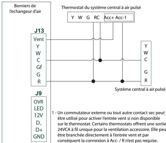
Fig. 17 – Câblage Pour Connexion Par Contact Sec
