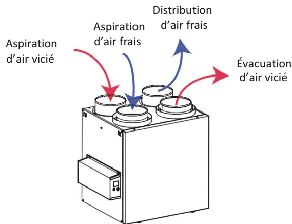
Fig. 1 – Distribution de l'Air
