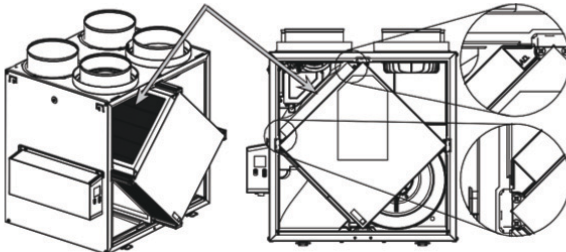
Fig. 28 – Filtre MERV13 en Option
