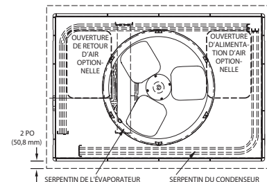
Figure 2 – Détails du montage sur dalle
