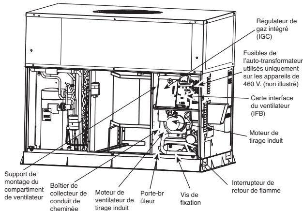
Figure 24 – Compartiment de ventilateur et boîtier de collecteur de conduit de cheminée
