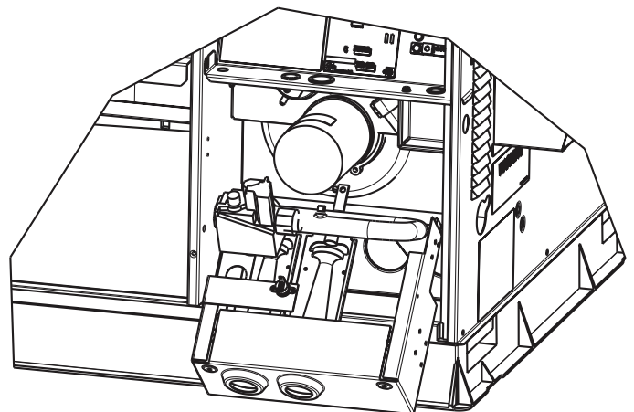
Figure 27 – Porte-brûleur retiré
