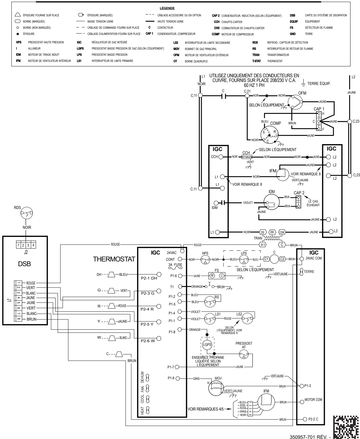
Figure 18 – Schéma de connexion en échelle 208/230-1-60
