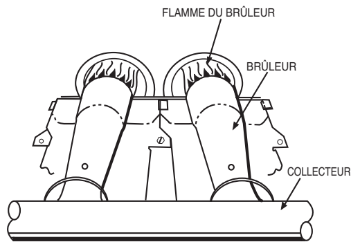
Figure 15 – Brûleur monoport
