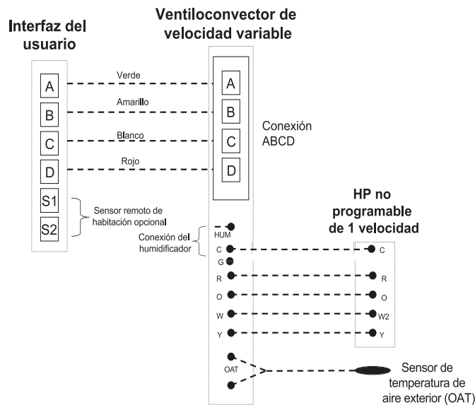
Fig. 3 – Diagrama de conexión del ventiloconvector FE con bomba de calor de una etapa sin comunicación
