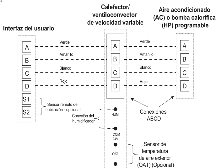
Fig. 1 – Diagrama de conexión de cuatro cables
