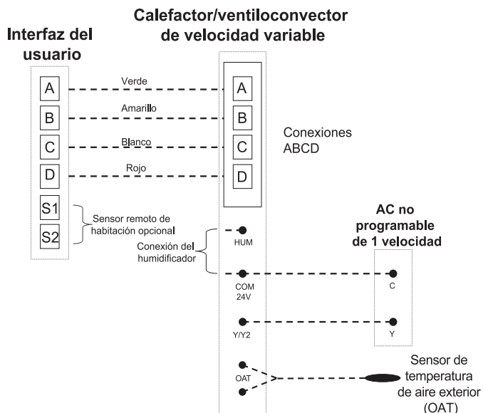
Fig. 2 – Diagrama de conexión del calefactor o el ventiloconvector FE con AA de una etapa
