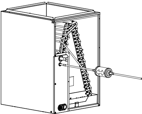
Fig. 6 – Filtro secador de la tubería de líquidos
