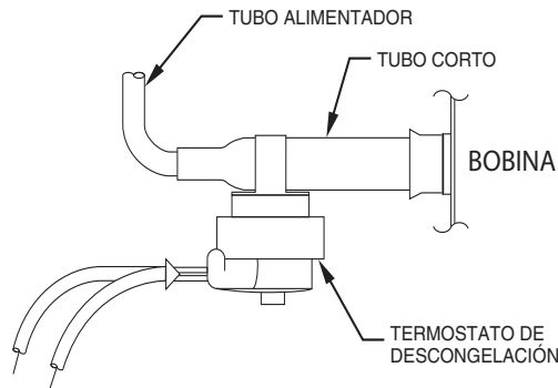
Fig. 3 – Ubicación del termostato de descongelación
