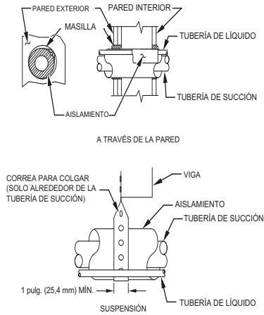
Fig. 1 – Instalación de la tubería de conexión
