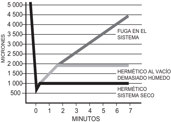
Fig. 7 – Gráfico de vacío profundo
