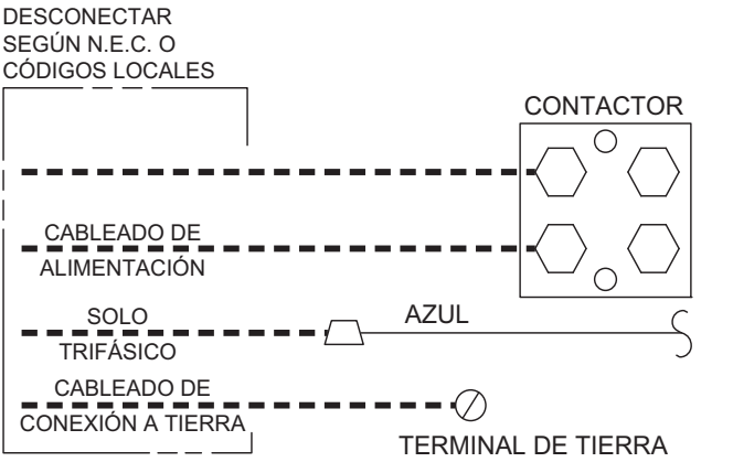
Fig. 8 – Conexiones de línea
