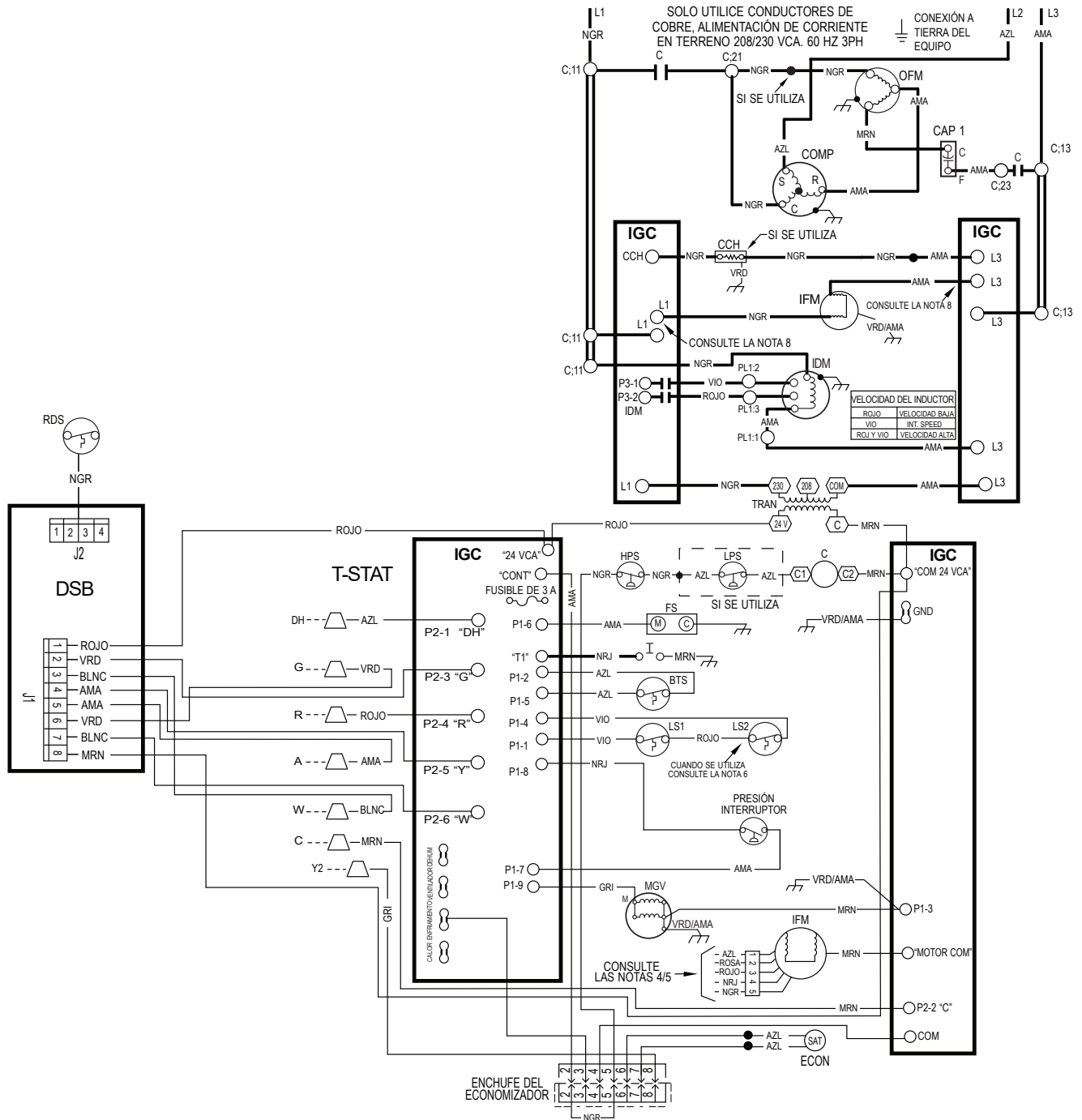
Fig. 21 – Diagrama eléctrico en escalera con NOx ultrabajo de 208/230-3-60, tamaño 30
