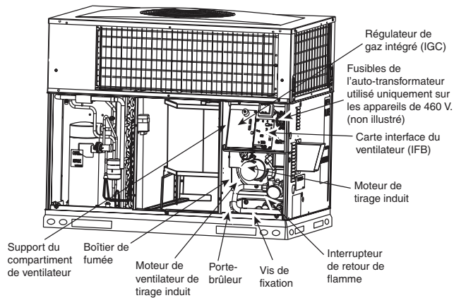
Figure 21 – Compartiment de ventilateur et boîtier de collecteur de conduit de cheminée
