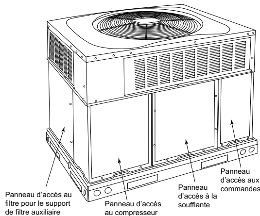
Figure 22 – Panneaux d'accès de l'appareil
