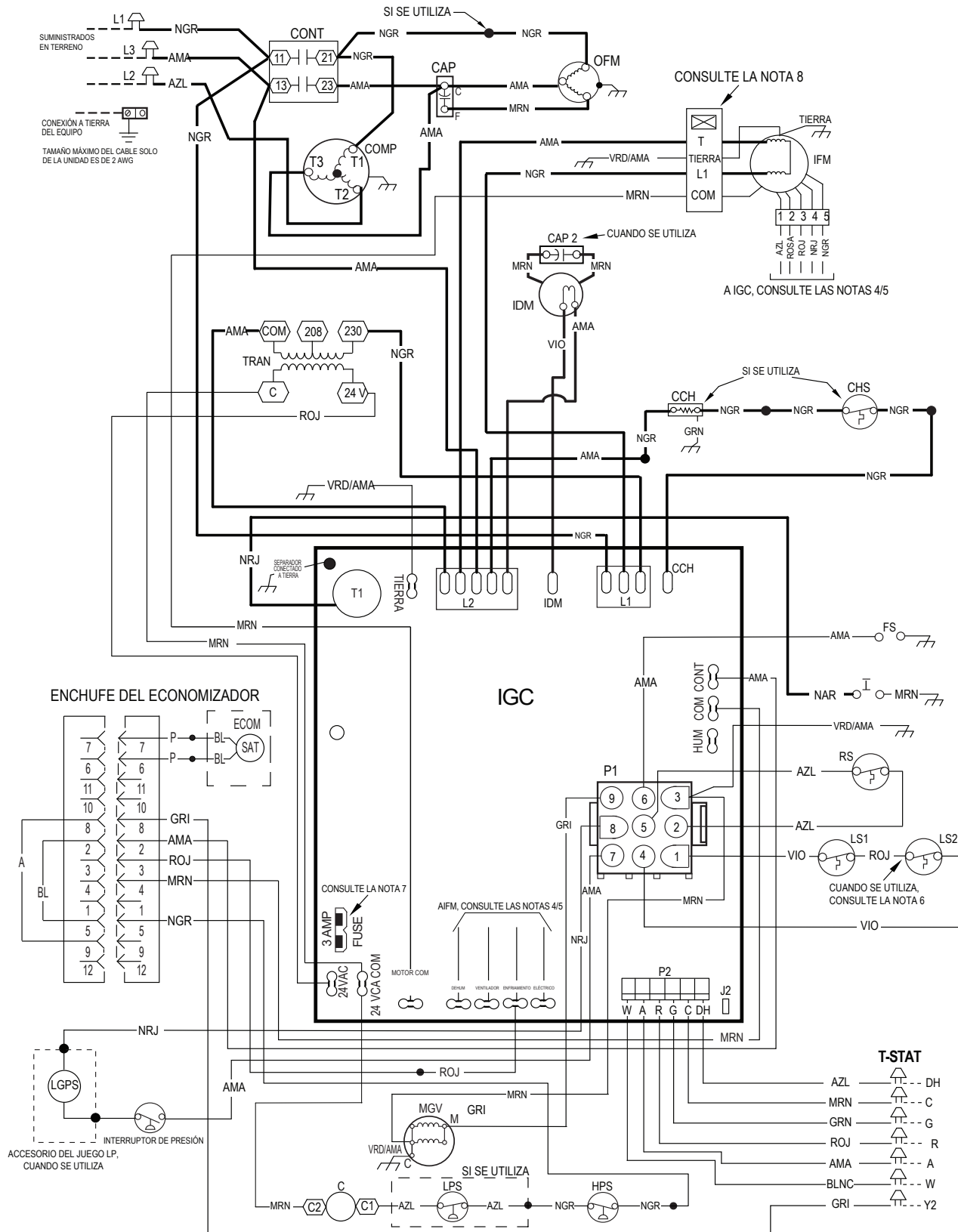
Fig. 16 – Diagrama eléctrico de conexión 208/230-3-60
