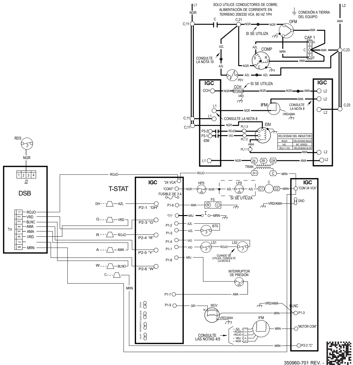
Fig. 19 – Diagrama eléctrico en escalera con NOx ultrabajo de 208/230-1-60, tamaño 30
