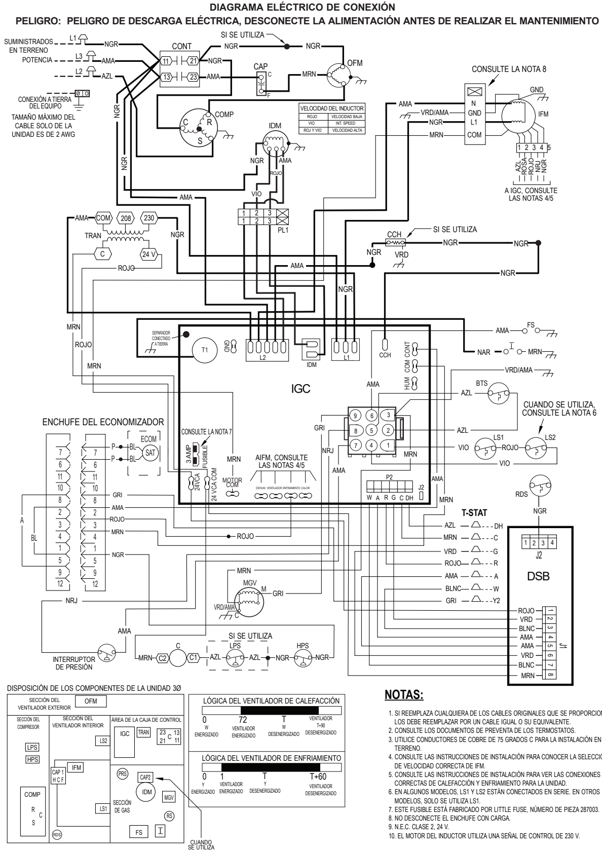
Fig. 20 – Diagrama eléctrico de conexión con NOx ultrabajo de 208/230-3-60
