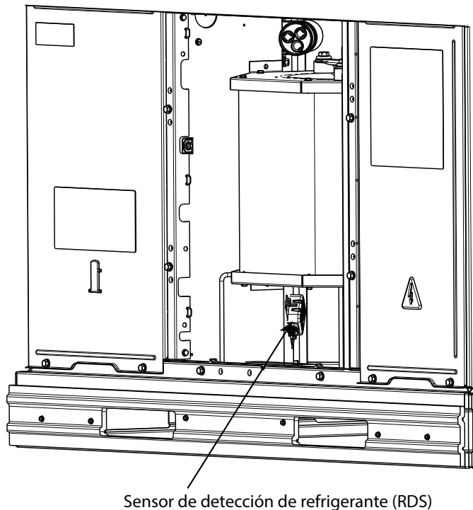
Fig. 13 – Sensor de detección de refrigerante de tamaños 36 y 60
