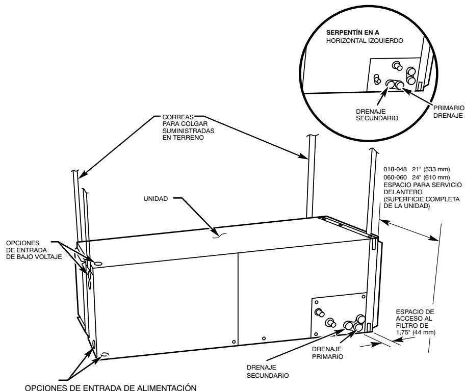
Fig. 3: Serpentín inclinado en aplicación horizontal izquierda (configuración de fábrica)
