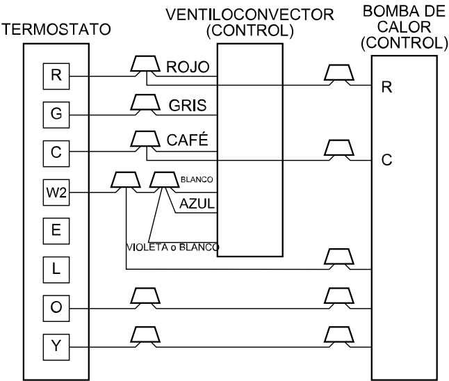
Fig. 12: Disposición del cableado, unidad de bomba de calor (Enfriamiento y calefacción de 2 etapas sin termostato exterior)
