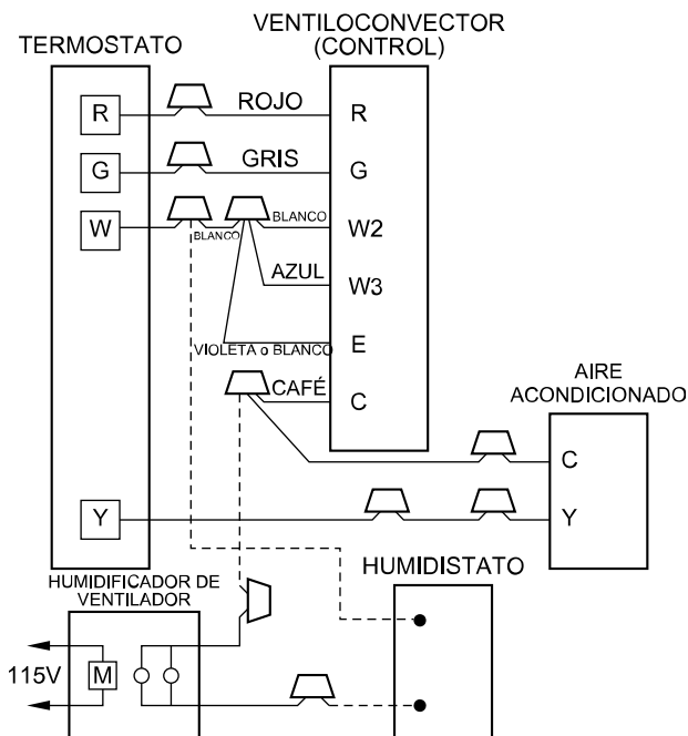
Fig. 21: Disposición del cableado del humidificador al ventiloconvector con calor eléctrico
