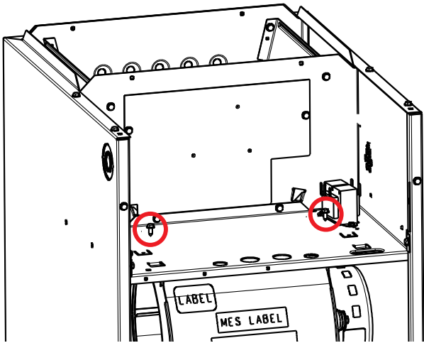
Fig. 22: Tornillos de envío
