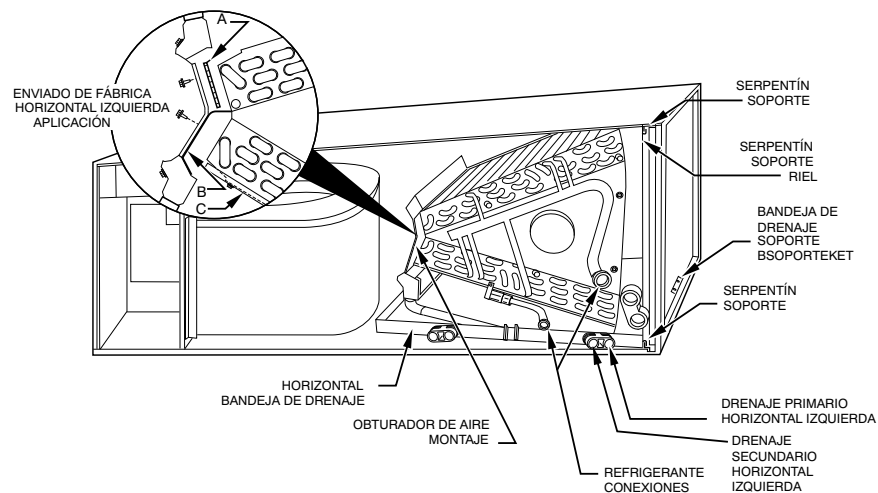
Fig. 4: Serpentín en A en aplicación horizontal izquierda (configuración de fábrica)
