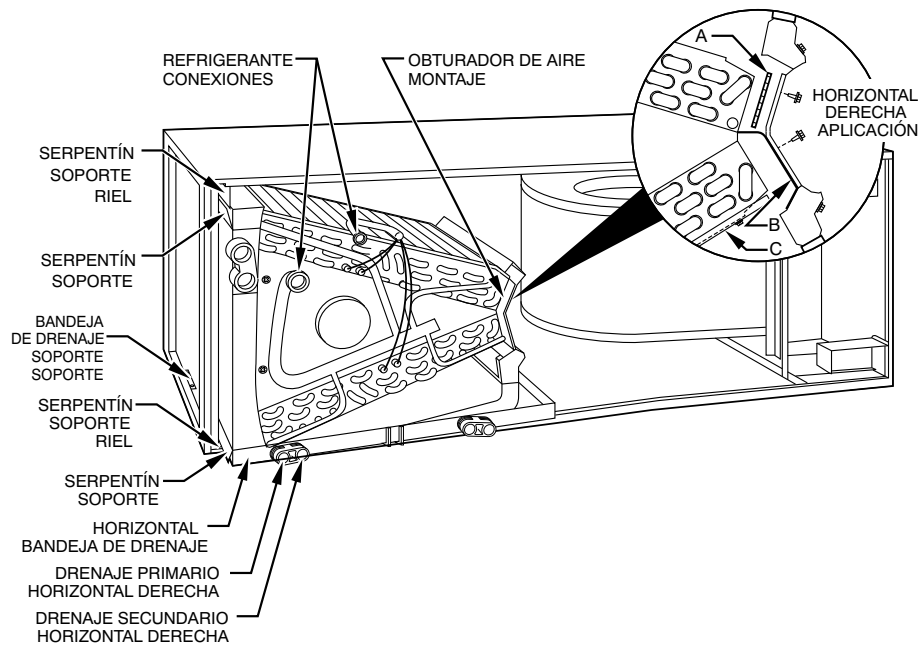
Fig. 6: Conversión para aplicaciones horizontales derechas - Serpentin en A
