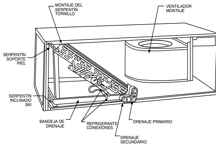
Fig. 5: Conversión para aplicaciones horizontales derechas - Serpentín inclinado
