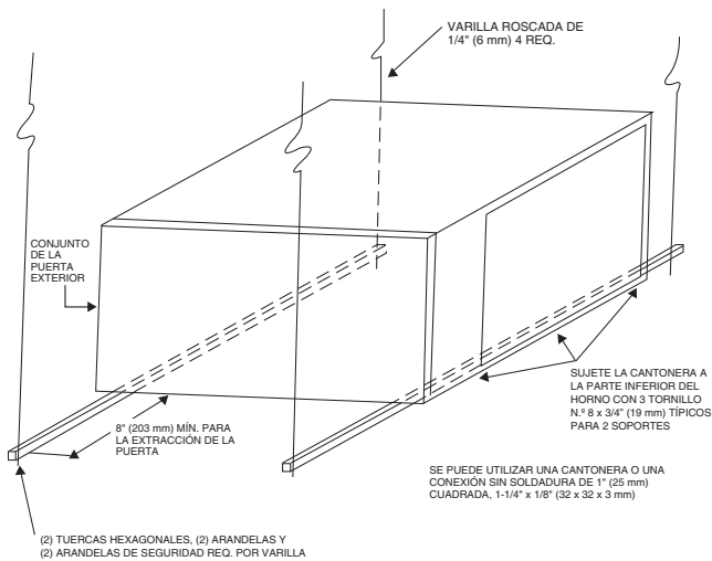
Fig. 15 – Suspensión horizontal de la unidad
