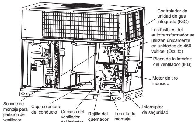
Fig. 21 – Carcasa del ventilador y caja colectora del conducto
