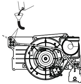
Fig. 60 – Amorçage du siphon de condensat (l'apparence peut varier)
