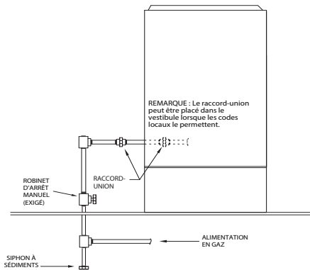
Fig. 31 – Disposition type de la tuyauterie de gaz
