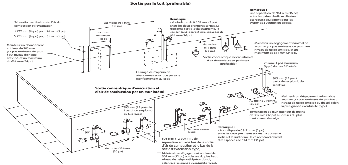
Fig. 40 – Air de combustion et sortie d'évent pour système d'évacuation directe (2 tuyaux)
