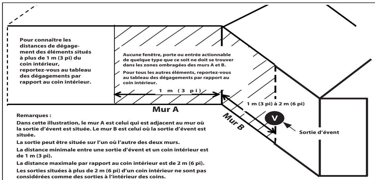
Fig. 44 – Sorties dans les coins intérieurs
