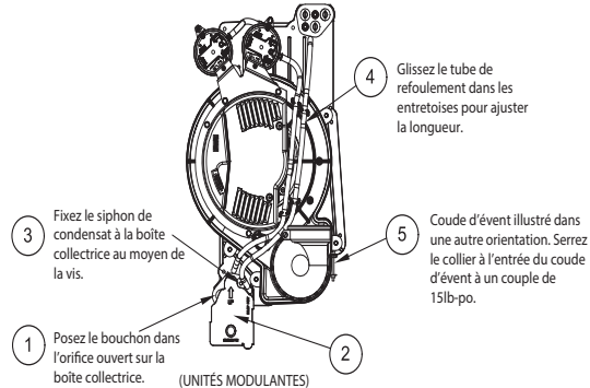
Configuration de siphon horizontal à droite
