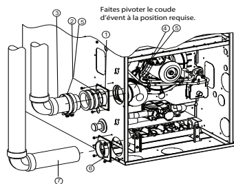
CONFIGURATION À GAUCHE À TIRAGE DESCENDANT
