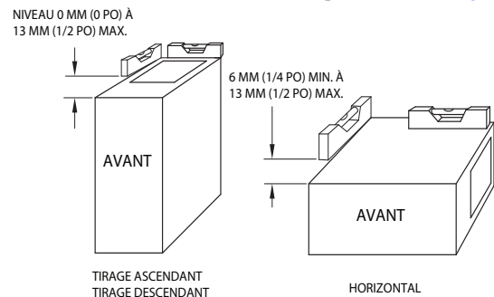
Fig. 18 – Exigences d'inclinaison de la chaudière
