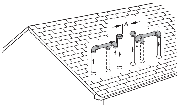
Fig. 46 – Sortie d'évacuation et de combustion
