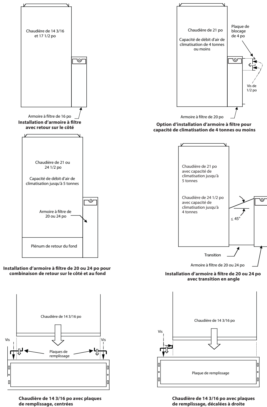
Fig. 25 – Filtre de boîtier
