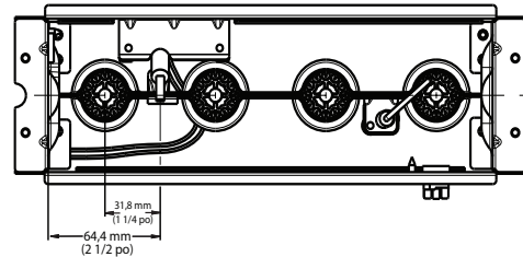
Fig. 69 – Position de l'allumeur - vue du haut
