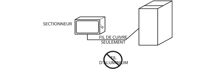
Fig. 33 – Coffret électrique externe fourni sur place sur le caisson de la chaudière
