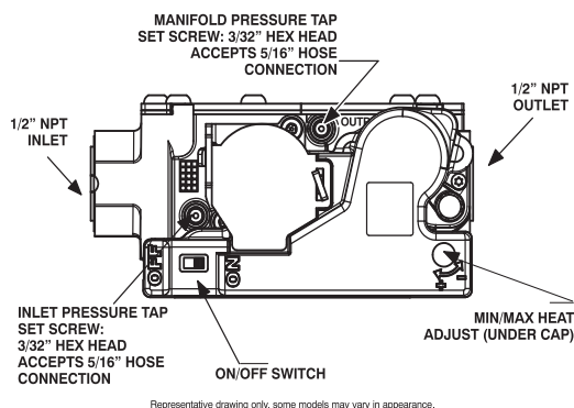
Fig. 62 – Vanne de gaz avec orifices de pression
