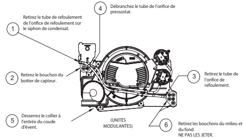
Configuration non convertie en usine telle que vue dans l'orientation à tirage descendant
