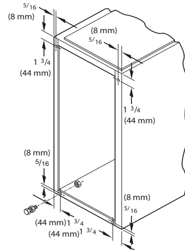
Fig. 28 – Pattes de mise à niveau
