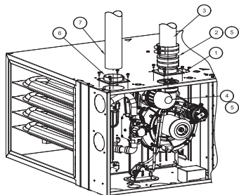
CONFIGURATION HORIZONTALE À GAUCHE ET VENTILATION VERTICALE
