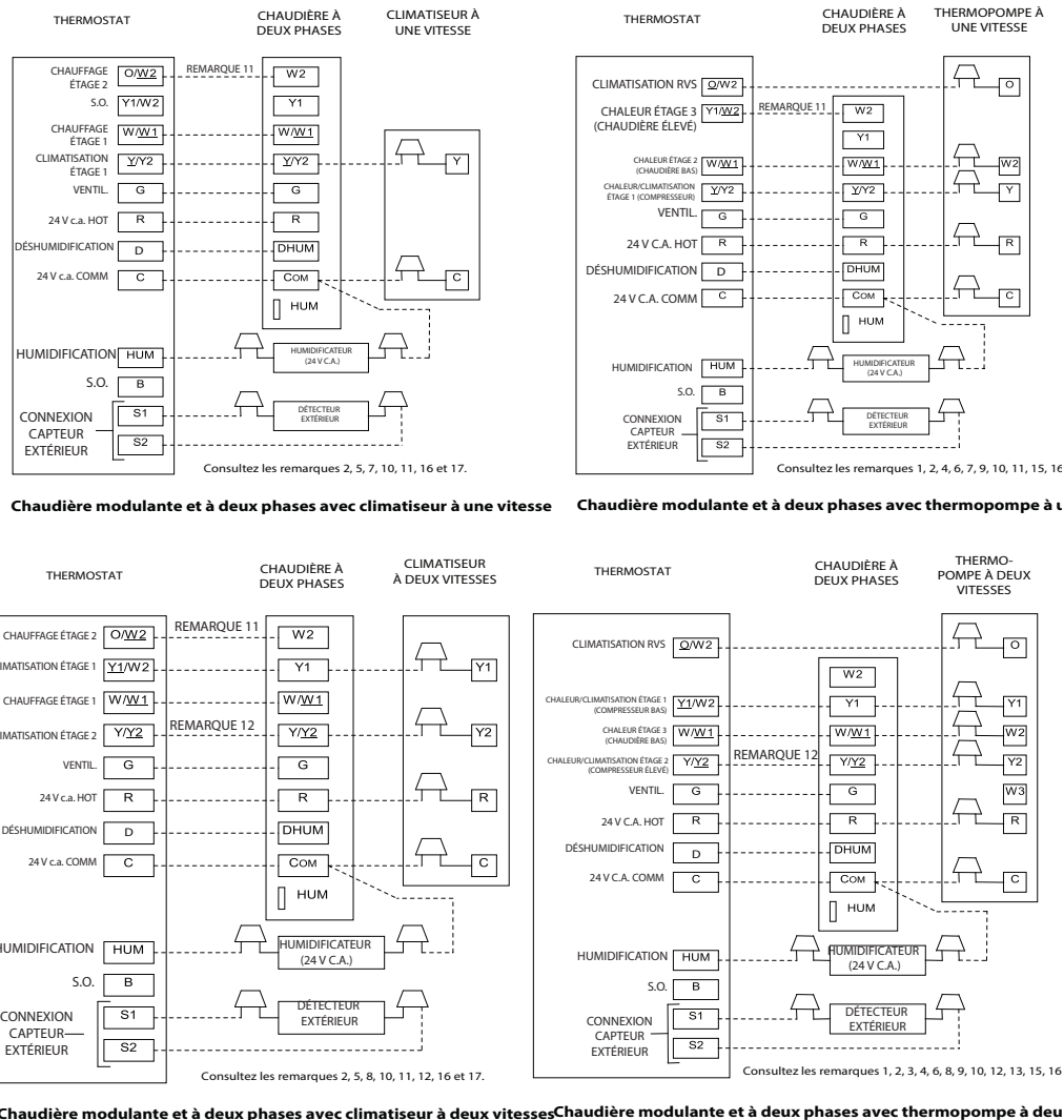
Fig. 39 – Schémas de câblage de thermostat
