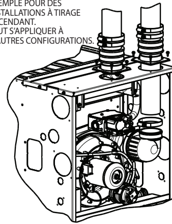
Fig. 50 – Exemple de raccordement de tuyau d'entrée d'air pour des systèmes de ventilation en polypropylène A12220FR
