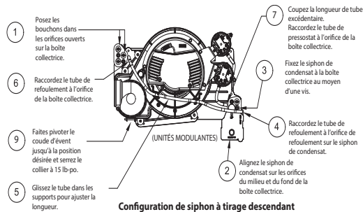
Configuration de siphon à tirage descendant
