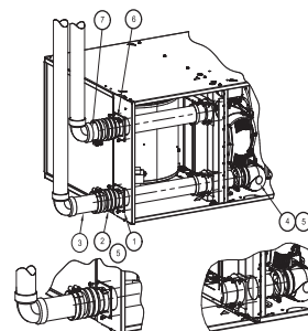
CONFIGURATION HORIZONTALE À DROITE ET VENTILATION VERTICALE
