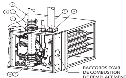
CONFIGURATION HORIZONTALE À DROITE ET VENTILATION VERTICALE
