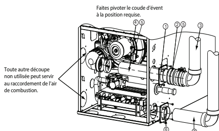
CONFIGURATION À DROITE À TIRAGE DESCENDANT
