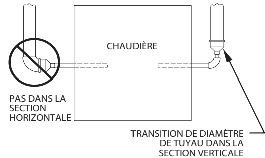
Fig. 48 – Emplacement des transitions de diamètre de tuyau de ventilation de l'air de combustion et configuration des coudes A93034FR
