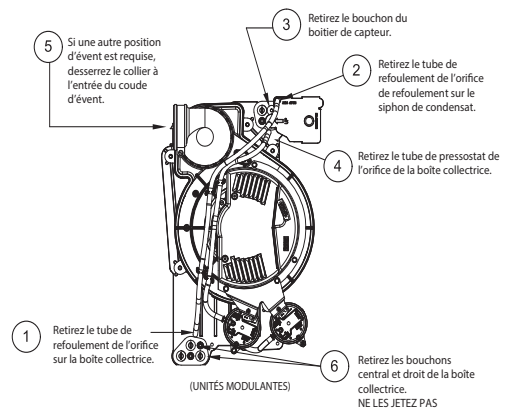
Configuration de siphon non convertie en usine telle que vue en position horizontale à gauche
