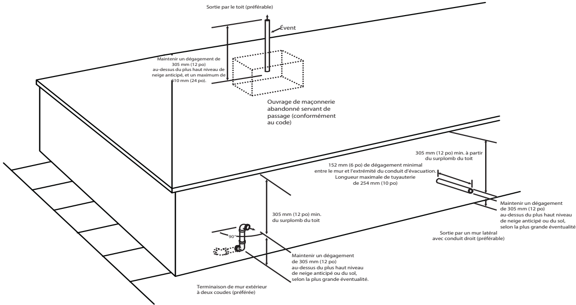
Fig. 41 – Sortie d'évent pour système d'évacuation non directe et d'air de combustion
