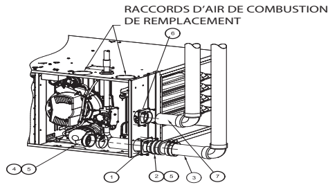
CONFIGURATION HORIZONTALE À DROITE ET VENTILATION À DROITE
