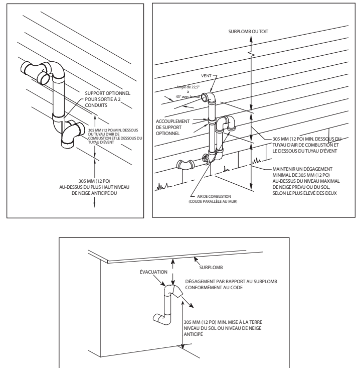
Fig. 49 – Sortie d'évent pour l'Alberta et la Saskatchewan A13078FR
