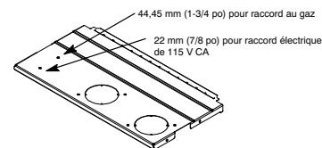
Fig. 30 – Entrée de gaz et d'électricité facultative
