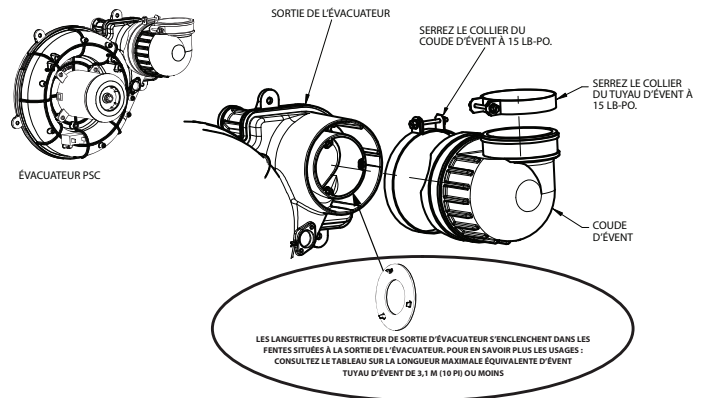
Fig. 53 – Coude d'évent d'évacuateur (l'apparence peut varier)
