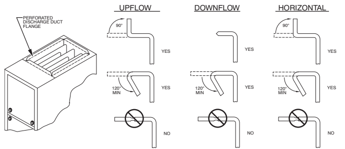
Fig. 19 – Brides d'attache de la conduite
