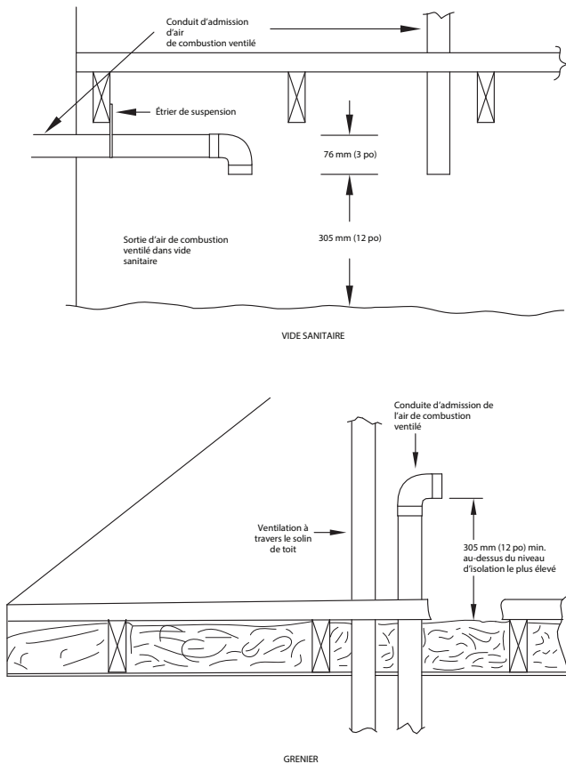
Fig. 47 – Sorties d'évent pour système à air de combustion ventilé A10497FR
