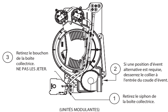
Configuration de siphon non convertie en usine telle que vue en configuration horizontale à droite
