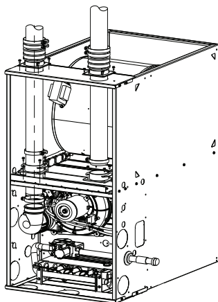
CONFIGURATION À DROITE À TIRAGE DESCENDANT
