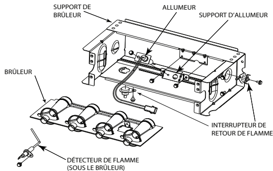
Fig. 68 – Ensemble du brûleur
