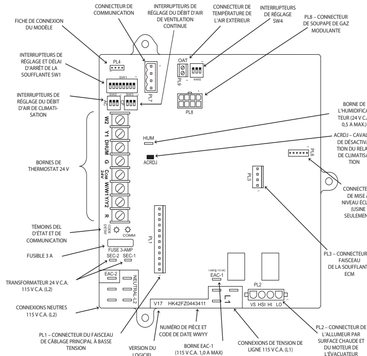
Fig. 37 – Exemple de commande de chaudière modulante
