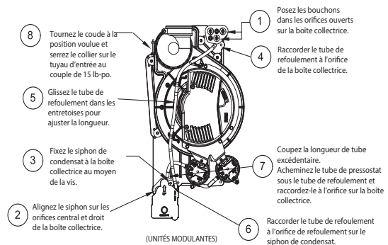
Siphon en configuration horizontale à gauche
