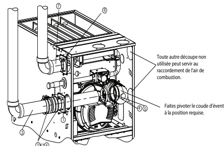
CONFIGURATION À GAUCHE À TIRAGE ASCENDANT
