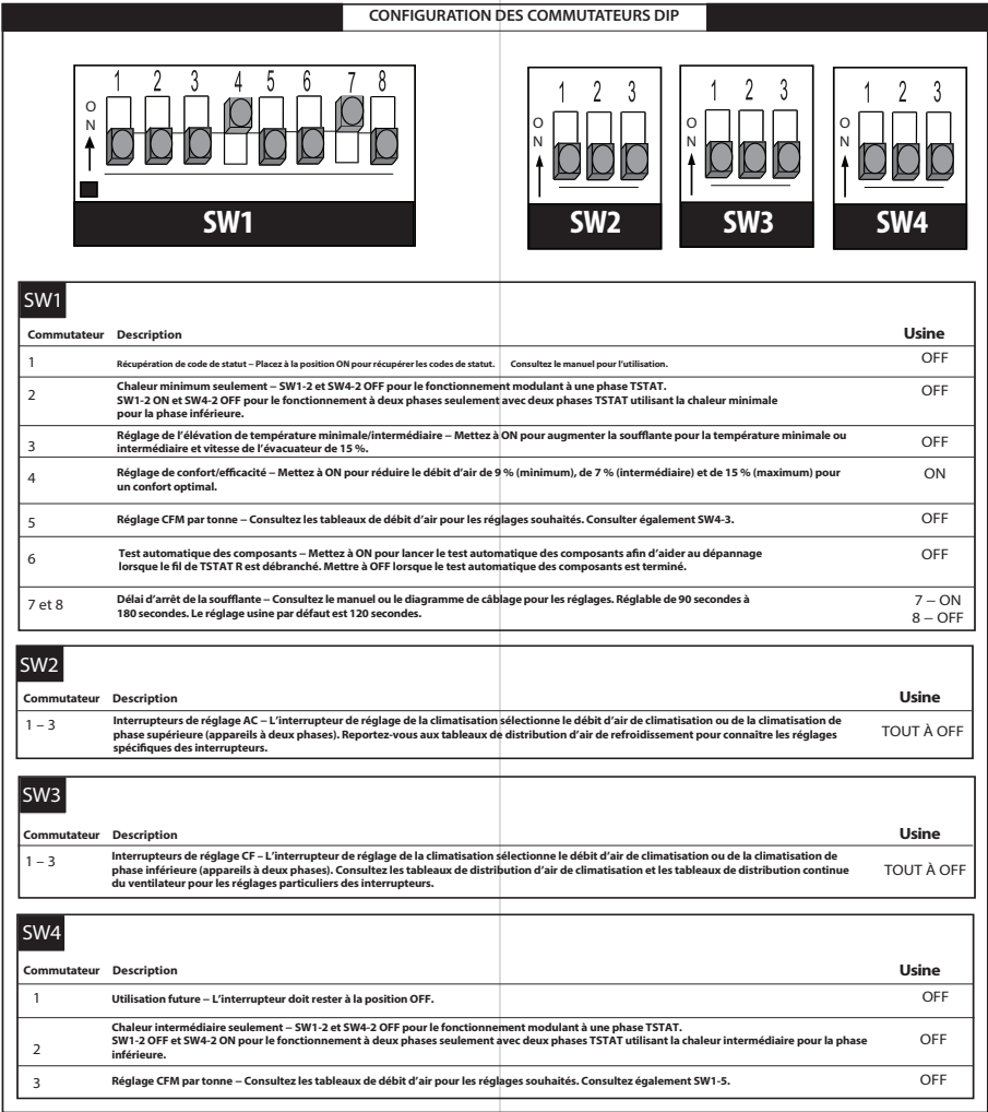
Fig. 59 – Description des interrupteurs de réglage de la chaudière
