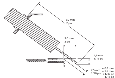
Fig. 70 – Position de l'allumeur - vue latérale
