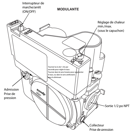
Fig. 63 – Vanne de gaz sans orifices de pression
