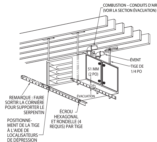
Fig. 26 – Plateforme de travail pour installation dans le grenier
