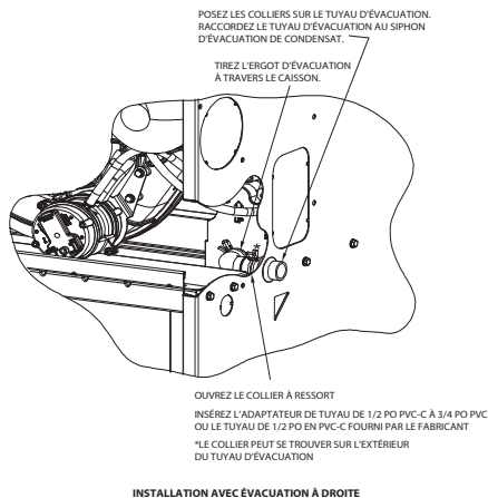
Fig. 13 – Œillet d'évacuation de condensat formé en caoutchouc AJ1342AFR
