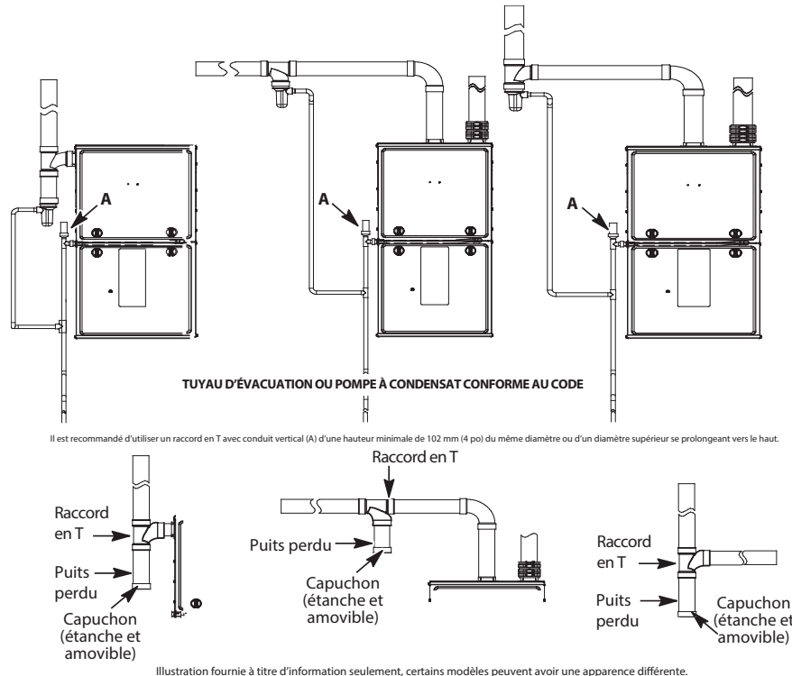
Fig. 51 – Siphon de condensat d'air de combustion recommandé
