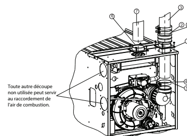
VENTILATION VERTICALE À TIRAGE ASCENDANT
