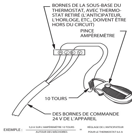
Fig. 65 – Vérification d'appel de courant à l'aide de l'ampèremètre Réglage de l'anticipateur de chaleur du thermostat
