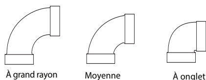
CONFIGURATIONS DES COUDES
