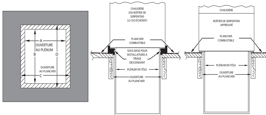
Fig. 24 – Installation sur revêtement de plancher combustible
