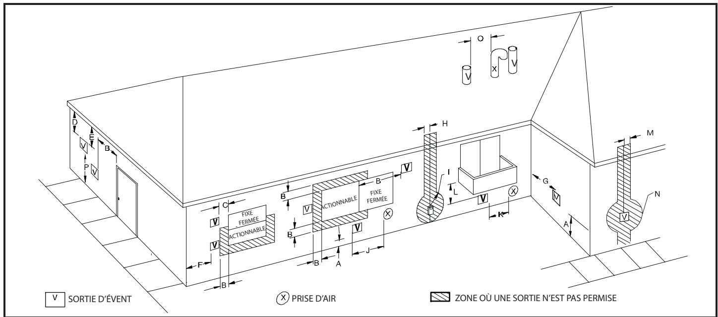
Fig. 42 – Dégagement de sortie à évacuation directe
