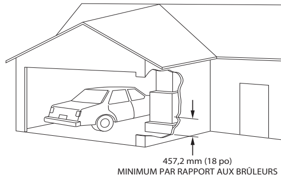
Fig. 5 – Installation dans un garage
