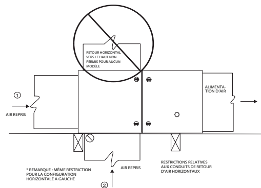
Fig. 22 – Configurations et restrictions des conduits de retour horizontal de retour d'air horizontal
