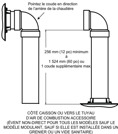
Fig. 45 – Fixation du tuyau d'air de combustion
