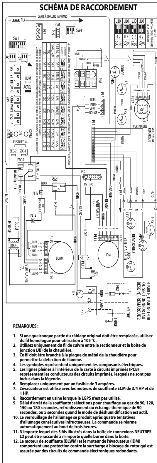
Fig. 73 – Schéma de câblage
