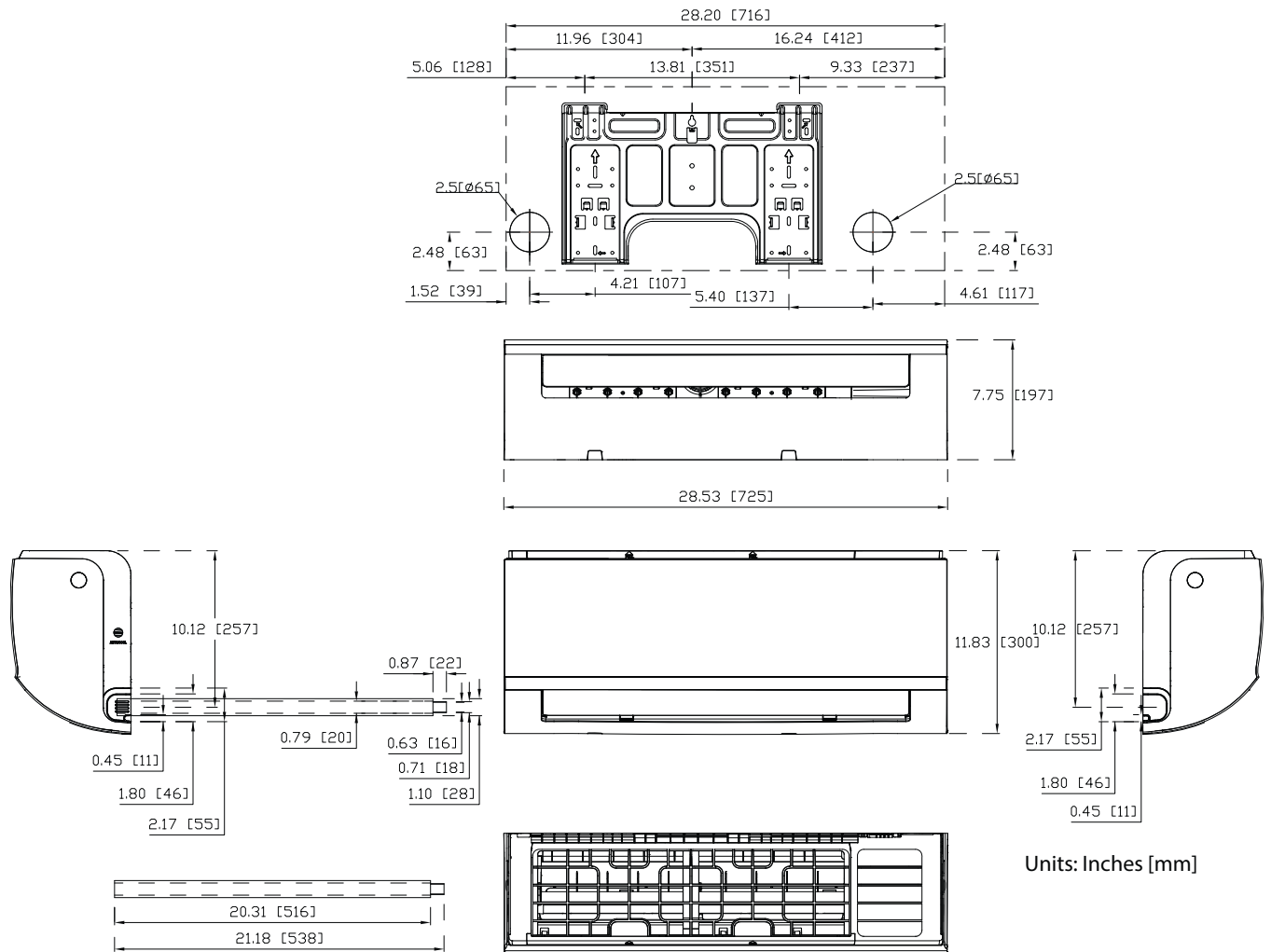
Fig. 4 — Dimensions Size 9K
