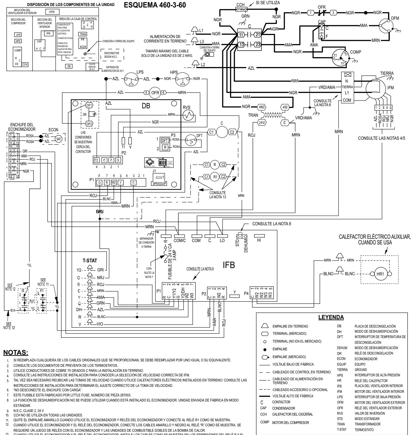
Fig. 16 – Diagrama eléctrico de conexión 460-3-60
