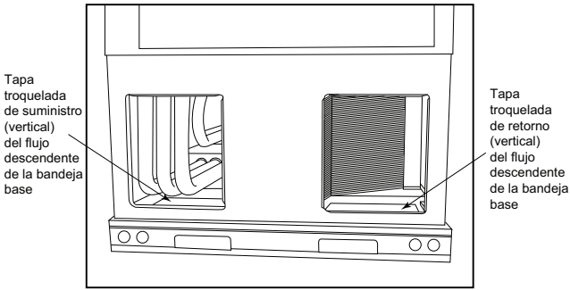
Fig. 6 – Abertura del conducto de alimentación y retorno
