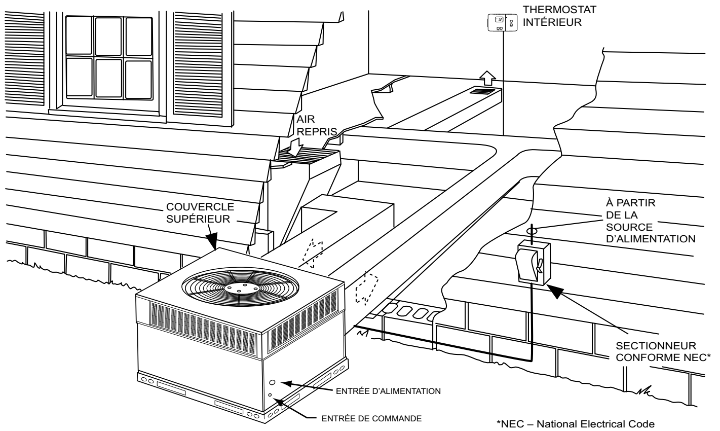
Fig. 11 – Installation typique
