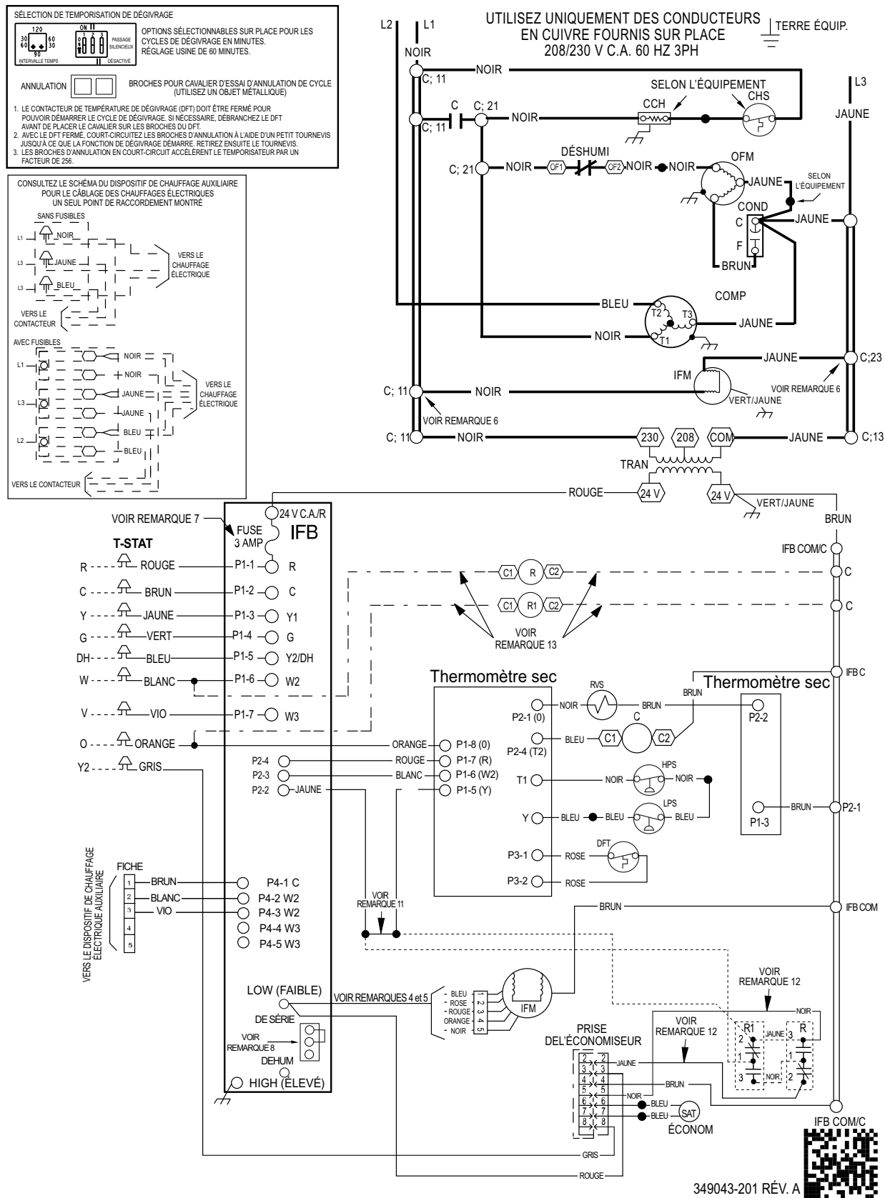
Fig. 15 – Schéma de câblage en échelle – 208/230-3-60
