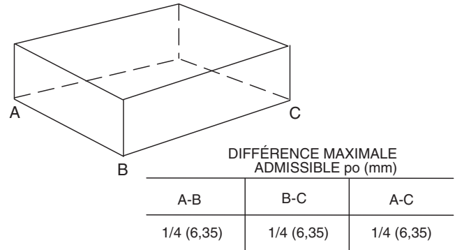
Fig. 7 – Degré de précision de niveau de l'appareil
