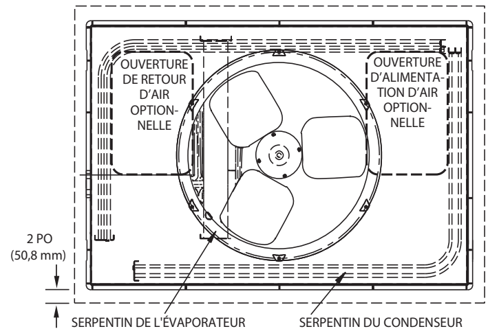
Fig. 8 – Détails du montage sur dalle
