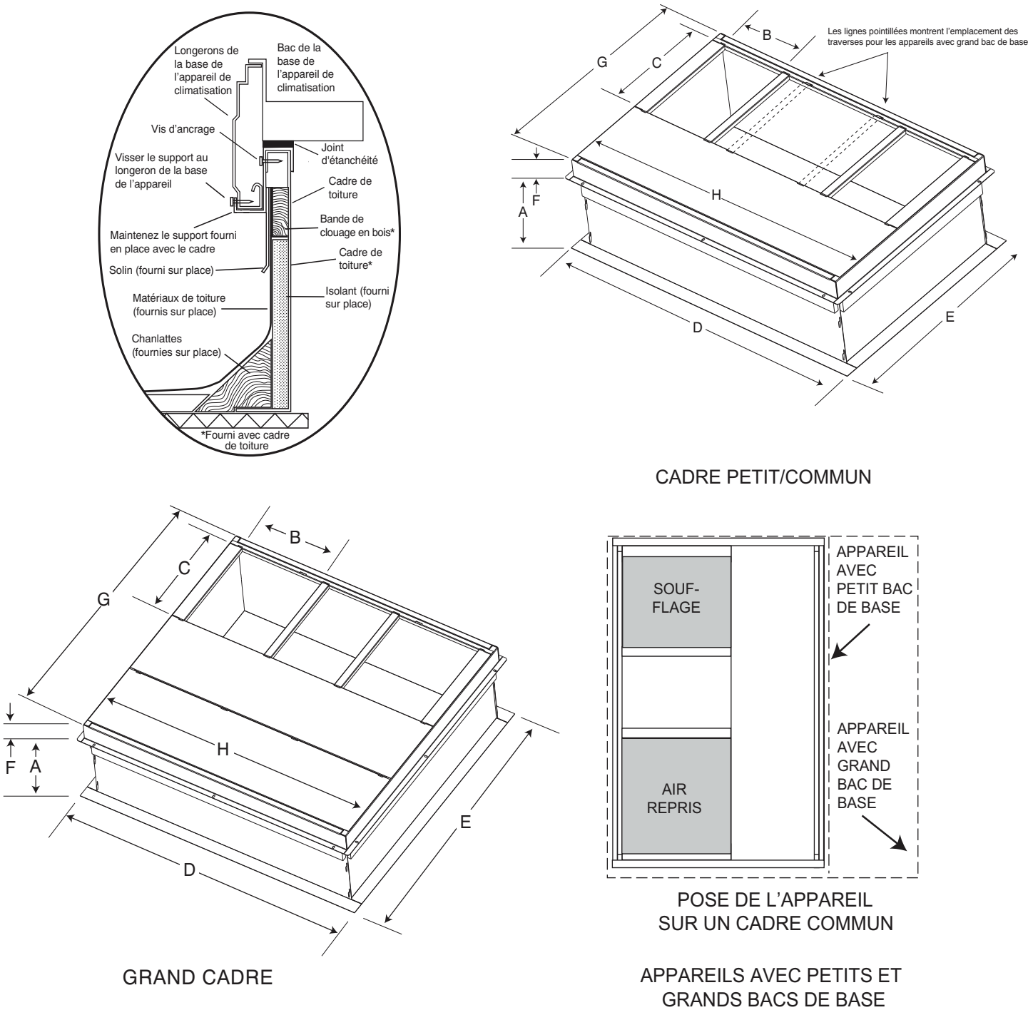
Fig. 4 – Dimensions du cadre de toiture
