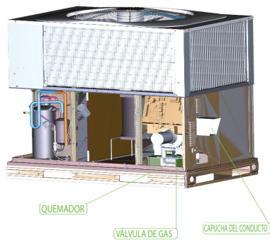
Fig. 3 – Unidad de calefacción a gas/enfriamiento eléctrico sin panel de acceso
