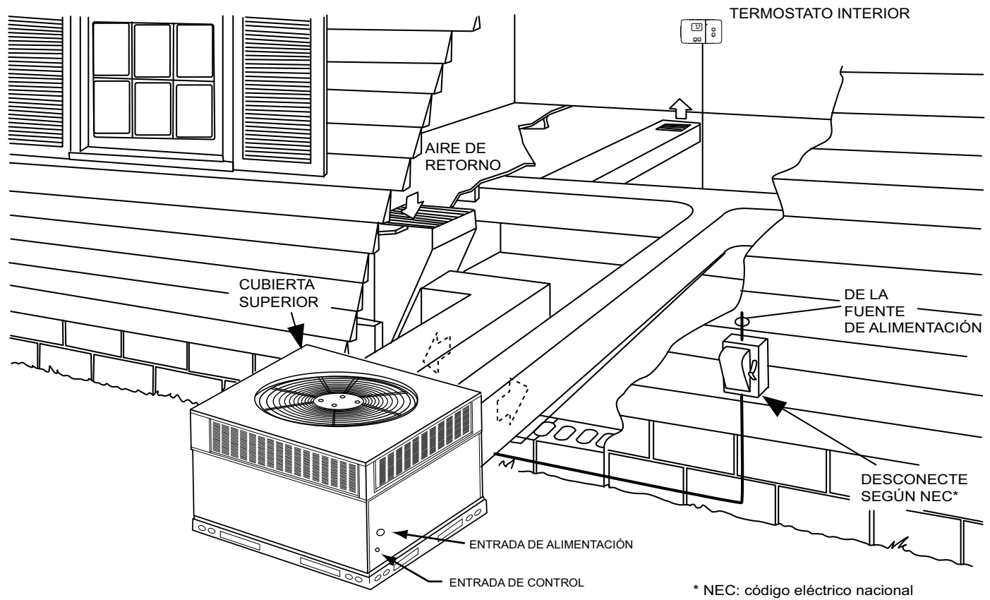
Fig. 11 – Instalación típica
