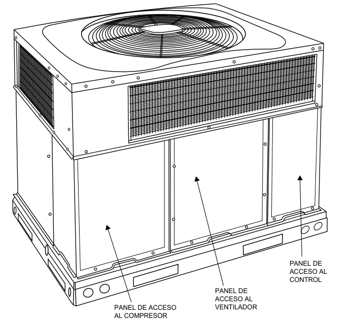
Fig. 23 – Paneles de acceso de la unidad
