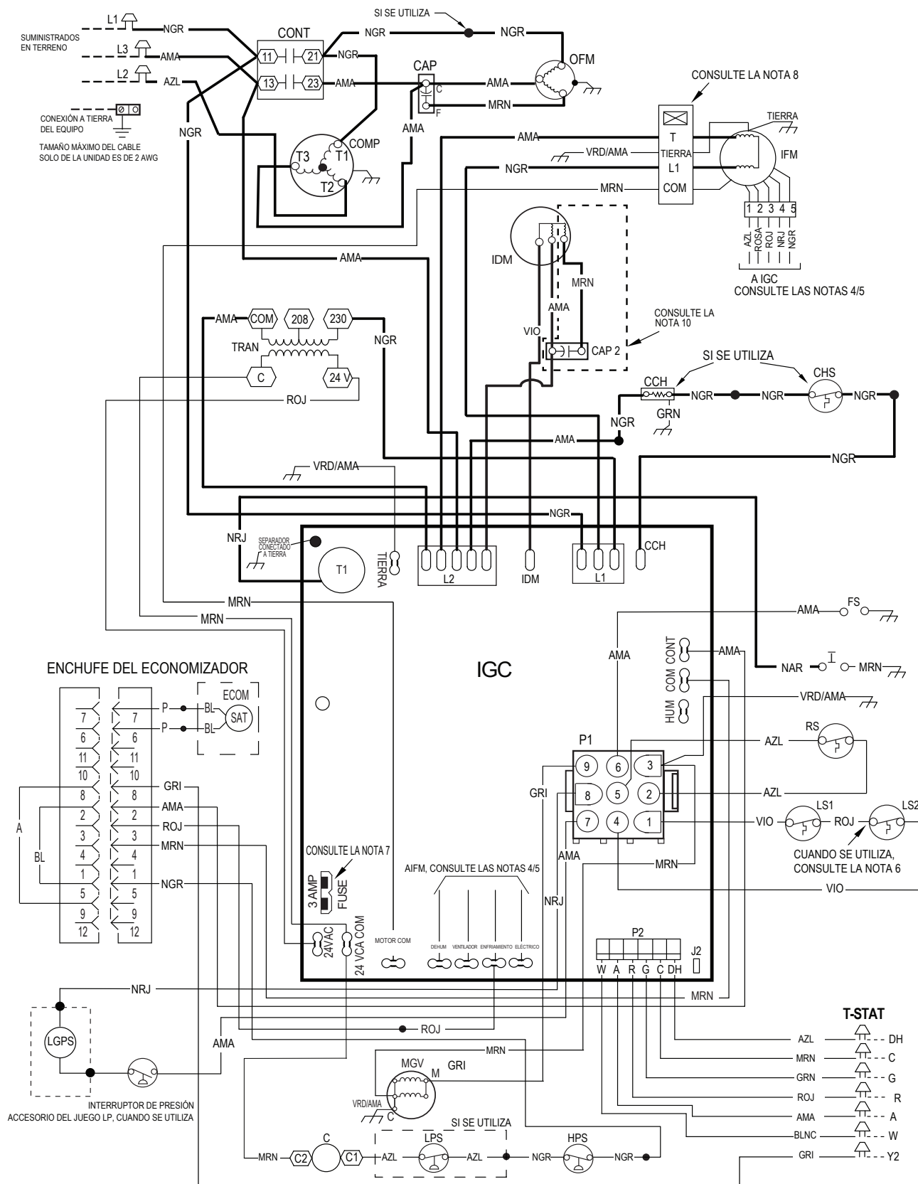
Fig. 18 – Diagrama eléctrico de conexión 460-3-60
