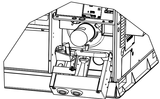
Fig. 23 – Extracción del motor y la rueda del ventilador
