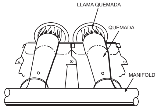
Fig. 12 – Quemador monopuerto
