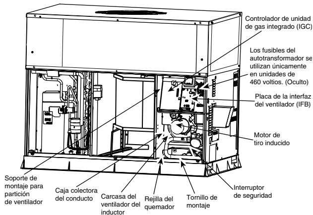
Fig. 21 – Carcasa del ventilador y caja colectora del conducto
