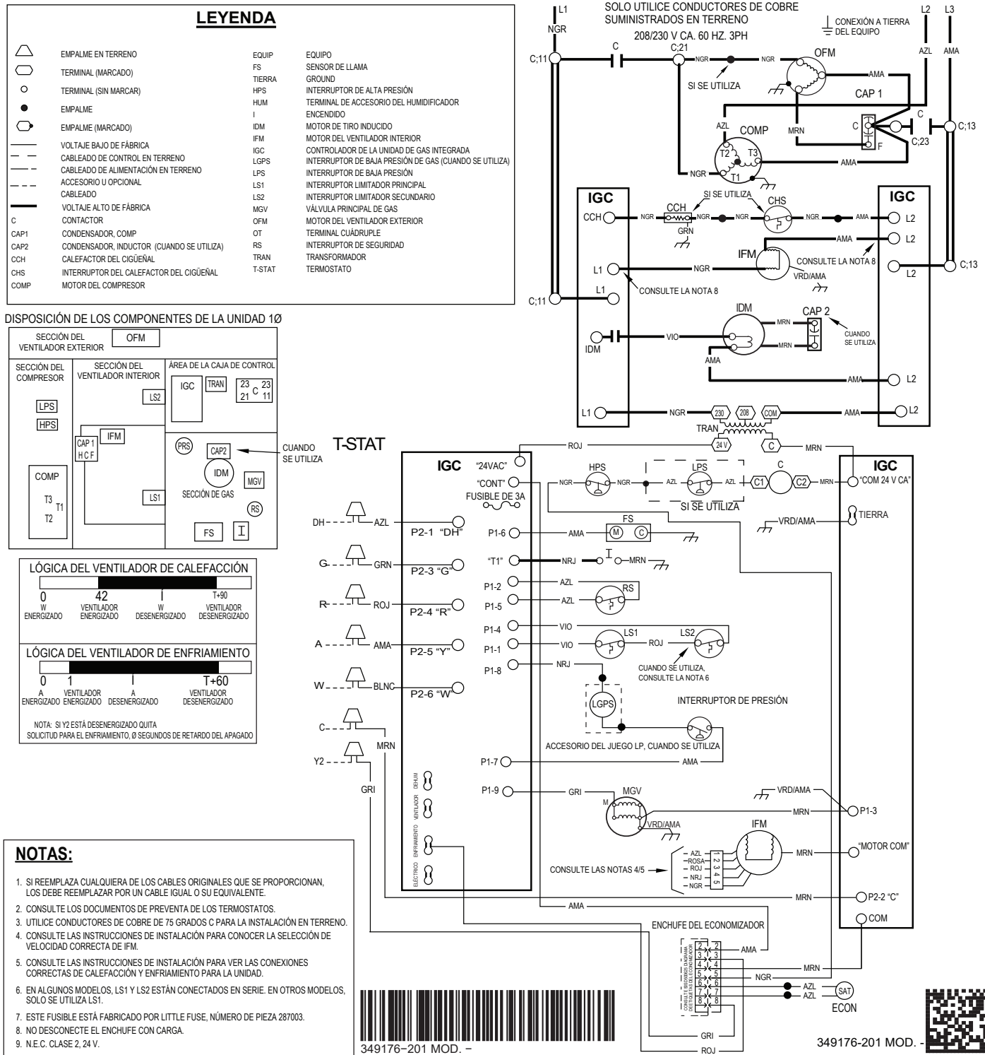
Fig. 17 – Diagrama eléctrico en escalera 208/230-3-60
