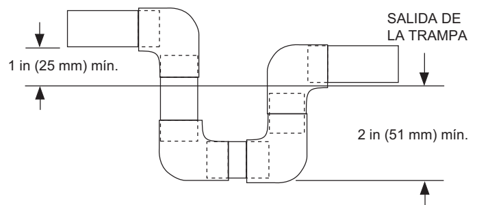
Fig. 7 – Trampa de condensado
