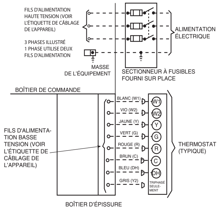
Fig. 10 – Branchements haute et basse tensions
