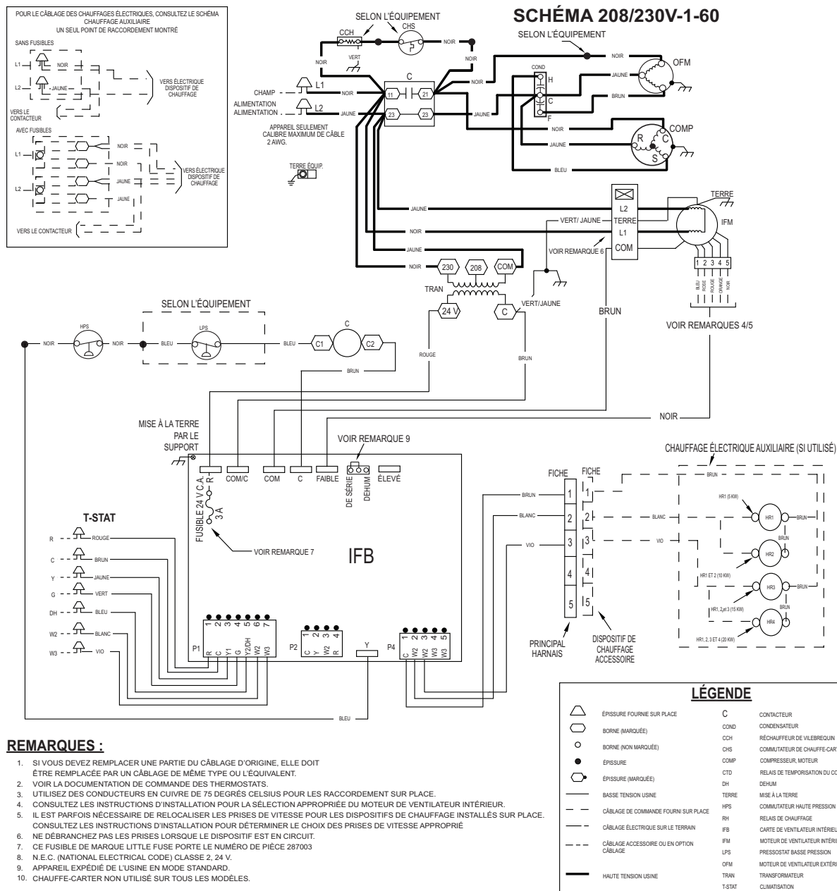
Fig. 12 – Schéma de connexion de câblage – 208/230V, 1 phase, 60Hz
