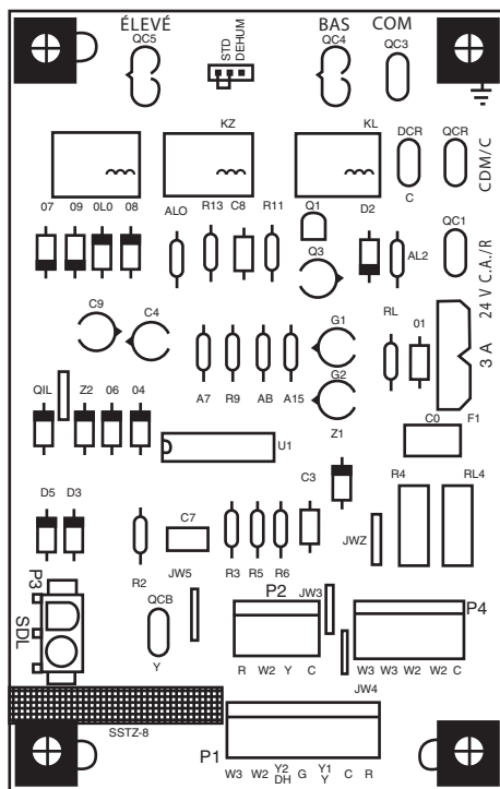
Fig. 11 – Carte interface du ventilateur (IFB)
