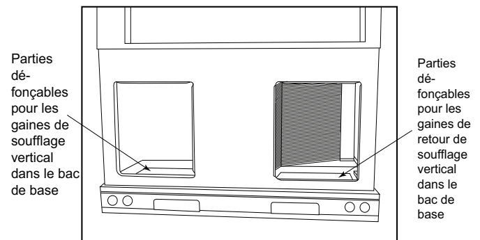
Fig. 9 – Ouvertures d'air de soufflage et de retour
