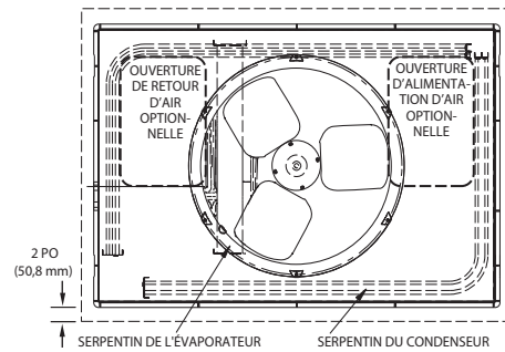
Fig. 7 – Détails du montage sur dalle
