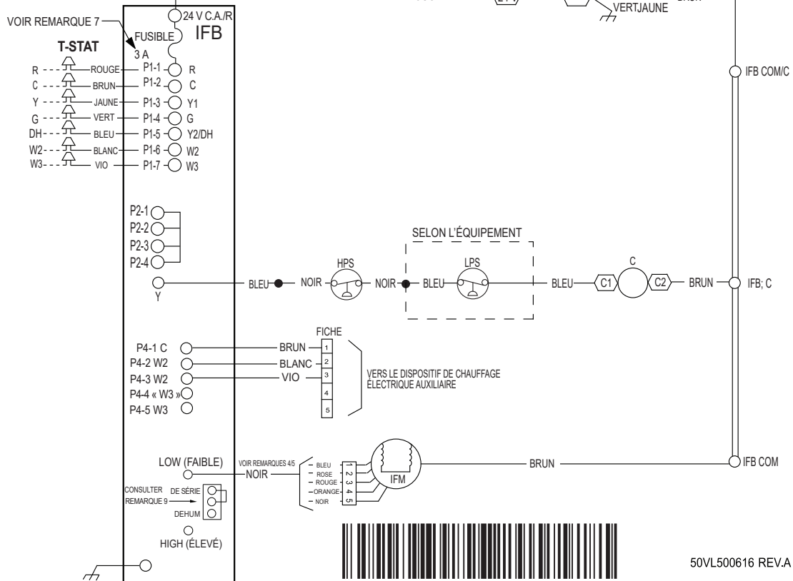
Fig. 13 – Schéma de câblage en échelle – 208/230-1-60
