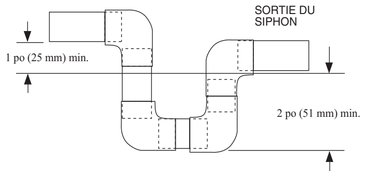
Fig. 8 – Siphon de condensat
