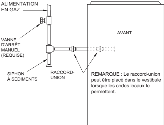
Fig. 31 – Disposition type de la tuyauterie de gaz
