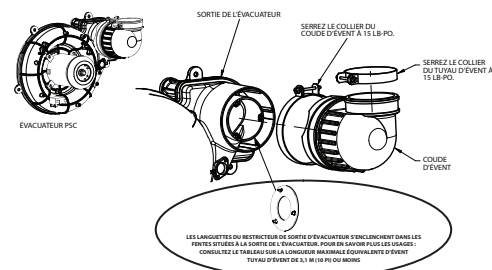
Fig. 52 – Coude d'évent d'évacuateur
