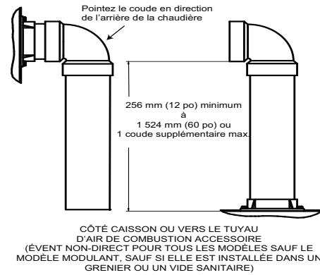
Fig. 44 – Fixation du tuyau d'air de combustion
