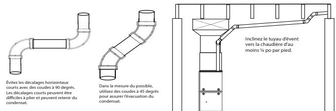
Fig. 51 – Raccordement des événements près de la chaudière
