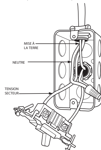
Fig. 35 – Coffret électrique externe fourni sur place sur le caisson de la chaudière
