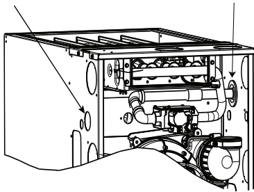
Fig. 29 – Entrée de gaz
