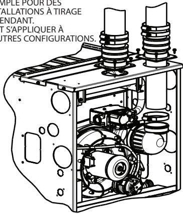
Fig. 43 – Exemple de raccordement de tuyau d'entrée d'air pour des systèmes de ventilation en polypropylène
