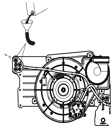
Fig. 59 – Amorçage du siphon de condensat
