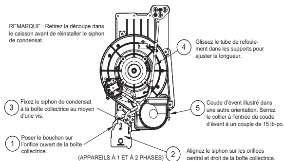
Fig. 10 – Configuration de siphon horizontal à droite A11573FR (l'apparence peut varier)
