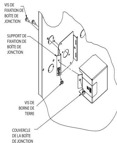
Fig. 34 – Installation d'une boîte de jonction (le cas échéant)
