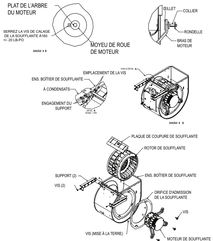
Fig. 64 – Ventilateur en marche 30040A et 36060A
