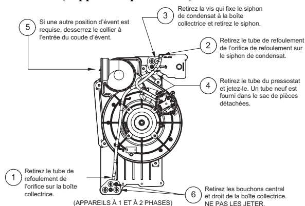
Fig. 10 – Configuration de siphon horizontal à droite A11573FR (l'apparence peut varier)
