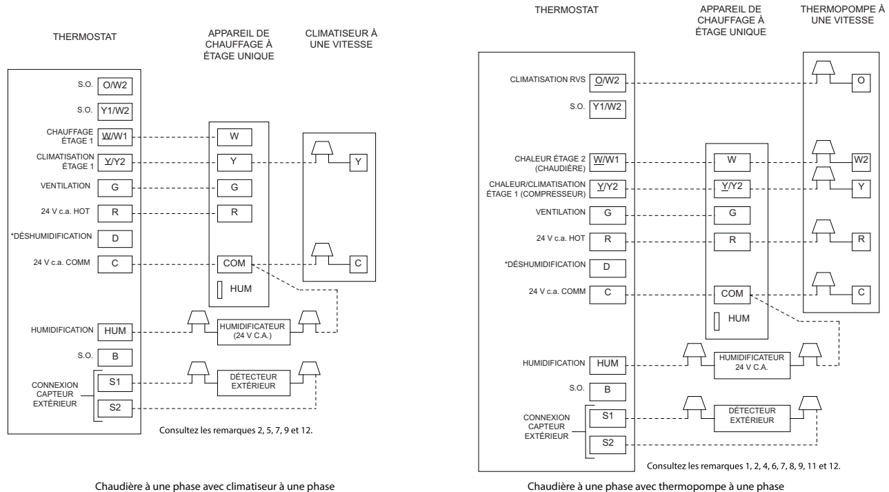
Fig. 37 – Exemple de panneau de commande de chaudière monophasée
