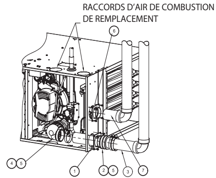
CONFIGURATION HORIZONTALE À DROITE ET VENTILATION À DROITE
