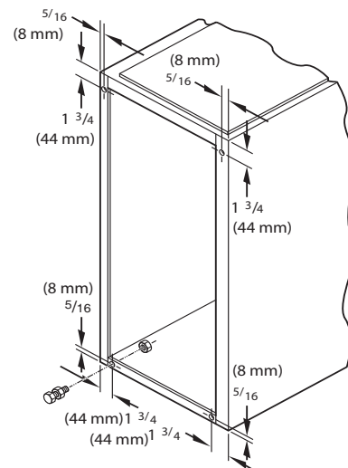
Fig. 28 – Pattes de mise à niveau
