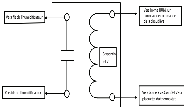
Fig. 36 – Relais d'isolation pour humidificateurs, fourni sur place, avec bloc d'alimentation interne
