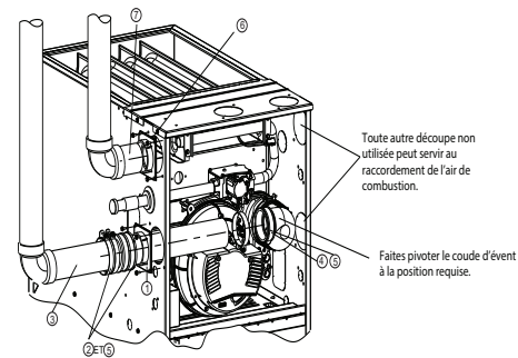
Fig. 52 – Coude d'évent d'évacuateur
