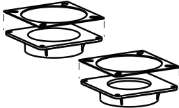
Fixez les joints aux adaptateurs de tuyaux d'évent et d'air de combustion.
