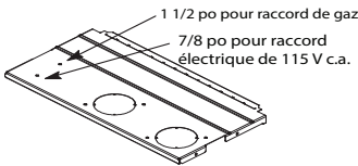
Fig. 30 – Entrée de gaz et d'électricité facultative
