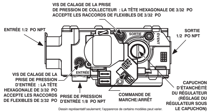
Fig. 62 – Soupapes de gaz
