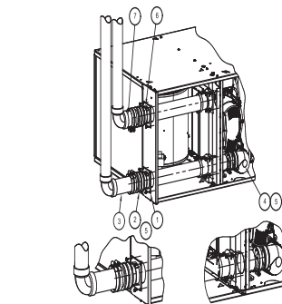
CONFIGURATION HORIZONTALE À DROITE ET VENTILATION VERTICALE
