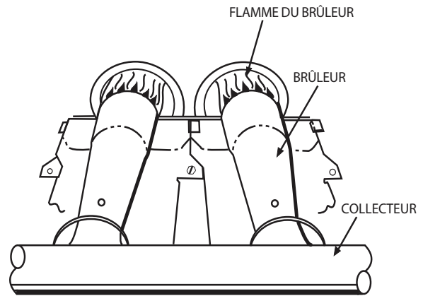
Fig. 8 – Brûleur monoport
