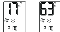
Economizer low limit temperature (°C) (°F)
