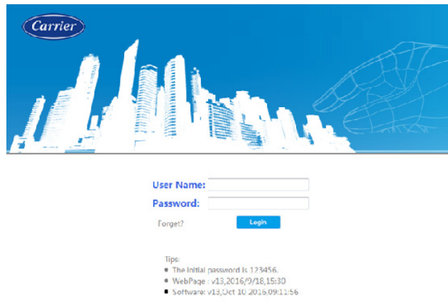
Fig. 7 —Login Screen
