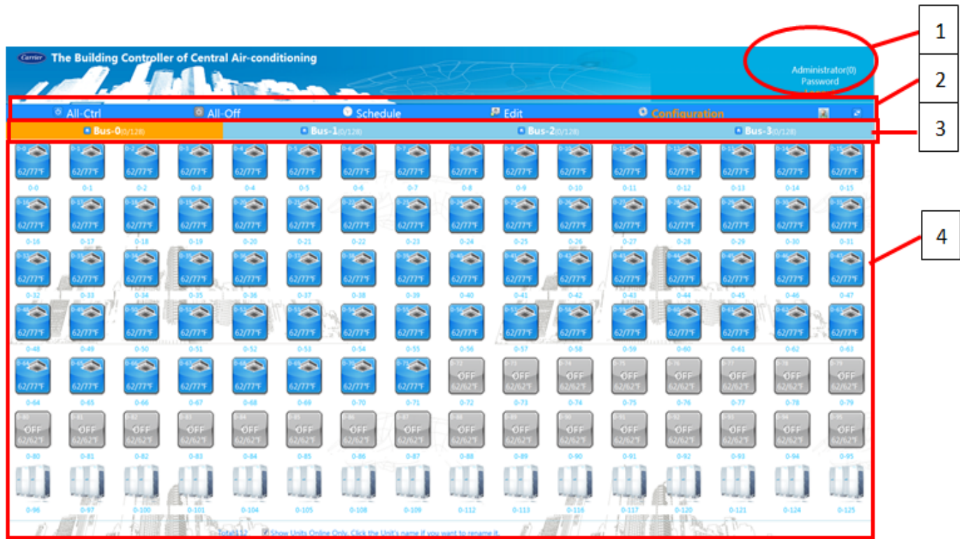
Fig. 9 —Homepage
