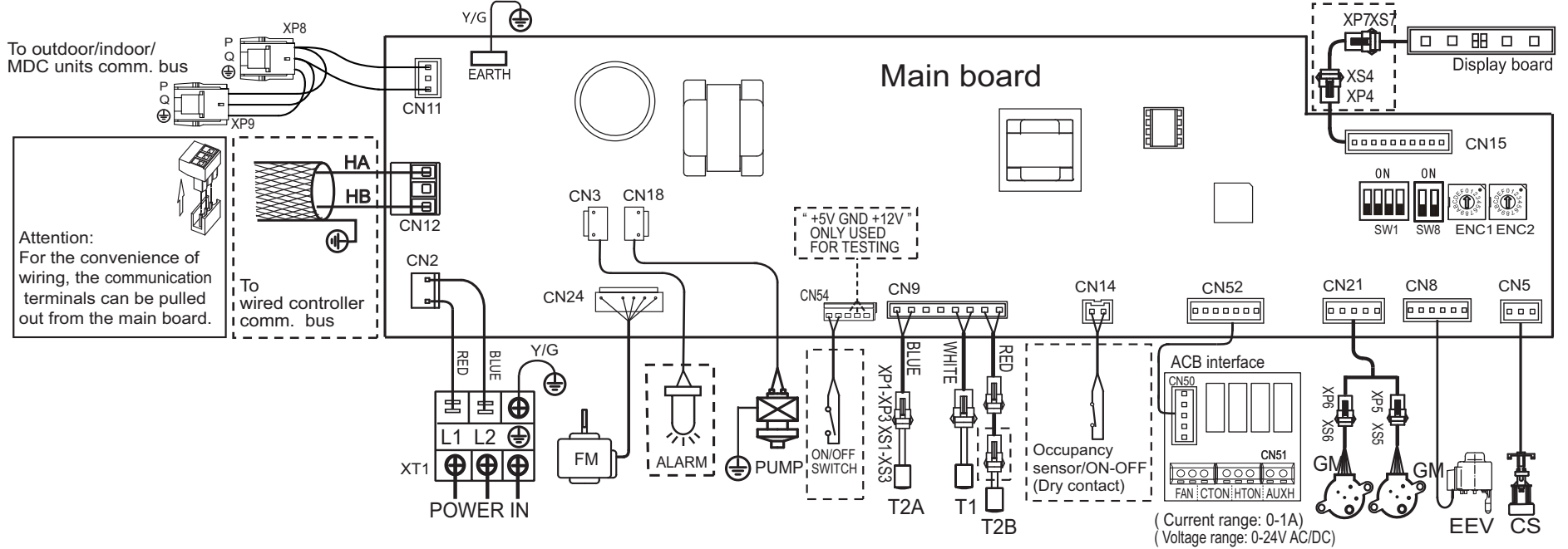
Fig. 3 —40VMF009A--3 to 40VMF048A--3
