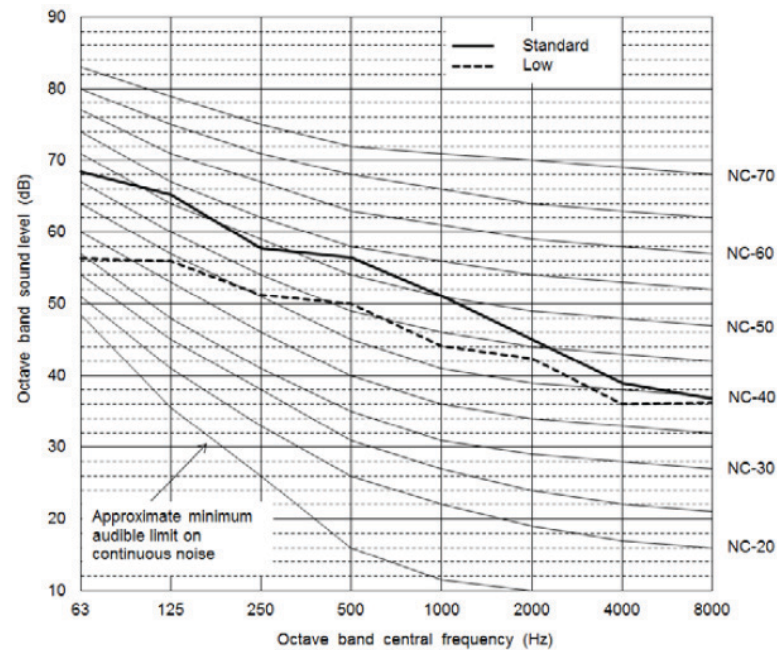
Fig. 21 —38VMA072RDS6-1
