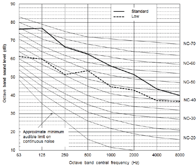
Fig. 33 —38VMA216RDS6-1
