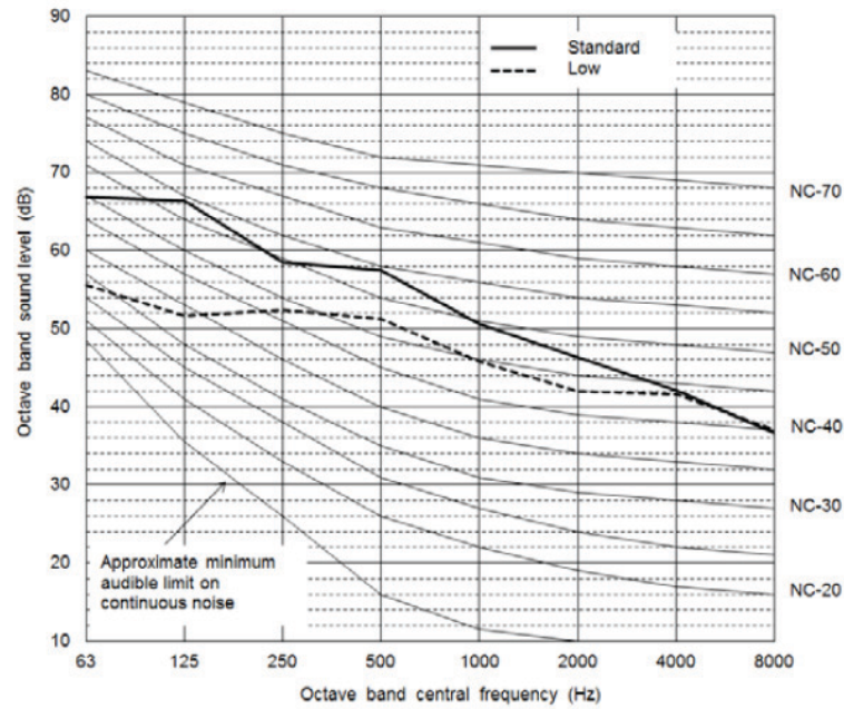
Fig. 20 —38VMA072RDS5-1
