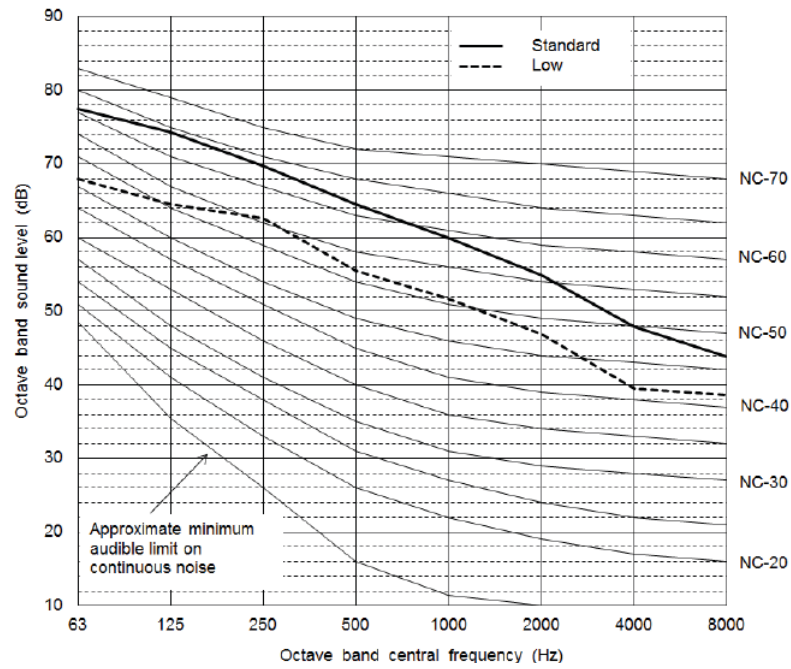
Fig. 44 —38VMA336RDS5-1
