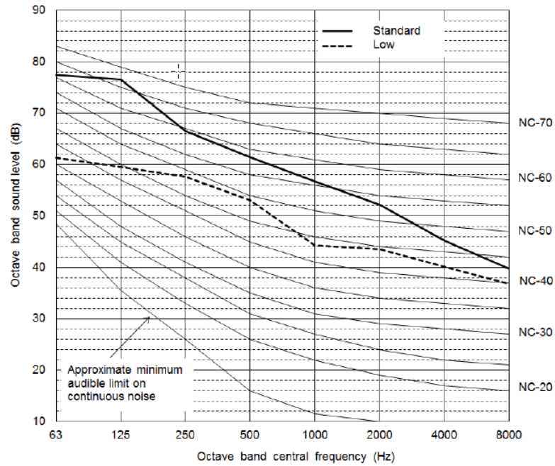
Fig. 32 —38VMA216RDS5-1
