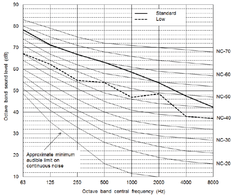
Fig. 38 —38VMA264RDS5-1
