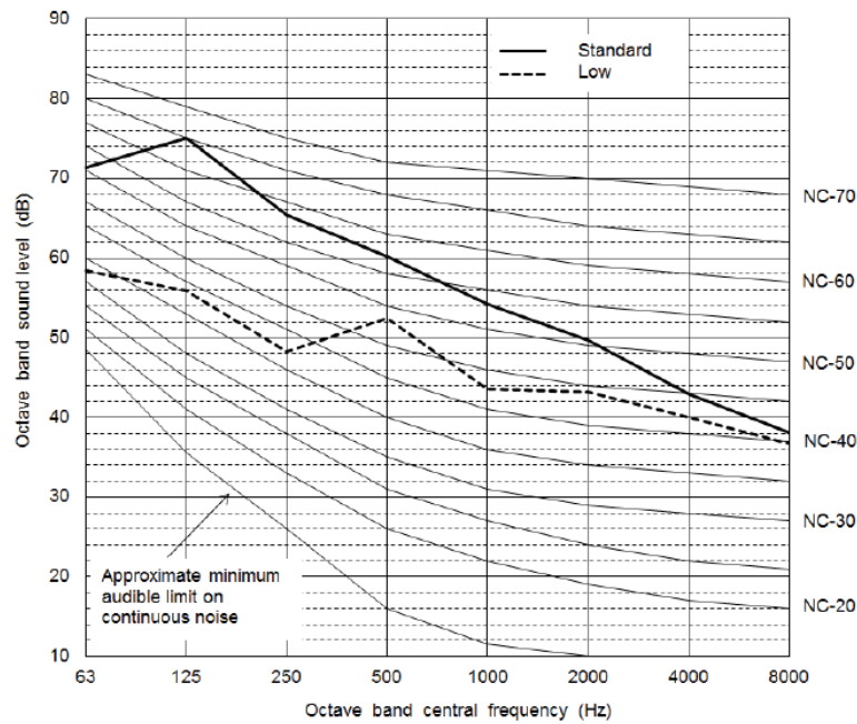
Fig. 30 —38VMA192RDS5-1
