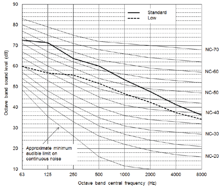
Fig. 24 —38VMA120RDS5-1
