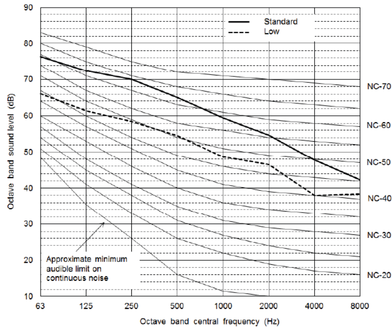
Fig. 42 —38VMA312RDS5-1
