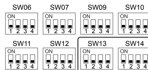
Commandez les réglages pour l'adresse de la ligne (système) sur la carte d'interface de unité extérieure principale
