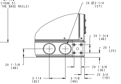
DETAIL A TYP. 4-PLCS
