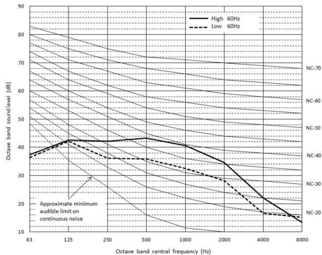
Fig. 20 —40VMC015A--3
