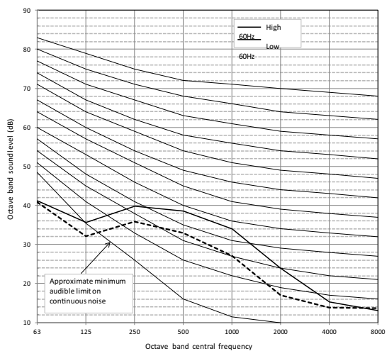
Fig. 16 —40VMC005A--3
