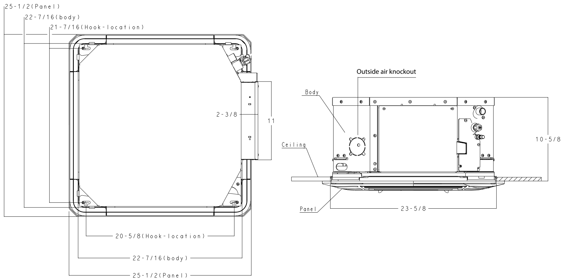
Fig. 3 —40VMC005A/007A/009A/012A/015A--3
