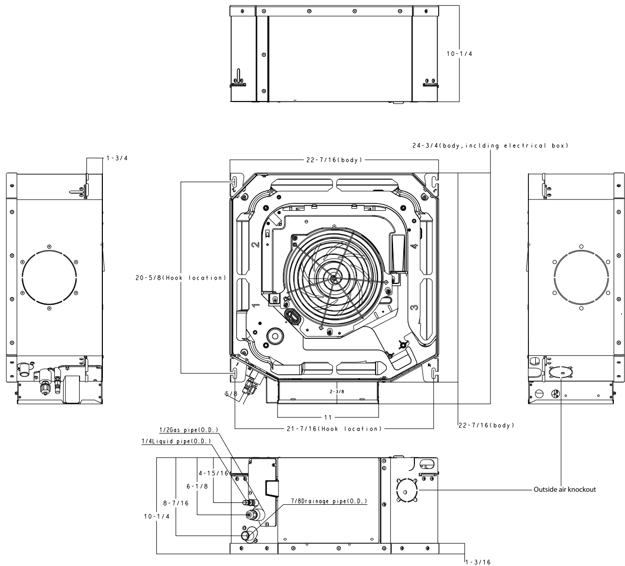
Fig. 2 —40VMC005A/007A/009A/012A/015A--3
