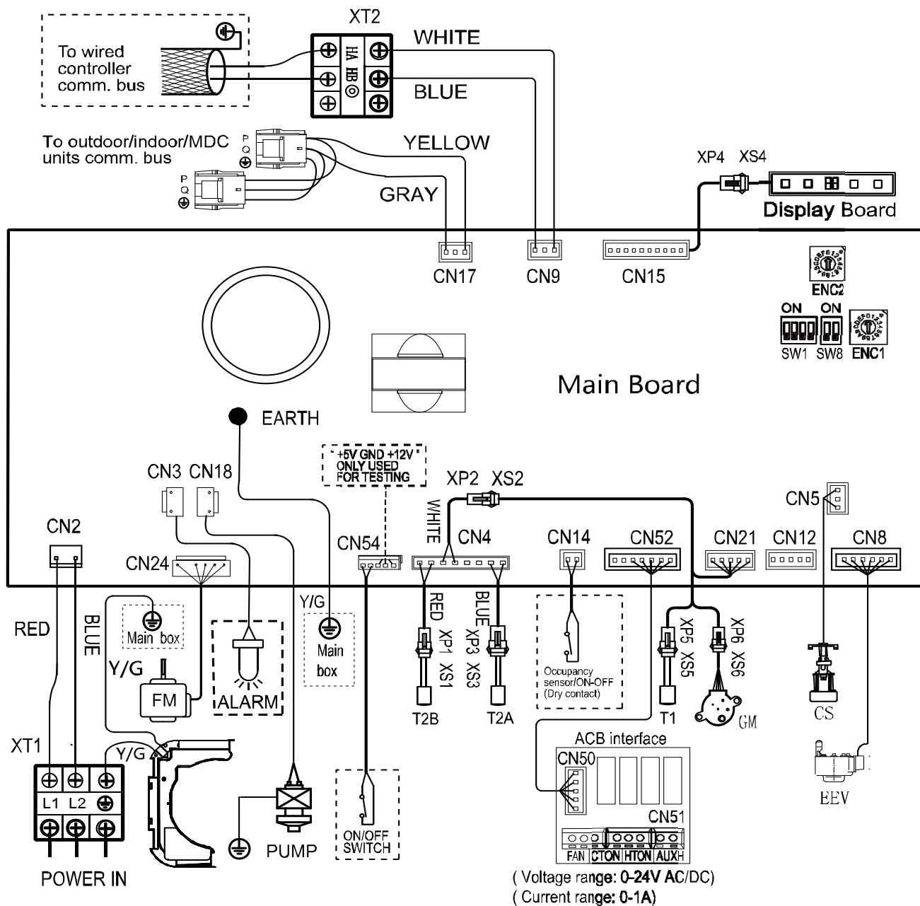
Fig. 4 —40VMC005A/007A/009A/012A/015A--3
