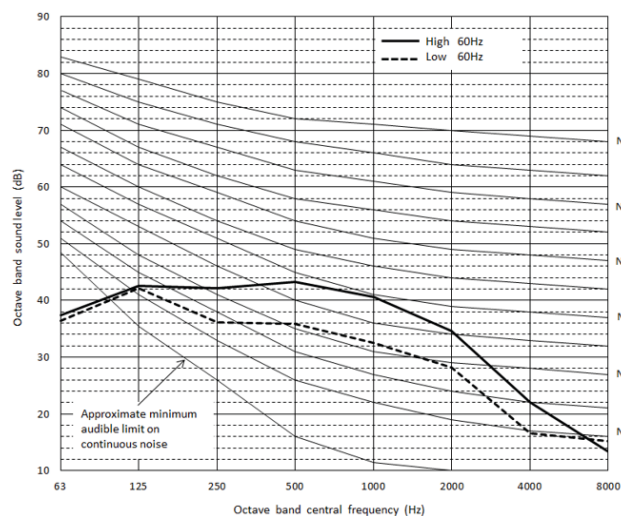
Fig. 19 —40VMC012A--3
