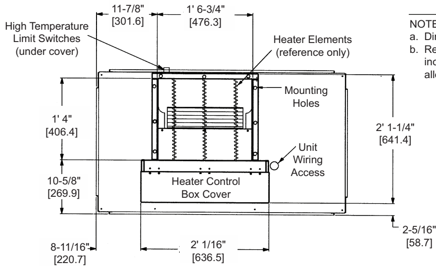
Top
