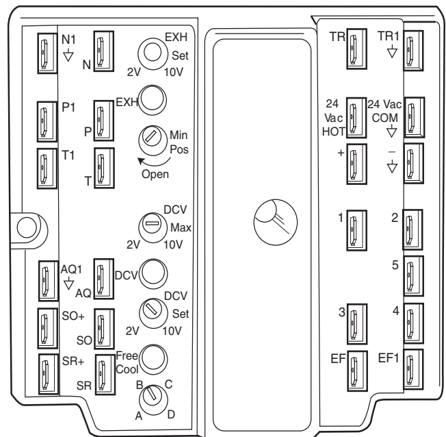
Fig. 63 — EconoMi$er IV W7212 Control
