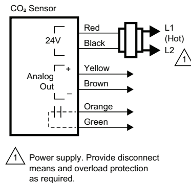
Fig. 70 — CO 2 Sensor Wiring
